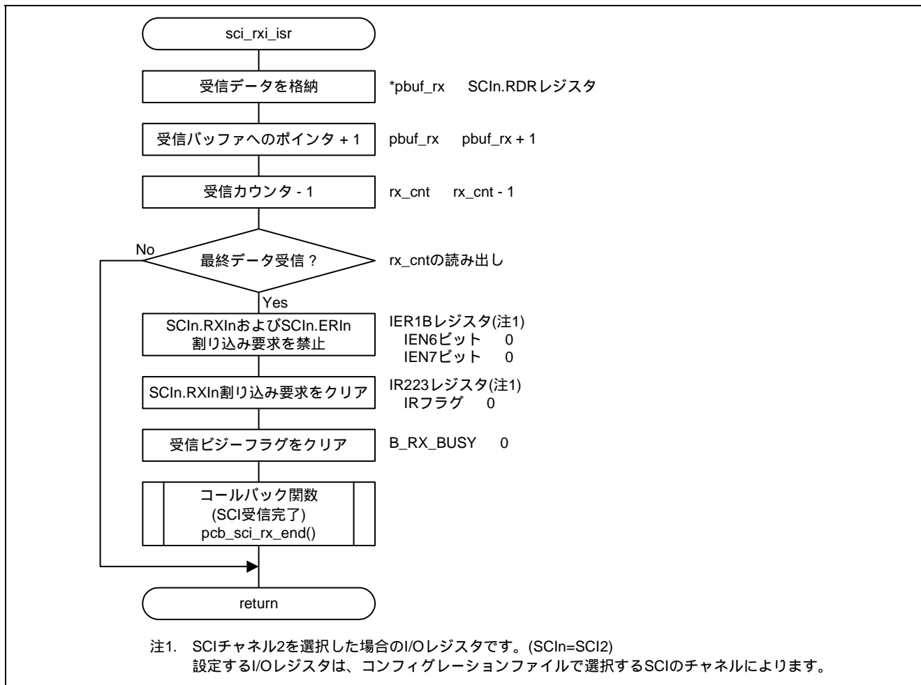
図 4.18 受信データフル割り込み
