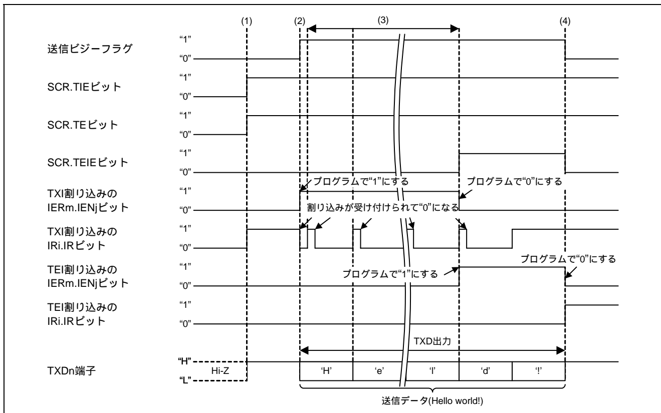
図 4.2 シリアル送信のタイミング図
