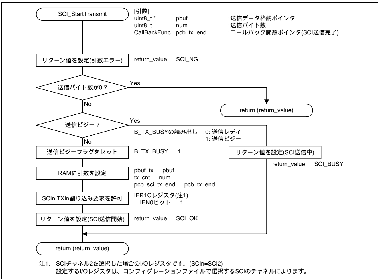
図 4.14 ユーザ I/F 関数 (SCI 送信開始)
