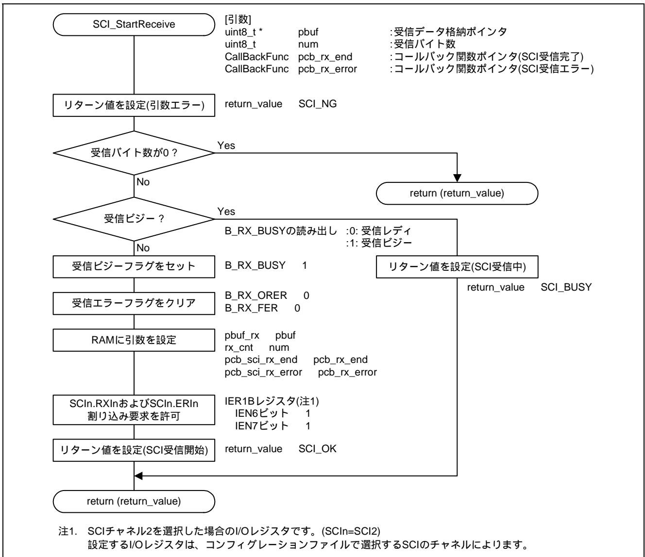
図 4.13 ユーザ I/F 関数 (SCI 受信開始)
