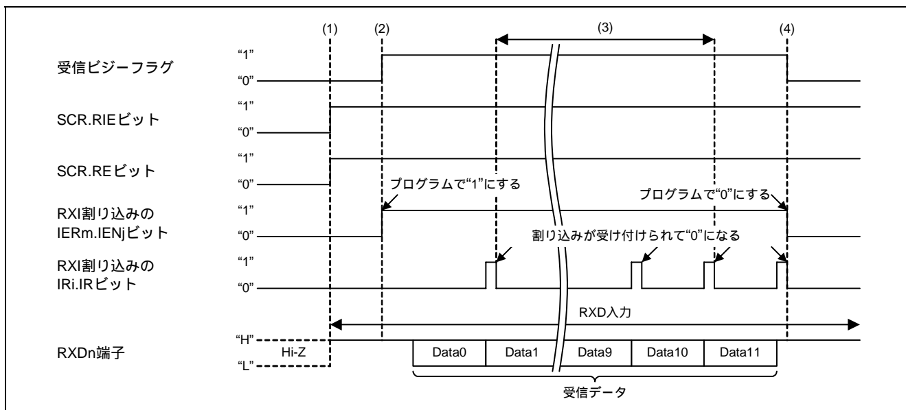
図 4.3 シリアル受信のタイミング図
