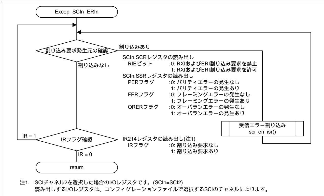
図 4.21 SCI.ERI 割り込み処理
