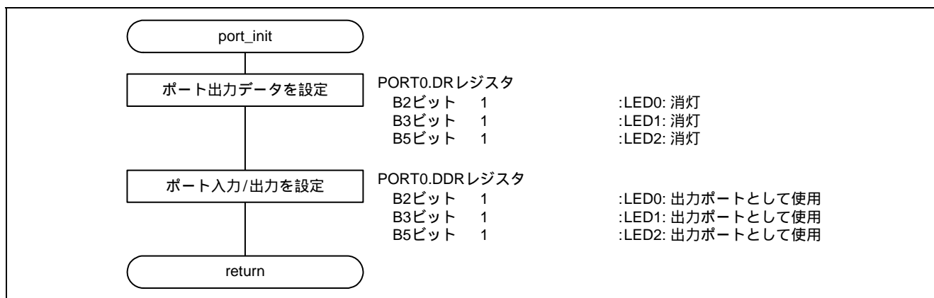
図 4.6 ポート初期設定
