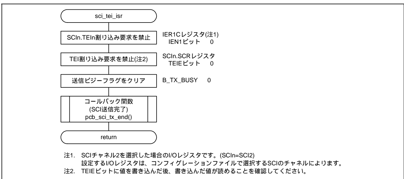
図 4.17 送信終了割り込み
