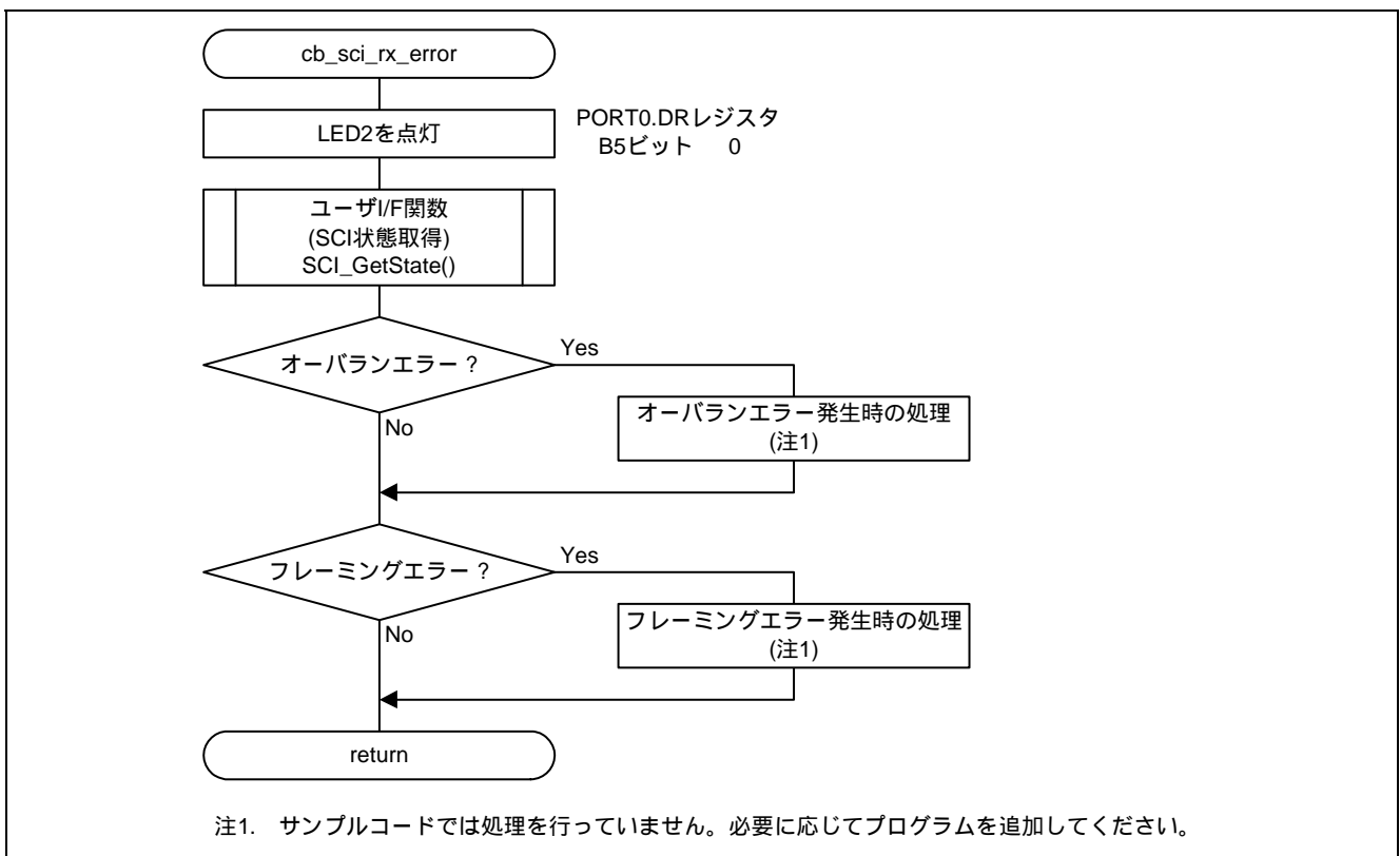
図 4.10 コールバック関数 (SCI 受信エラー)
