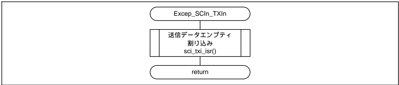
図 4.23 SCI.TXI 割り込み処理
