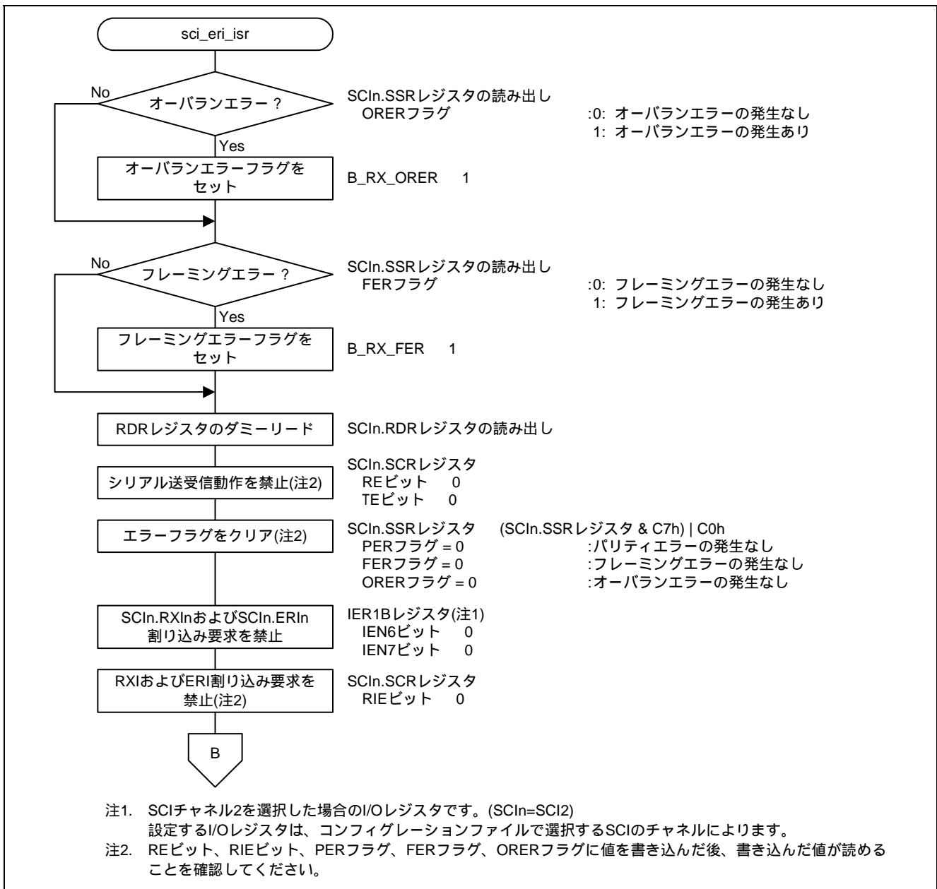
図 4.19 受信エラー割り込み (1/2)
