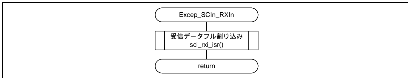
図 4.22 SCI.RXI 割り込み処理
