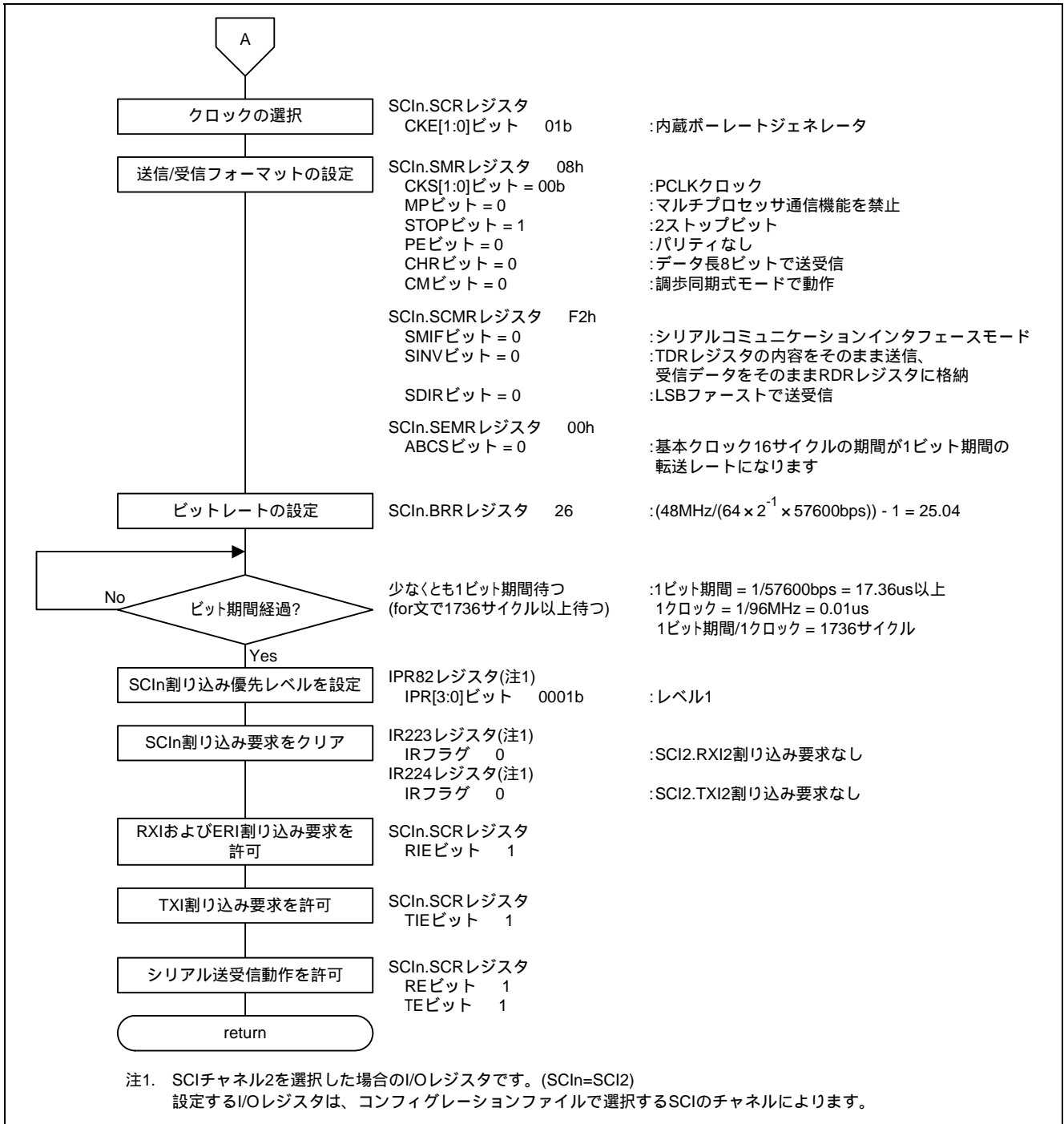
図 4.12 ユーザ I/F 関数 (SCI 初期設定) (2/2)
