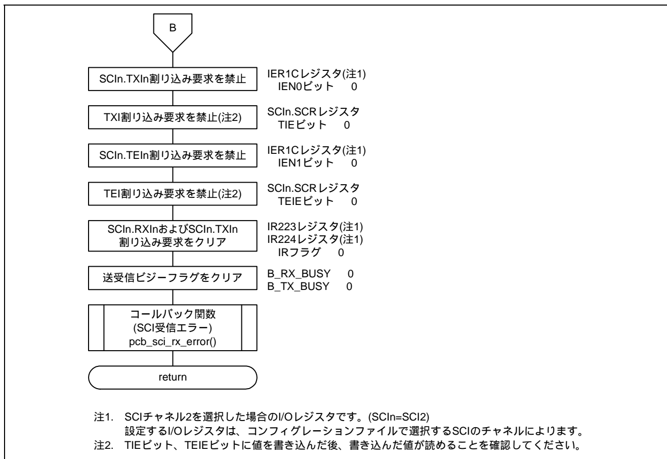
図 4.20 受信エラー割り込み ( 2/2 )
