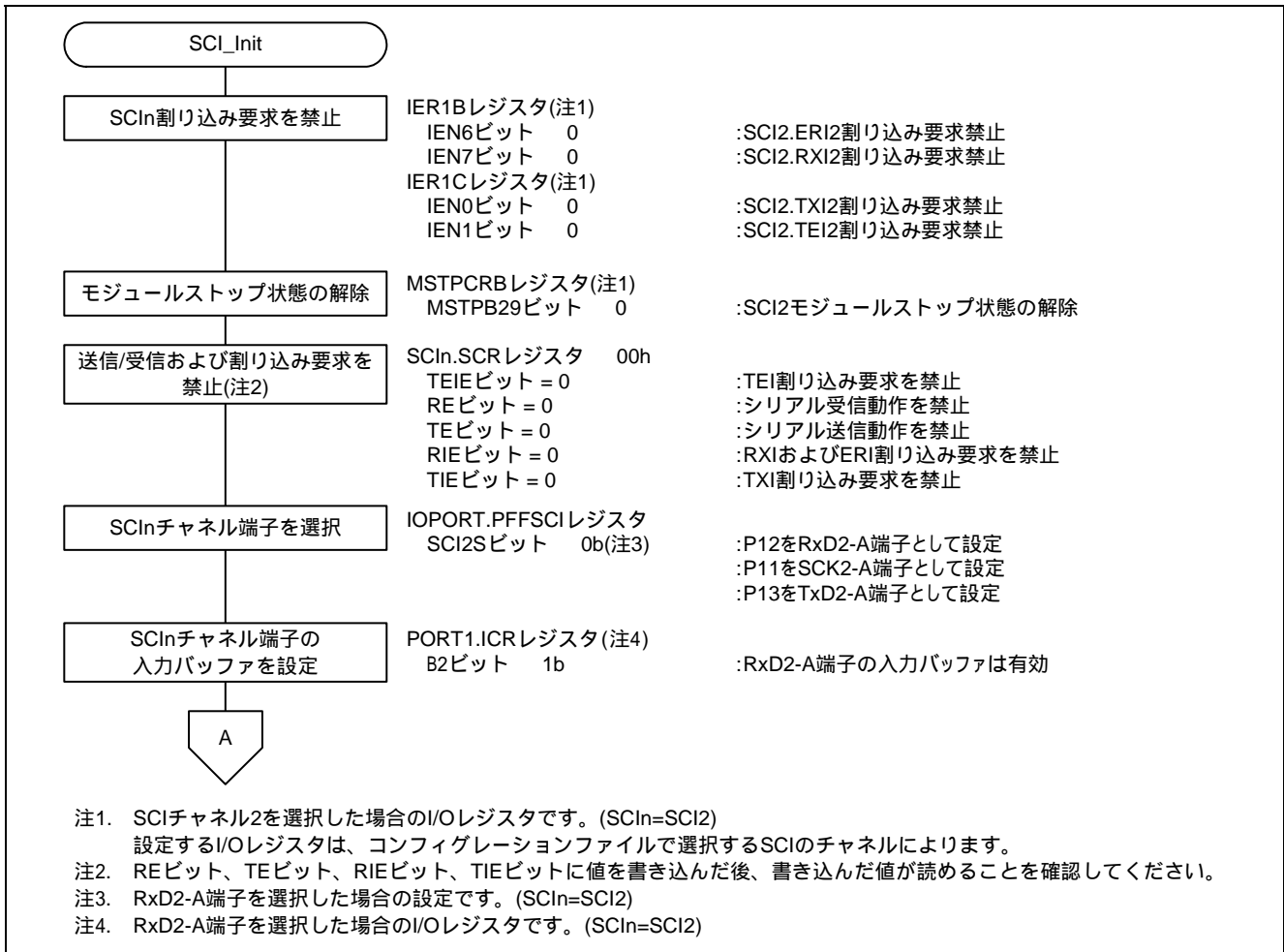
図 4.11 ユーザ I/F 関数 (SCI 初期設定) (1/2)
