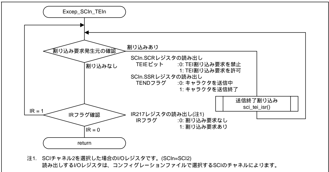
図 4.24 SCI.TEI 割り込み処理
