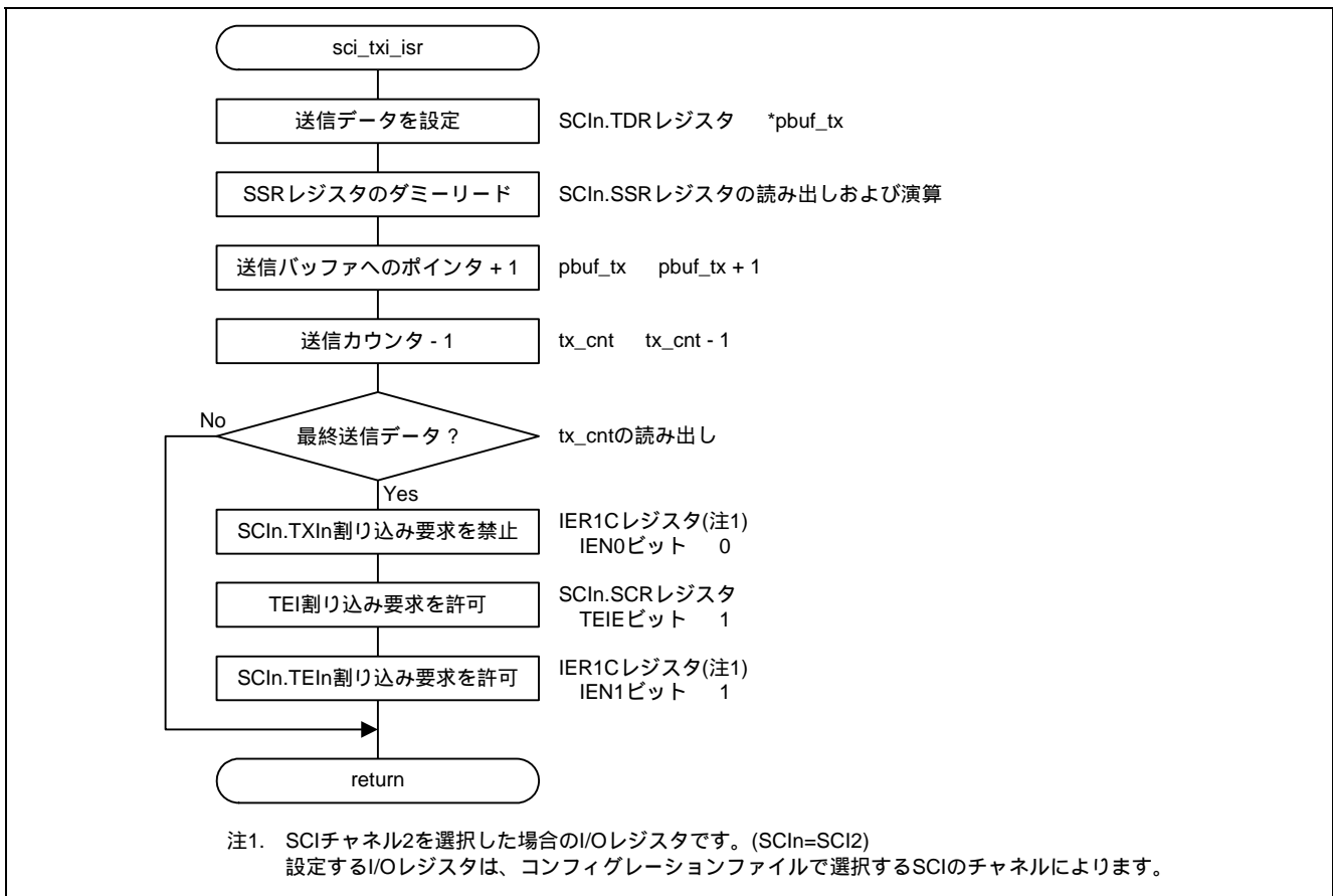
図 4.16 送信データエンプティ割り込み
