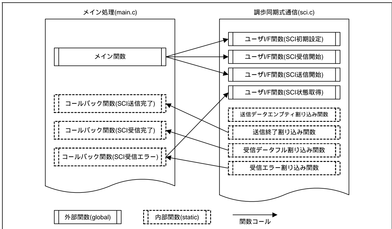
図 4.1 ソフトウェア構成
