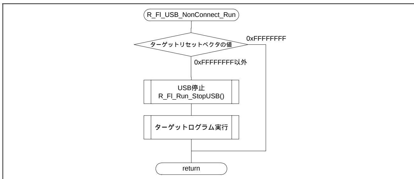
図5.37 USB 未接続時のターゲットプログラム実行
