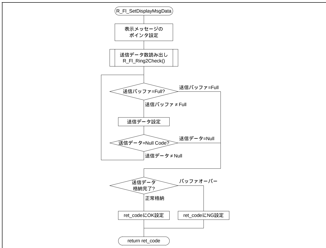
図5.34 メッセージ表示
