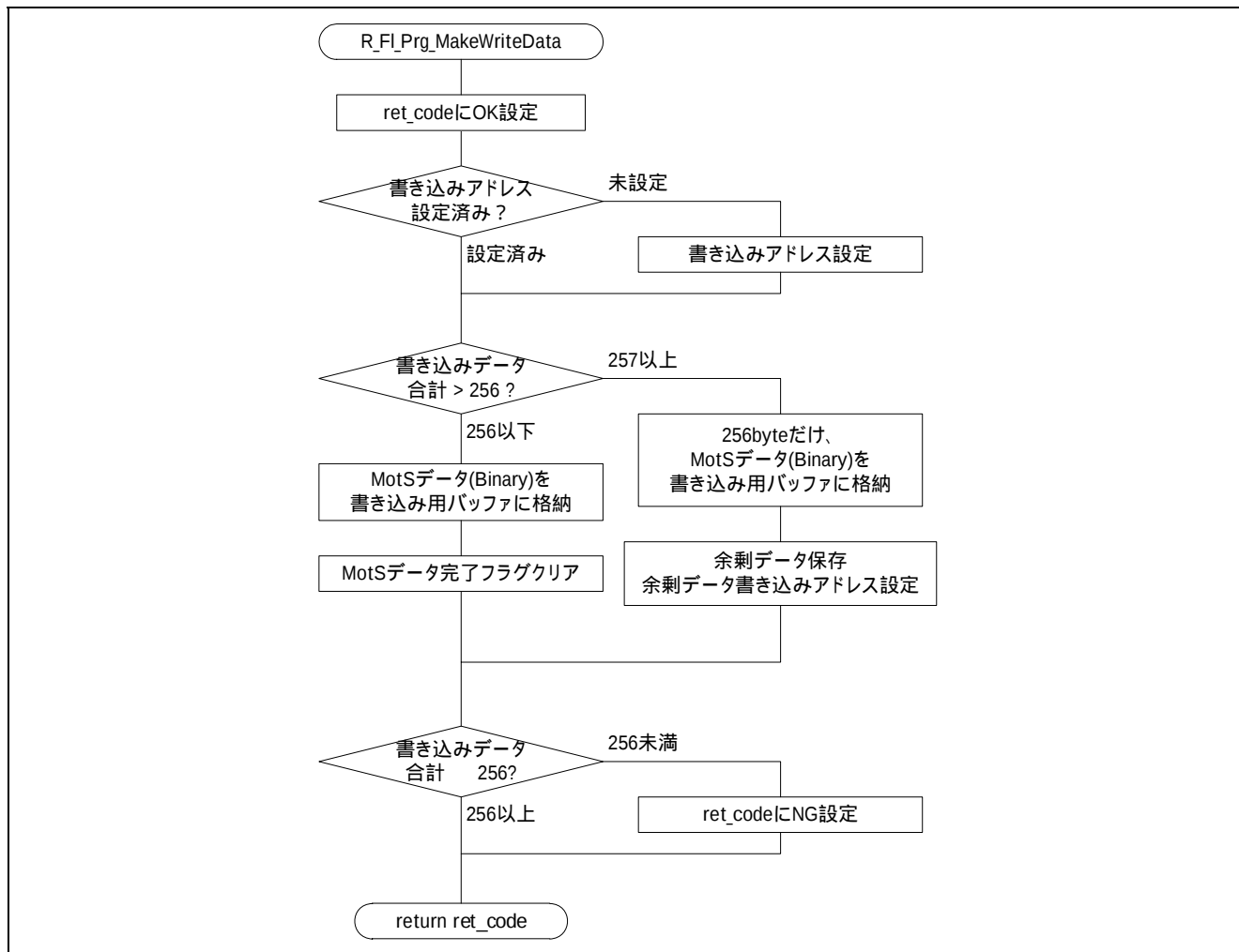
図5.28 ターゲットエリアへの書き込みデータ作成
