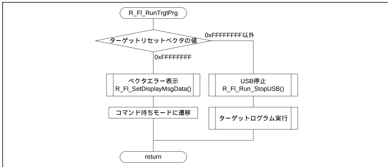
図5.15 実行モード処理
