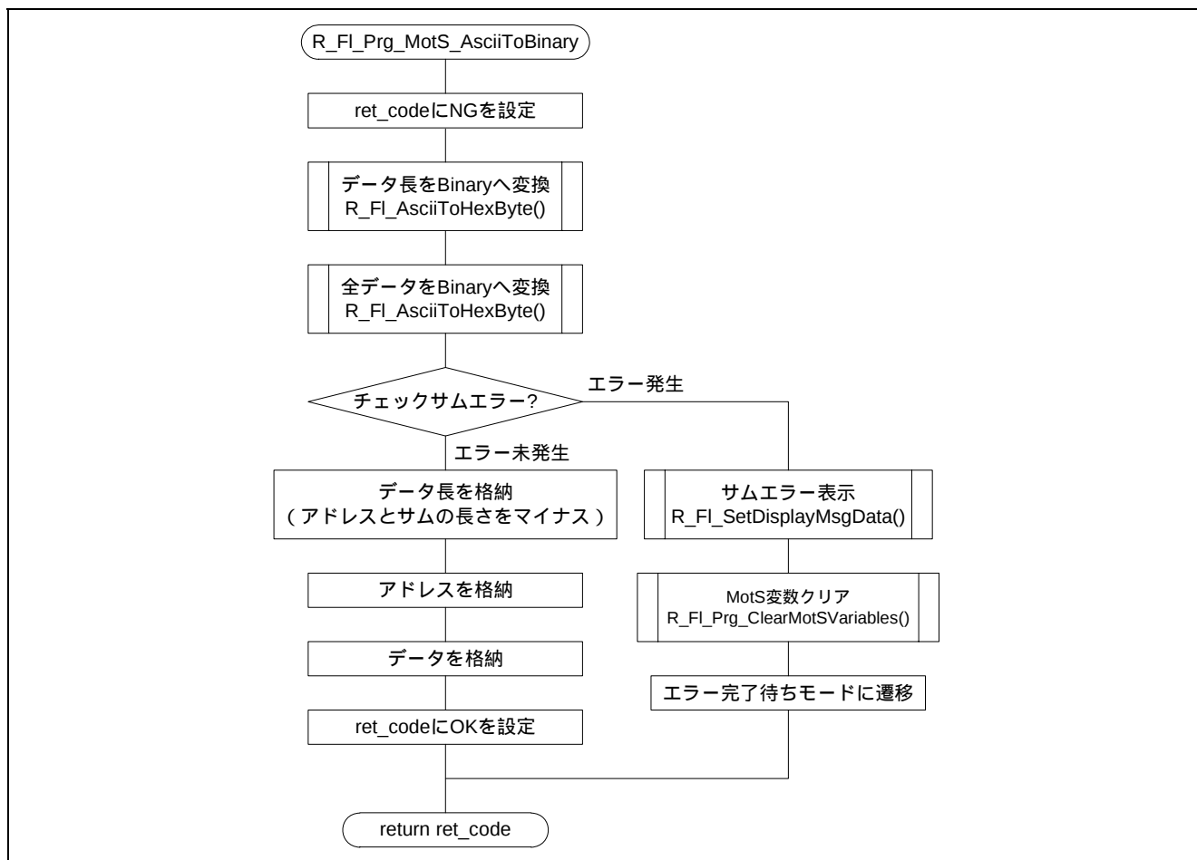
図5.27 Motorola S フォーマットデータ ASCII - Binary 変換
