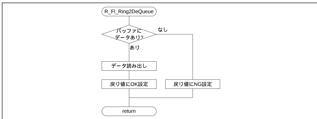
図5.43 送信用リングバッファからのデータ読み出し
