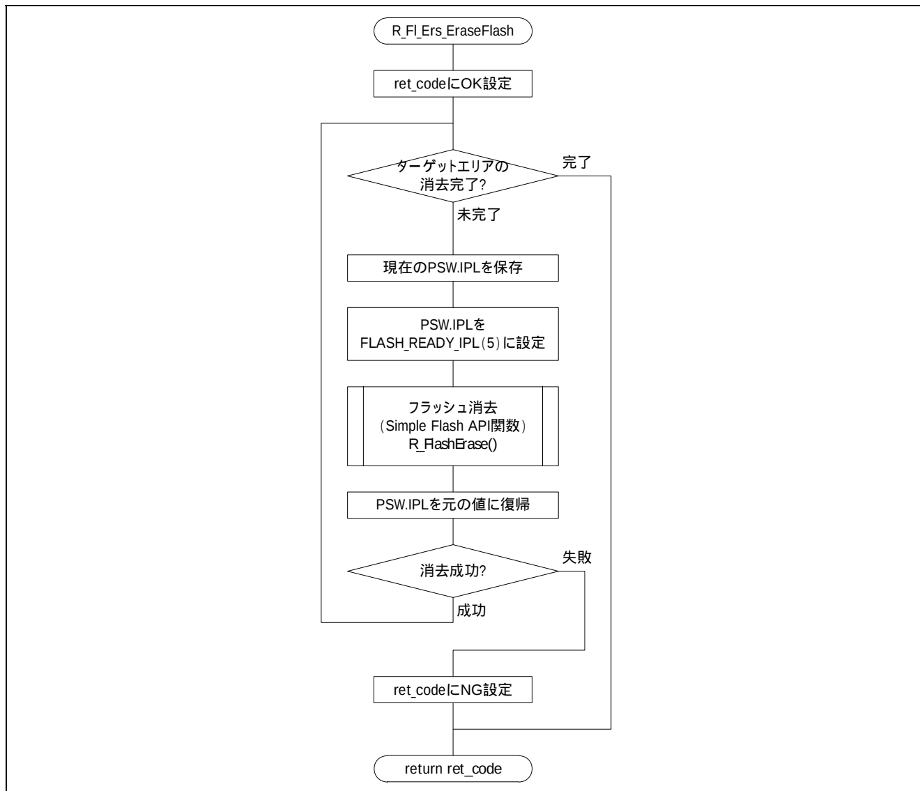
図5.23 ターゲットエリア消去
