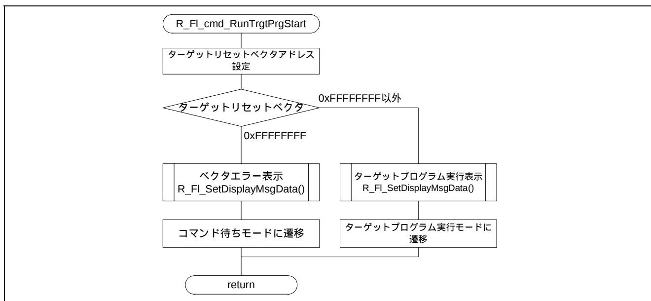
図5.21 ターゲットプログラム実行開始
