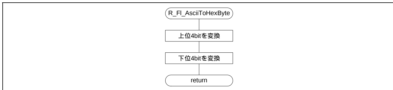
図5.46 ASCII コードから Binary データへの変換
