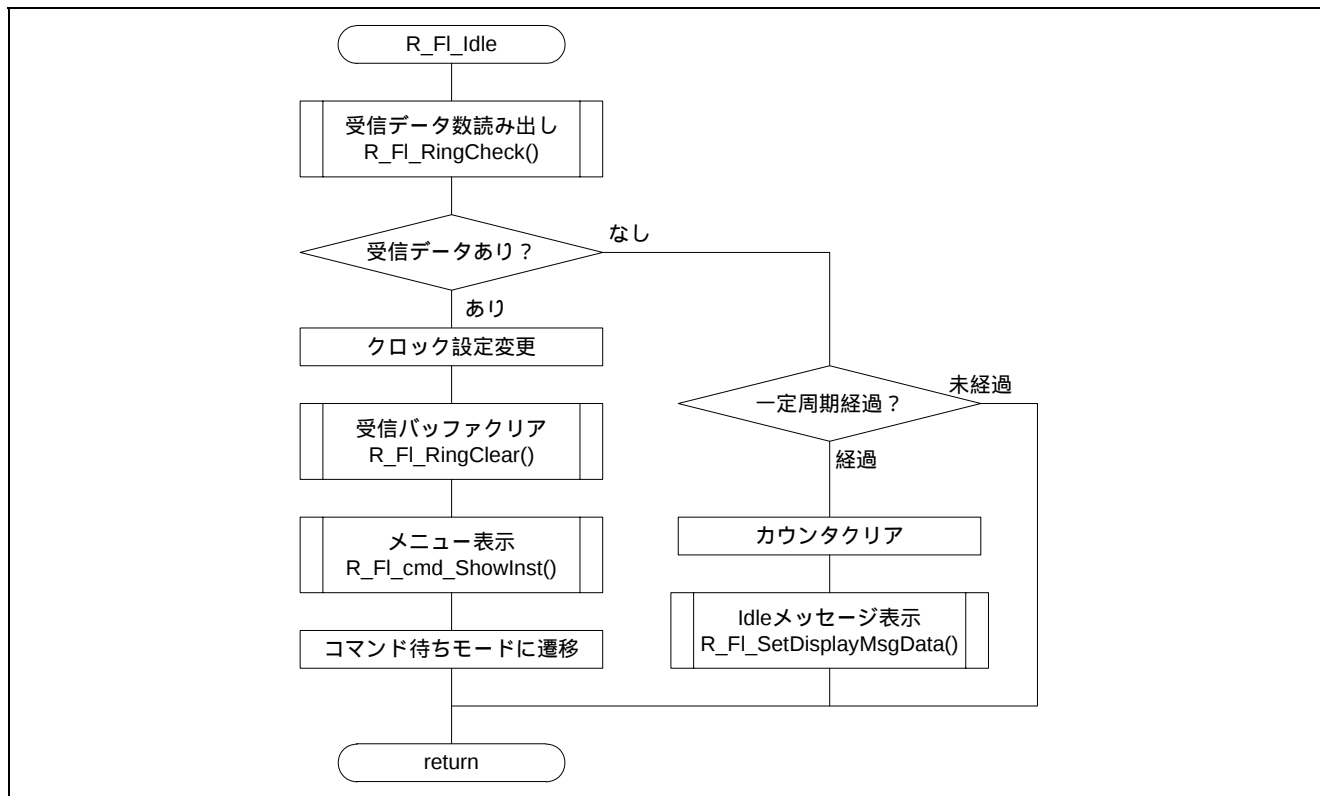
図5.11 Idle モード処理
