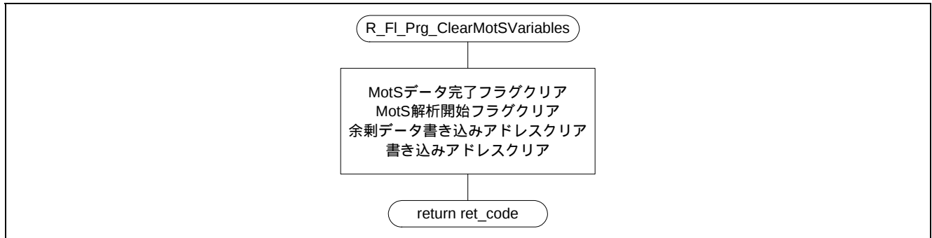
図5.30 Motorola S フォーマット用変数クリア
