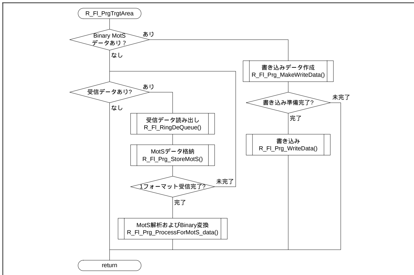
図5.14 書き込みモード処理
