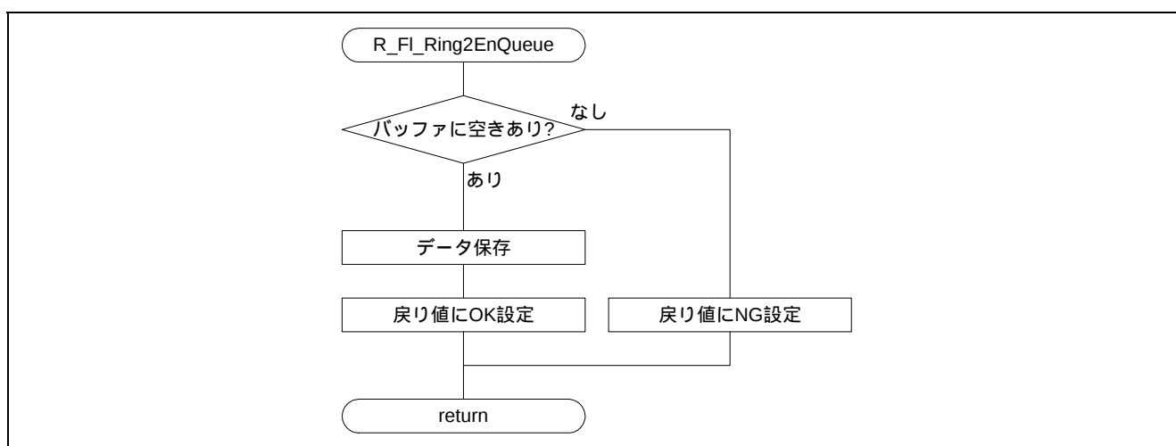
図5.42 送信用リングバッファへのデータ格納
