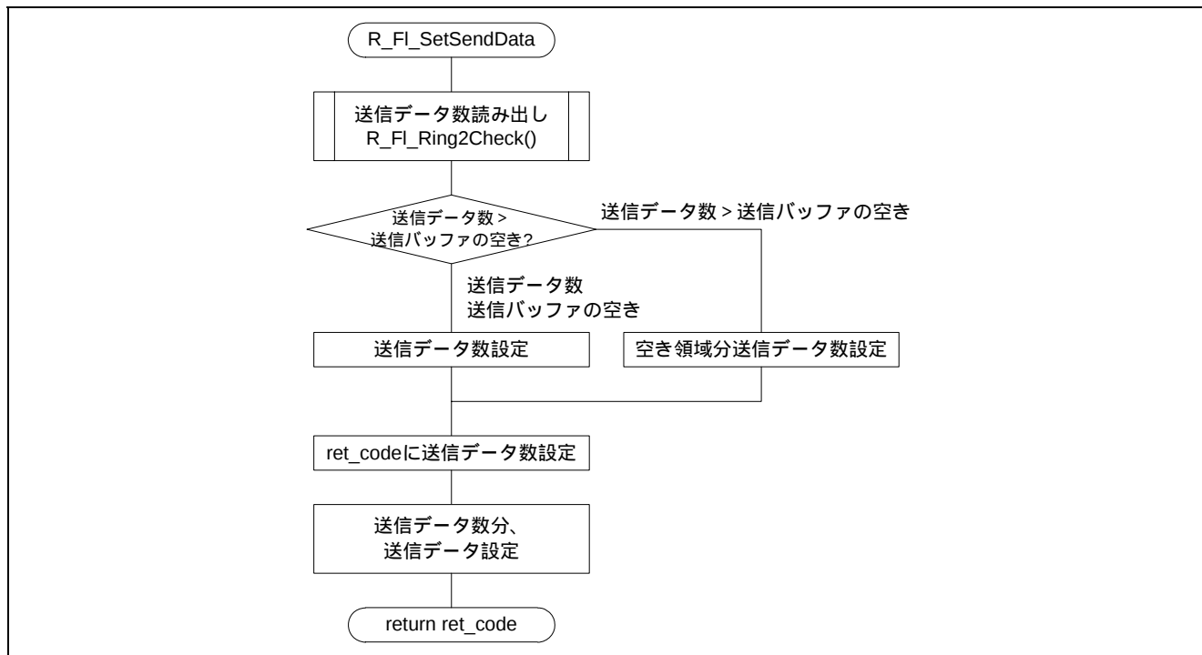
図5.33 USB 送信データ格納
