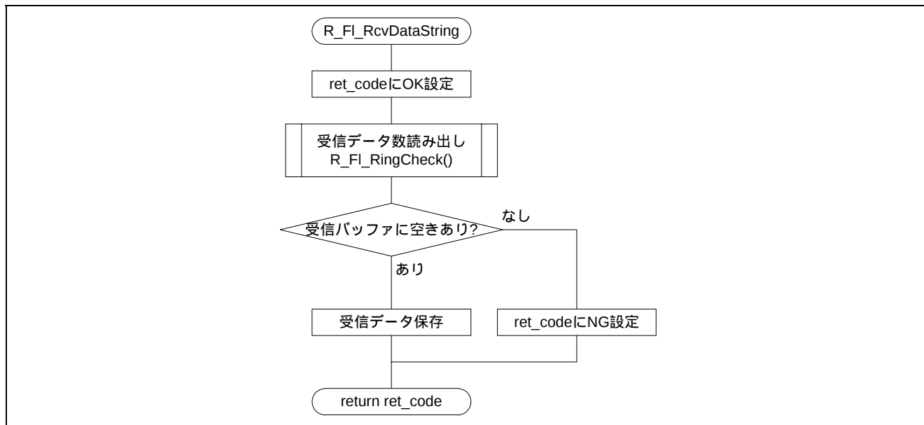
図5.32 USB 受信データ格納
