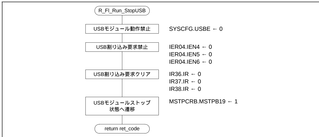
図5.31 USB 停止
