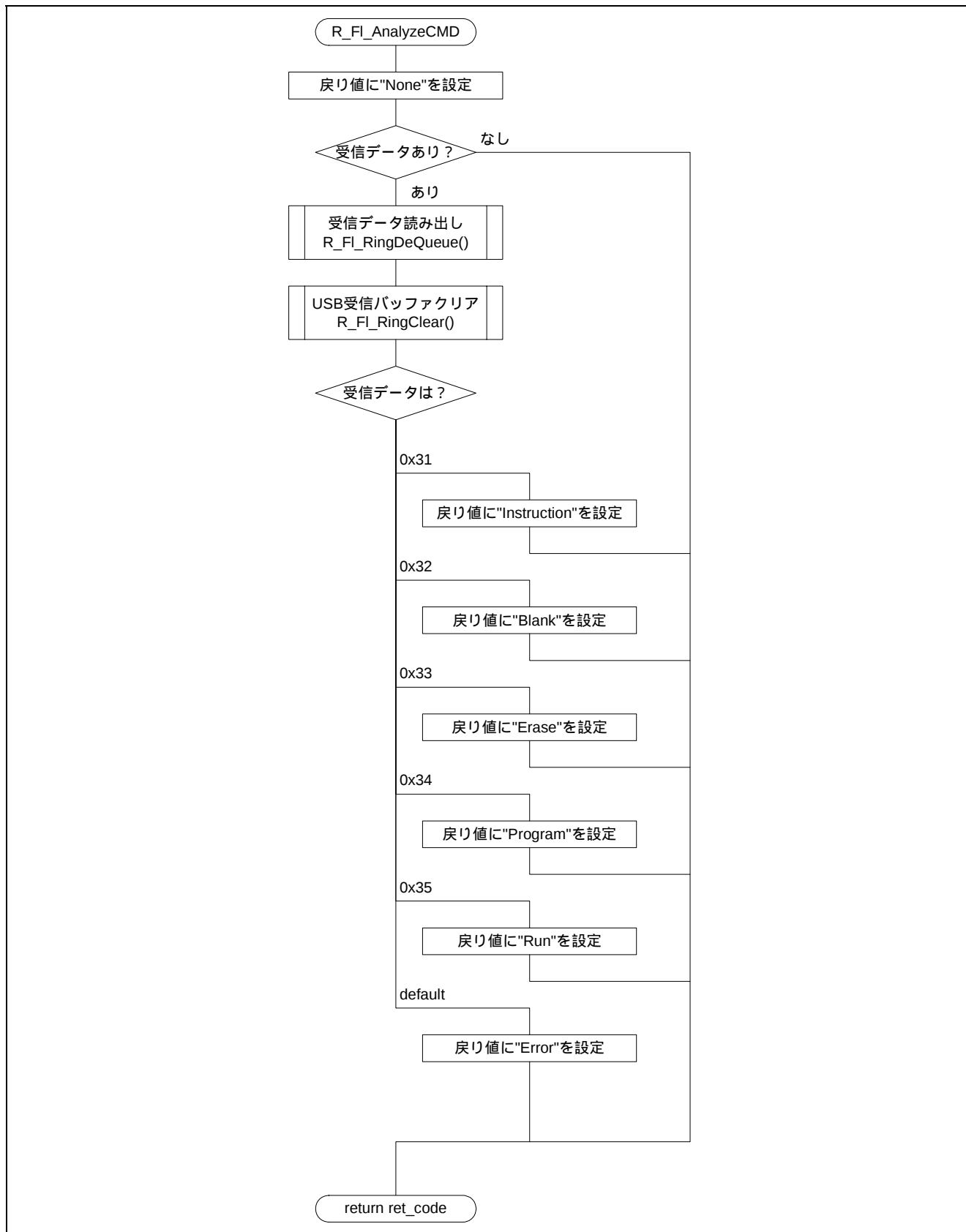
図5.12 コマンド解析
