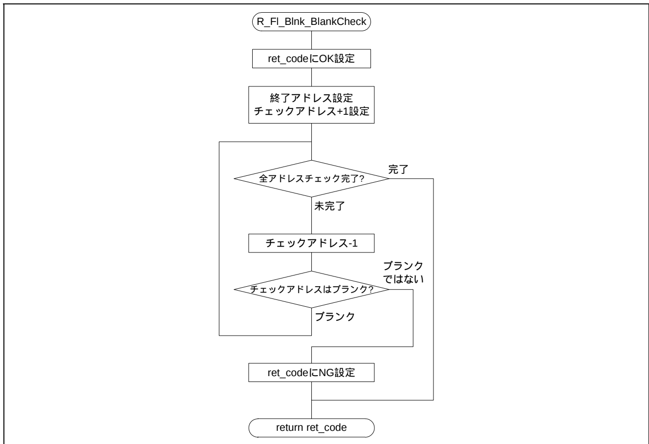
図5.22 ブランクチェック
