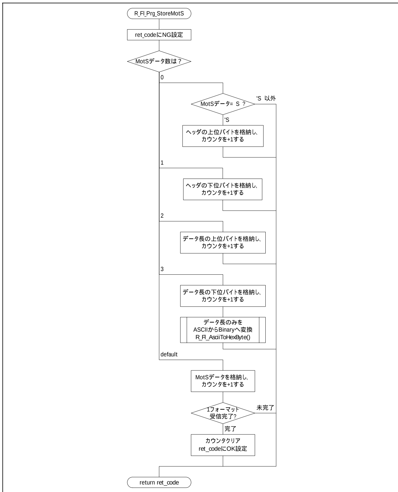
図5.24 Motorola S フォーマットデータ格納
