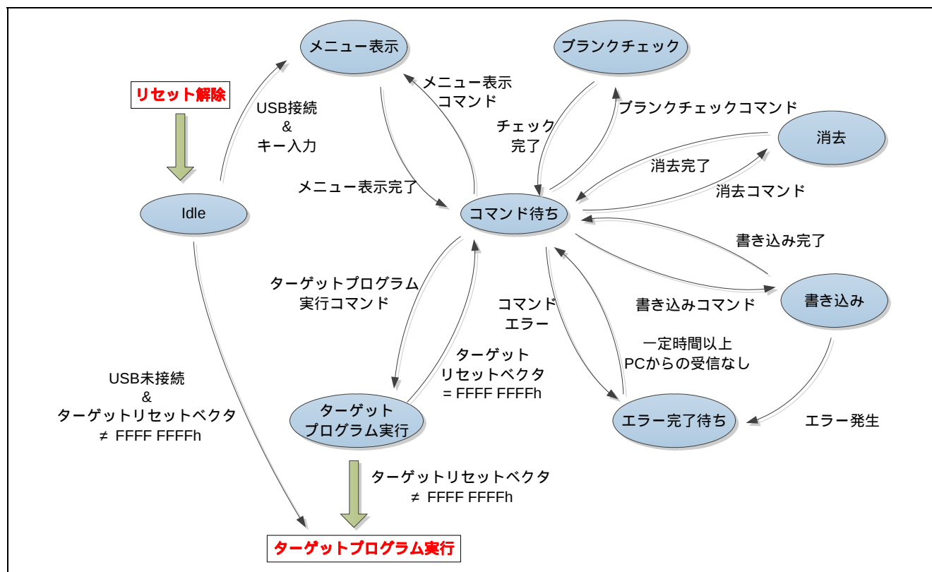
図5.5 モード遷移図
