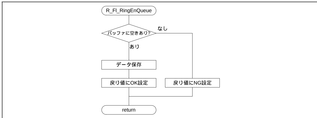
図5.38 受信用リングバッファへのデータ格納
