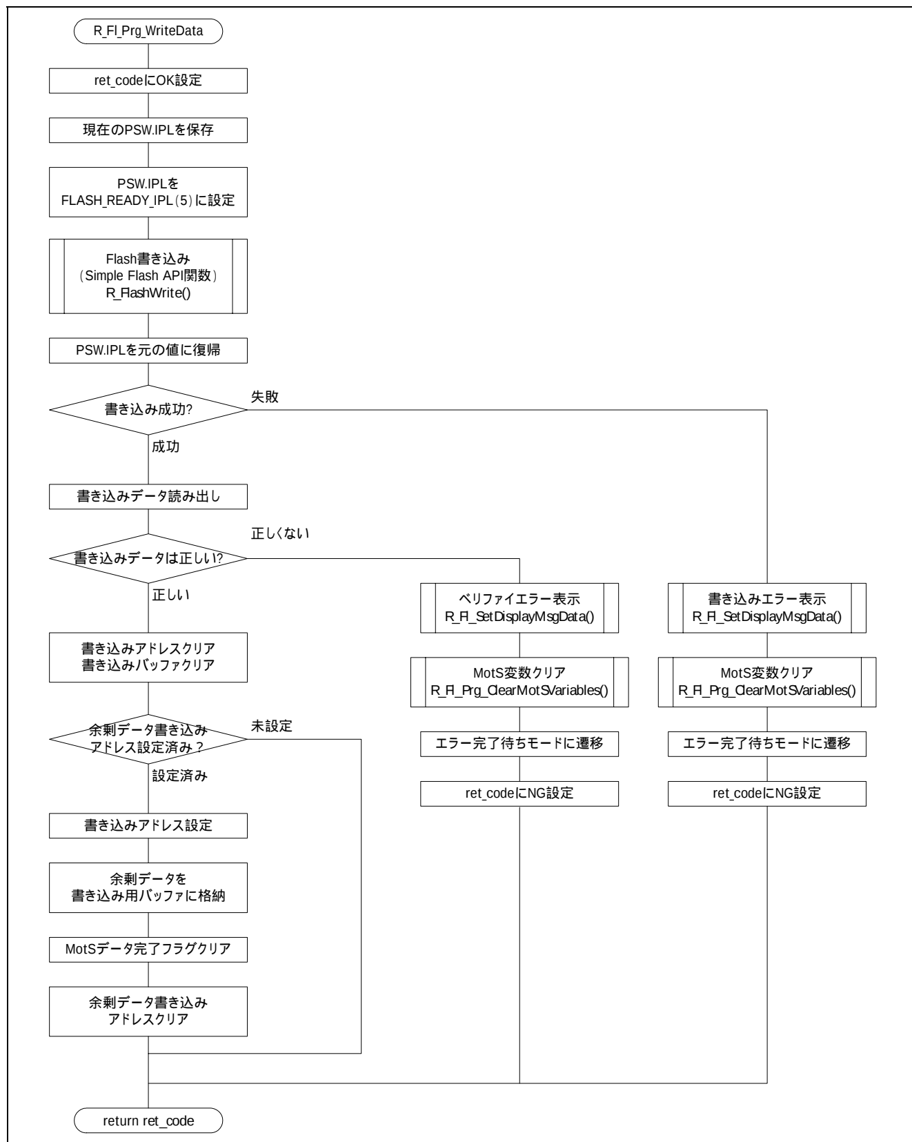
図5.29 ターゲットエリアへの書き込み
