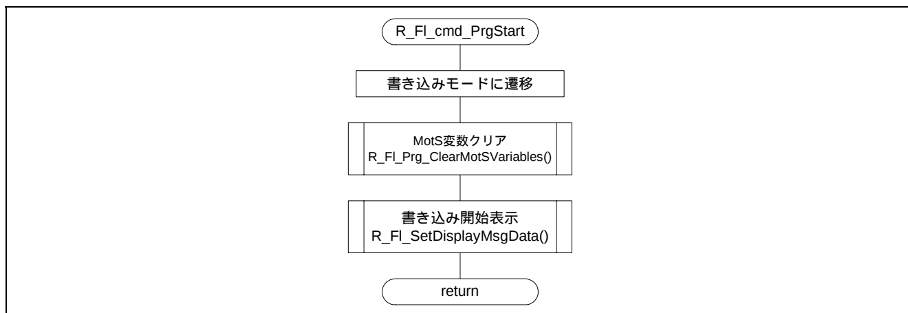
図5.20 書き込み開始
