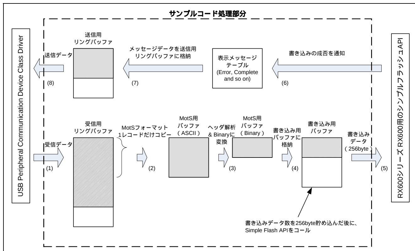
図5.6 書き込み時のデータの流れ
