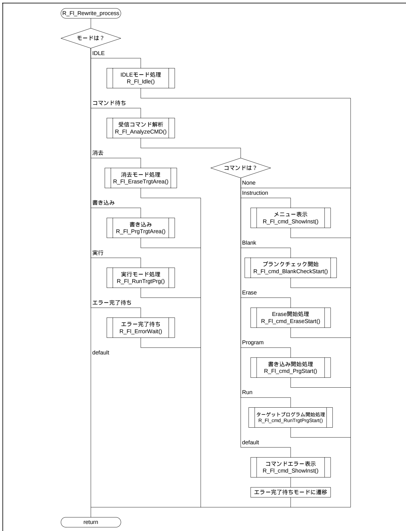
図5.10 書き込み処理メイン
