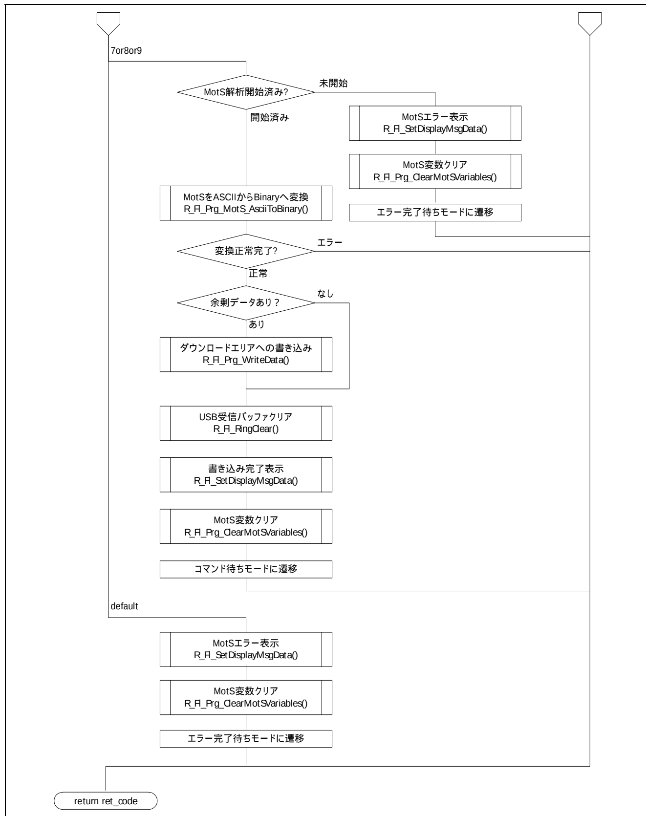
図5.26 Motorola S フォーマットヘッダ解析、および Binary 変換
