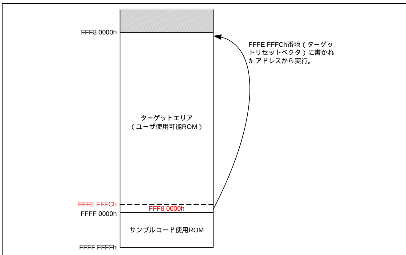
図5.4 ターゲットリセットベクタ
