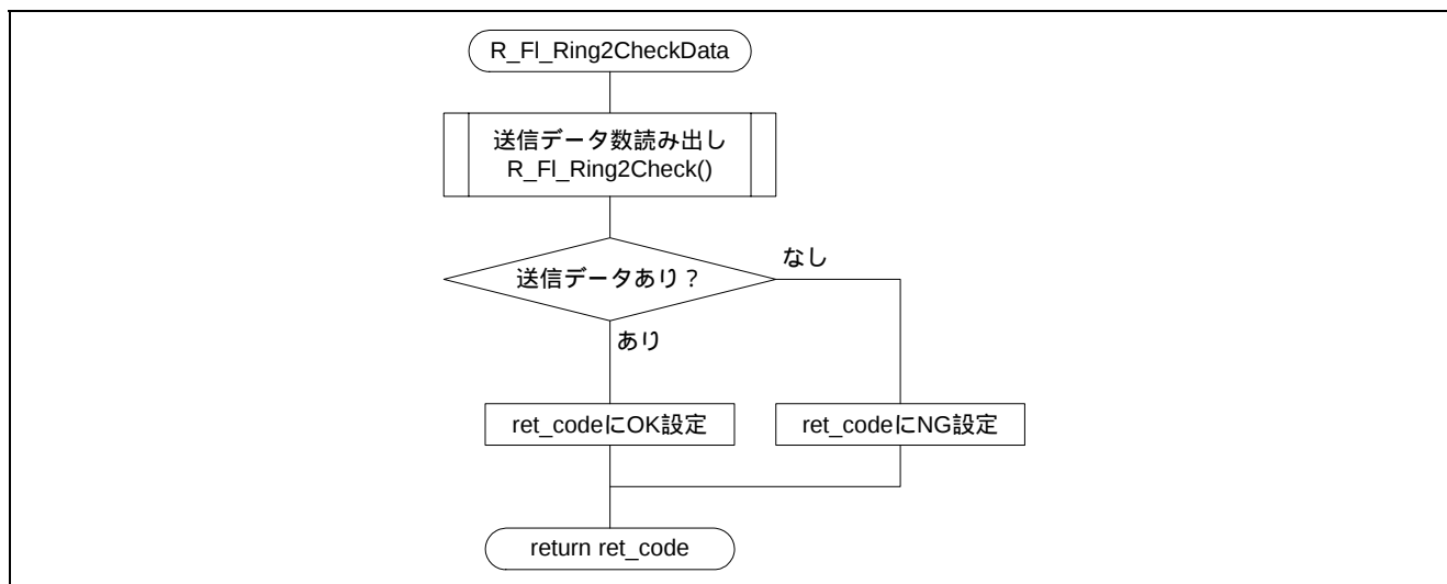
図5.36 送信用リングバッファのデータ確認
