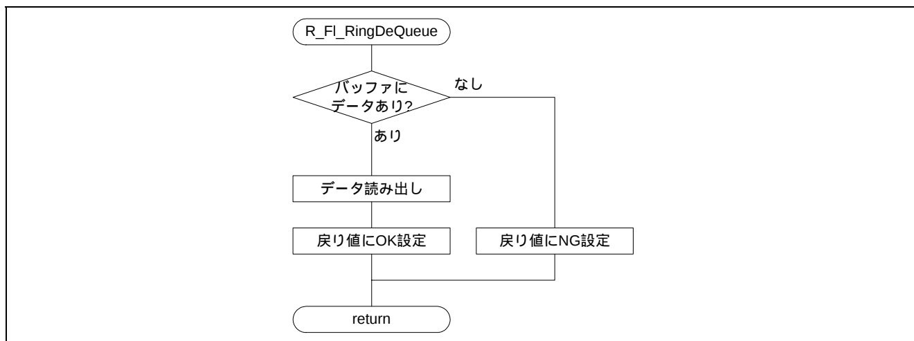
図5.39 受信用リングバッファからのデータ読み出し
