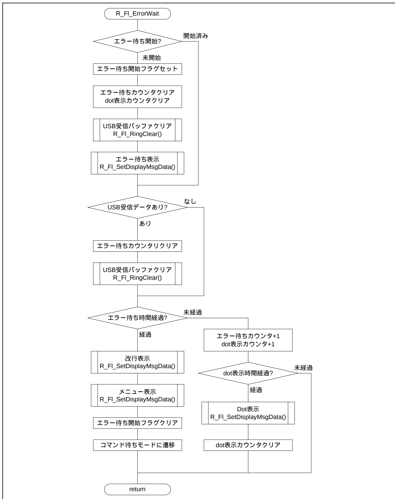
図5.16 エラー完了待ちモード処理
