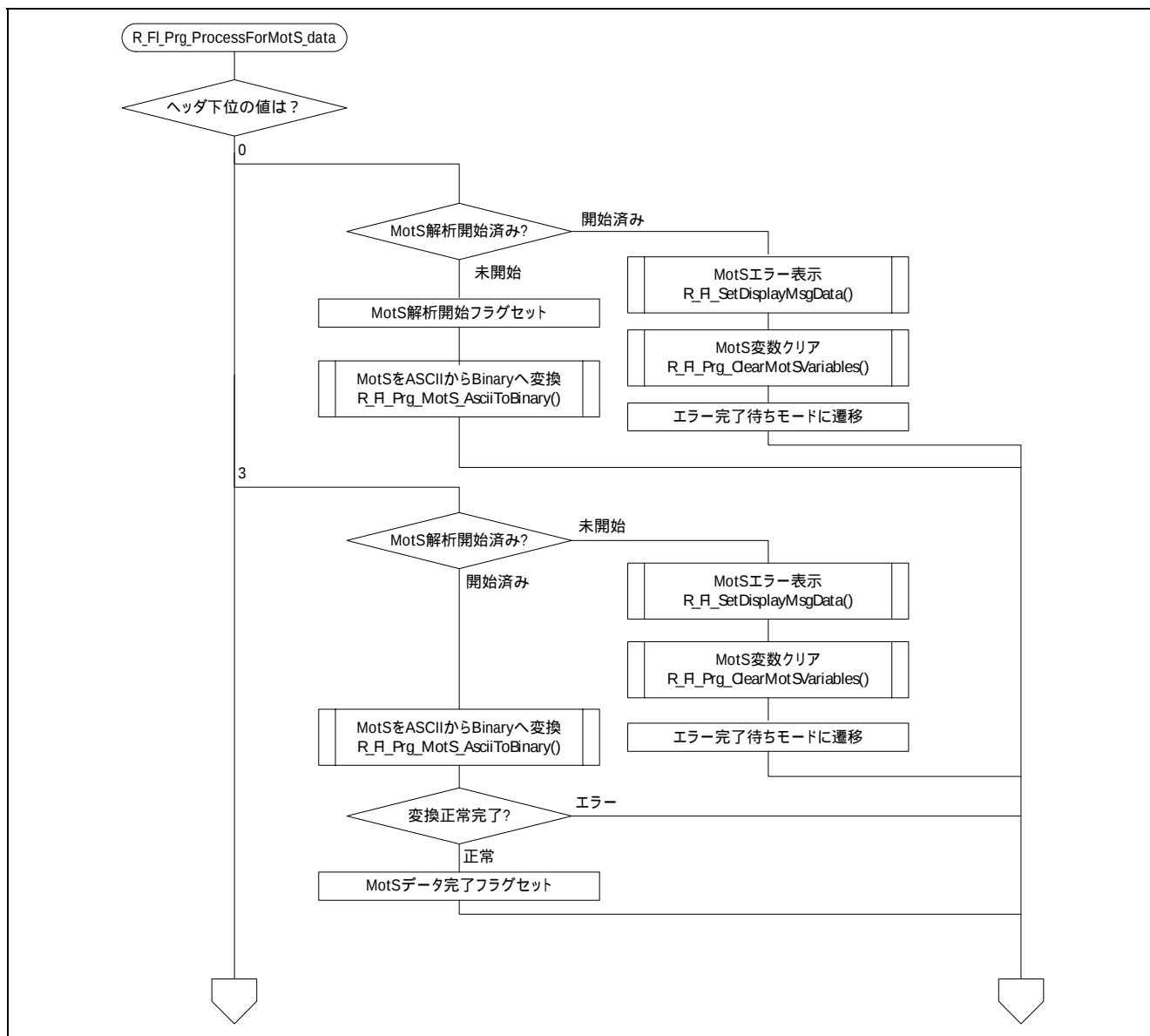
図5.25 Motorola S フォーマットヘッダ解析、および Binary 変換
