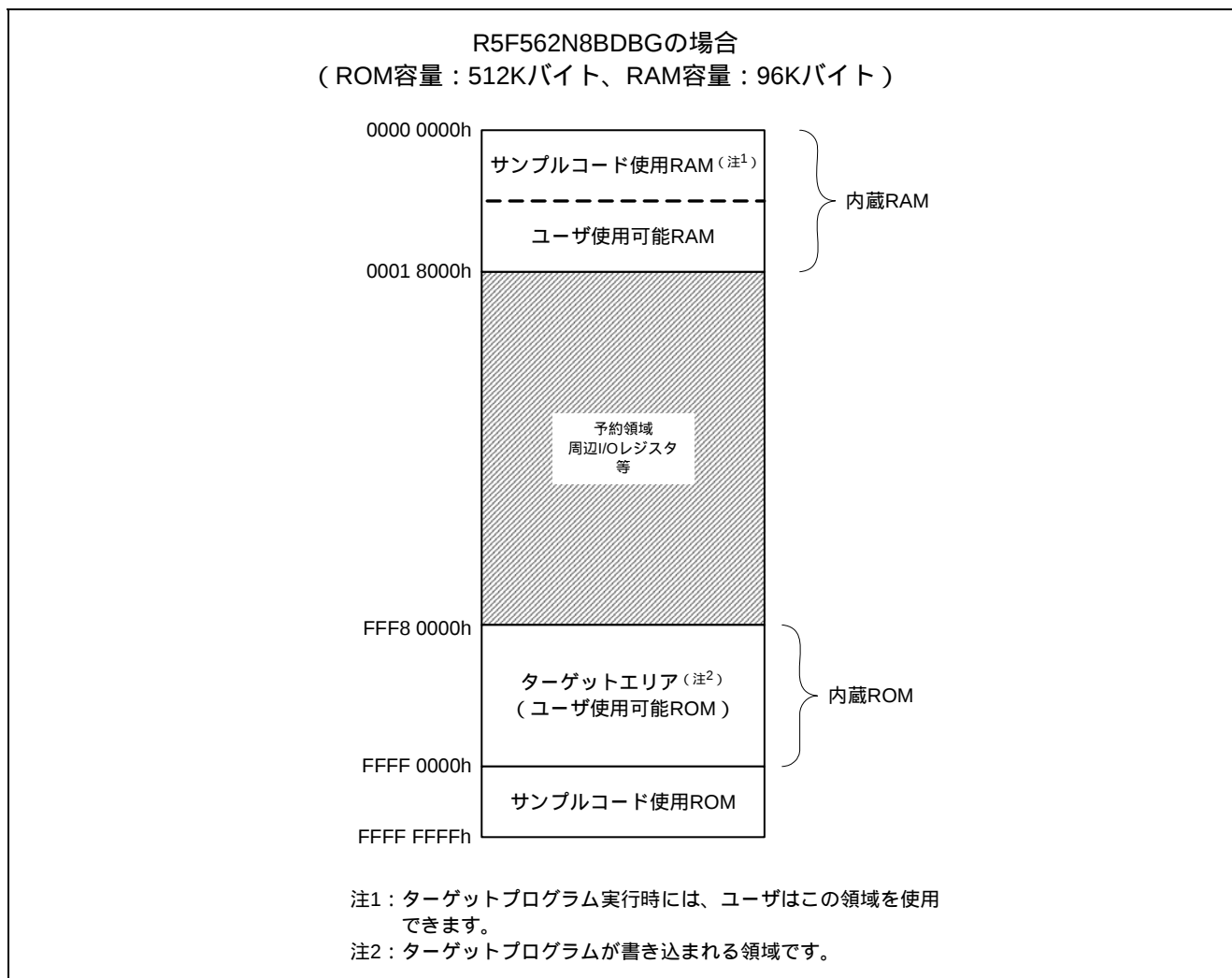
図5.1 メモリ配置
