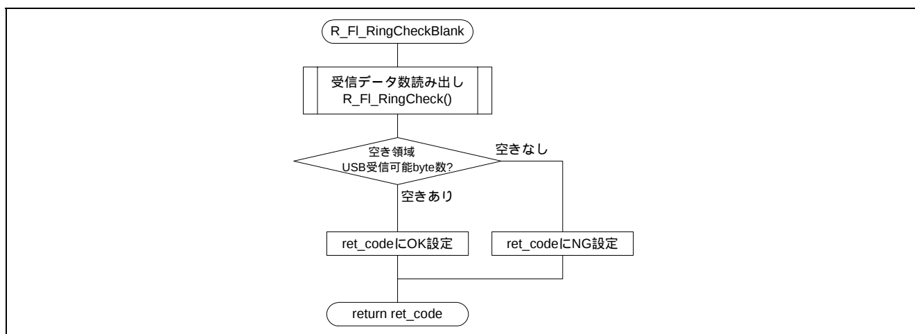
図5.35 受信用リングバッファの空き容量確認
