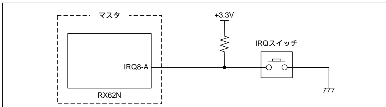
図 10 マスタの IRQ スイッチ接続図
