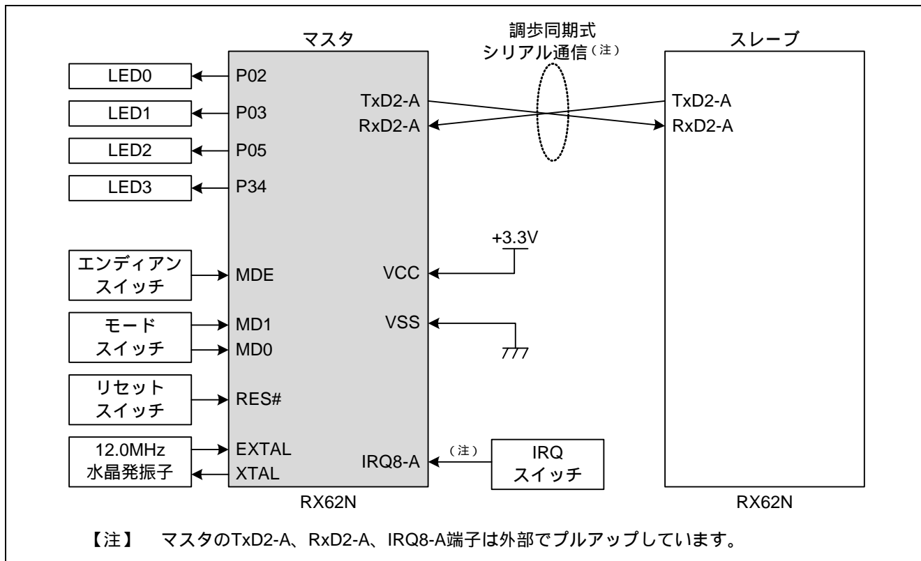
図 2 マスタのハードウェア構成図
