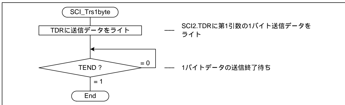
図 17 フローチャート (SCI_Trns1byte) (マスタ)
