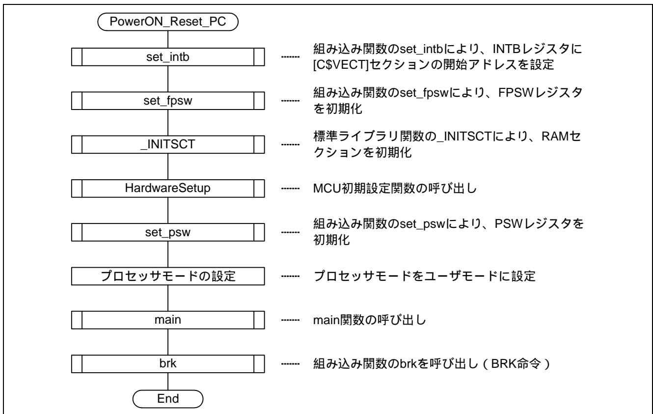
図 12 フローチャート (PowerON_Reset_PC) (マスタ)
