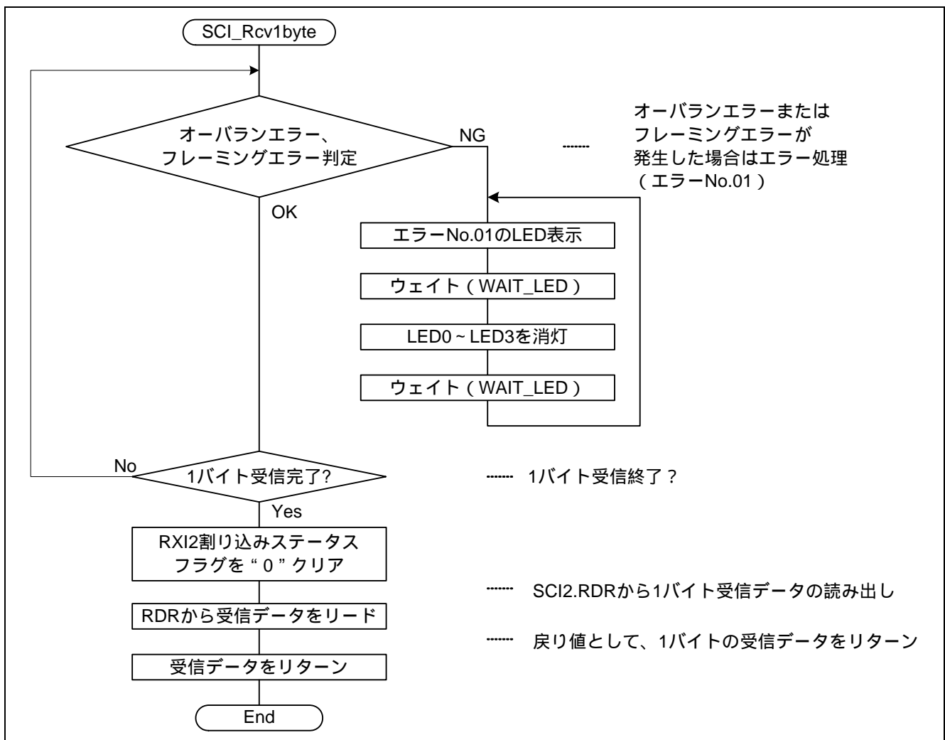
図 19 フローチャート (SCI_Rcv1byte) (マスタ)
