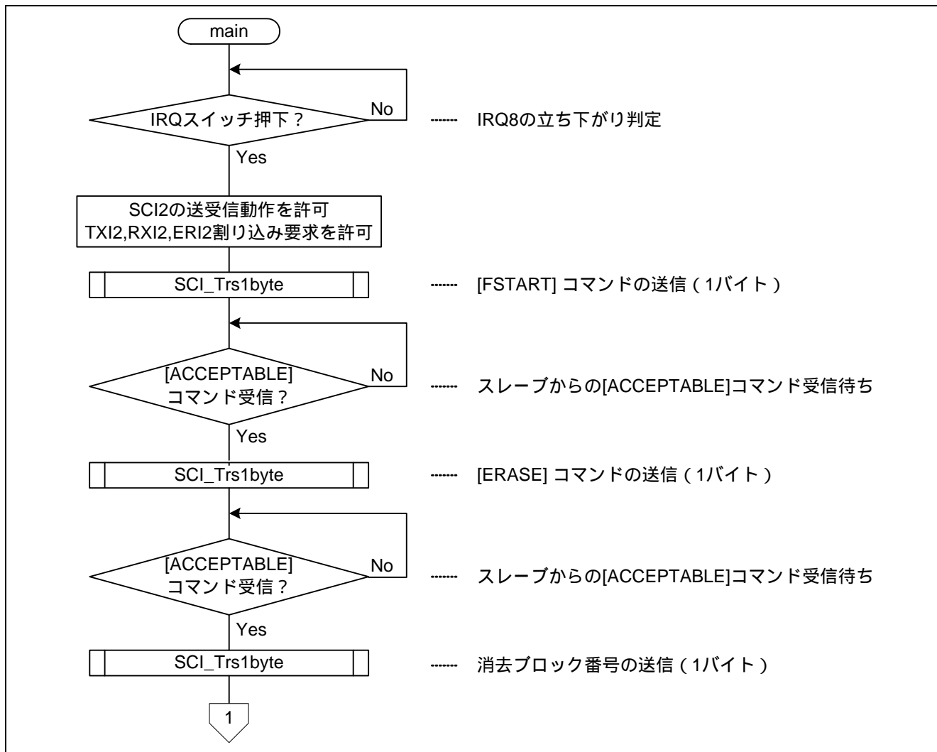
図 14 フローチャート (main) (1) (マスタ)
