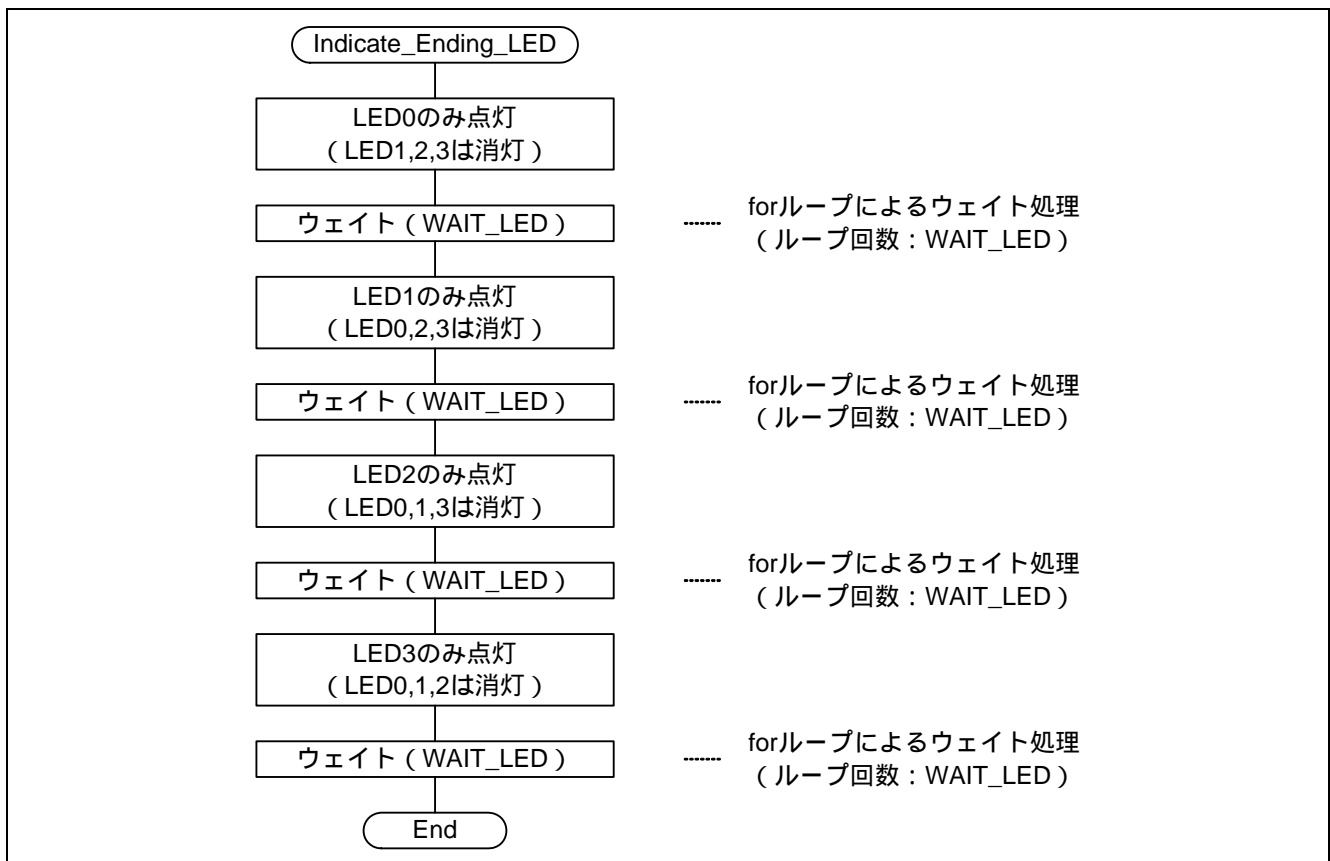
図 16 フローチャート (Indicate_Ending_LED) (マスタ)
