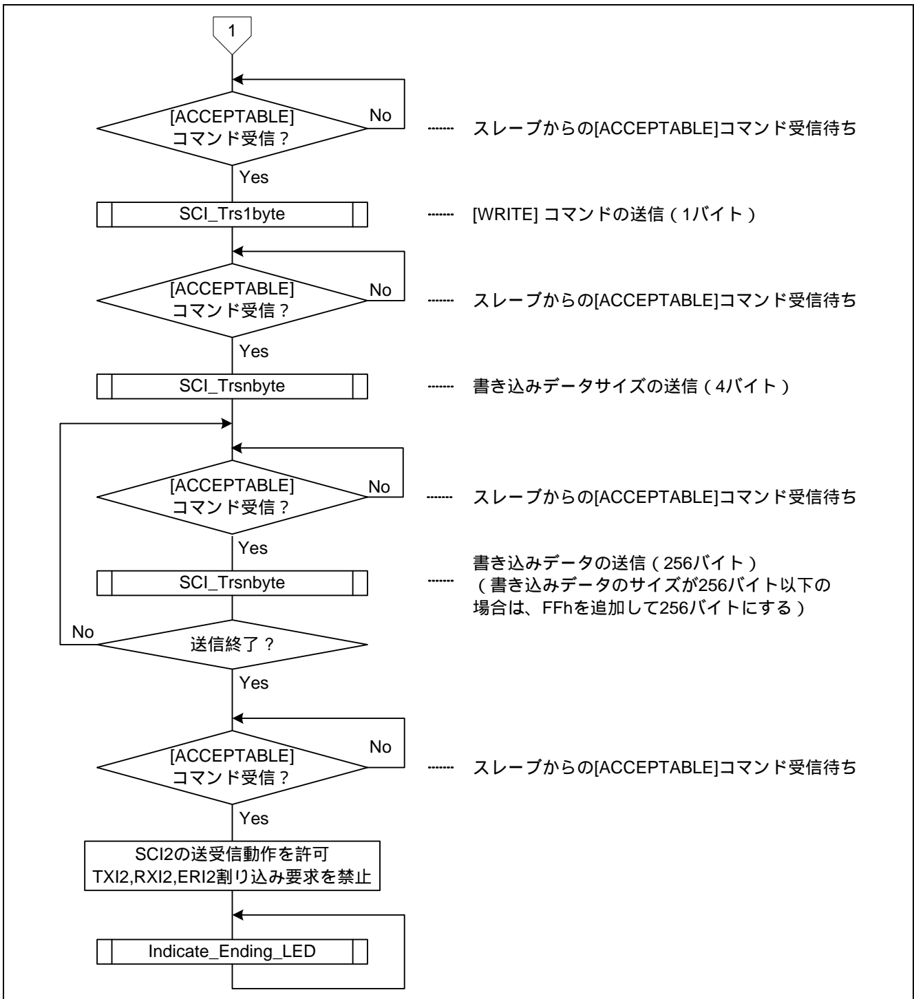
図 15 フローチャート (main) (2) (マスタ)
