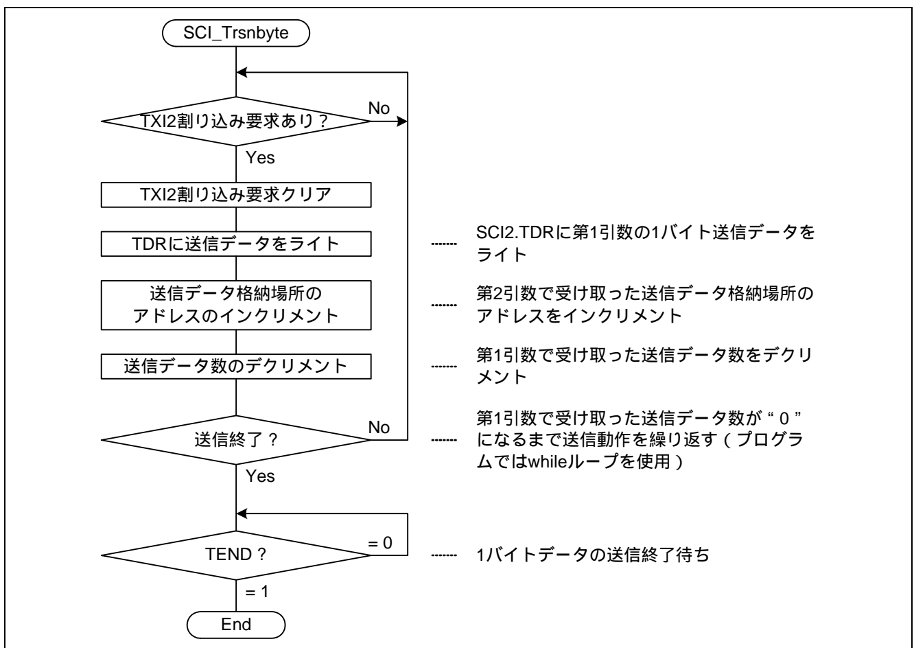
図 18 フローチャート (SCI_Trnsbyte) (マスタ)
