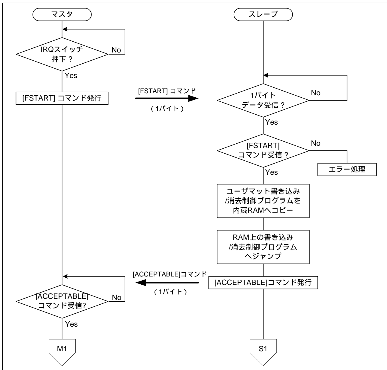
図3 通信フロー (1)
