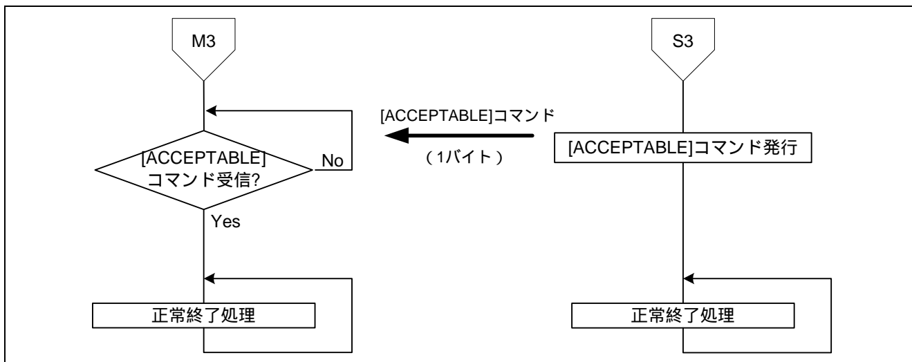
図 6 通信フロー (4)
