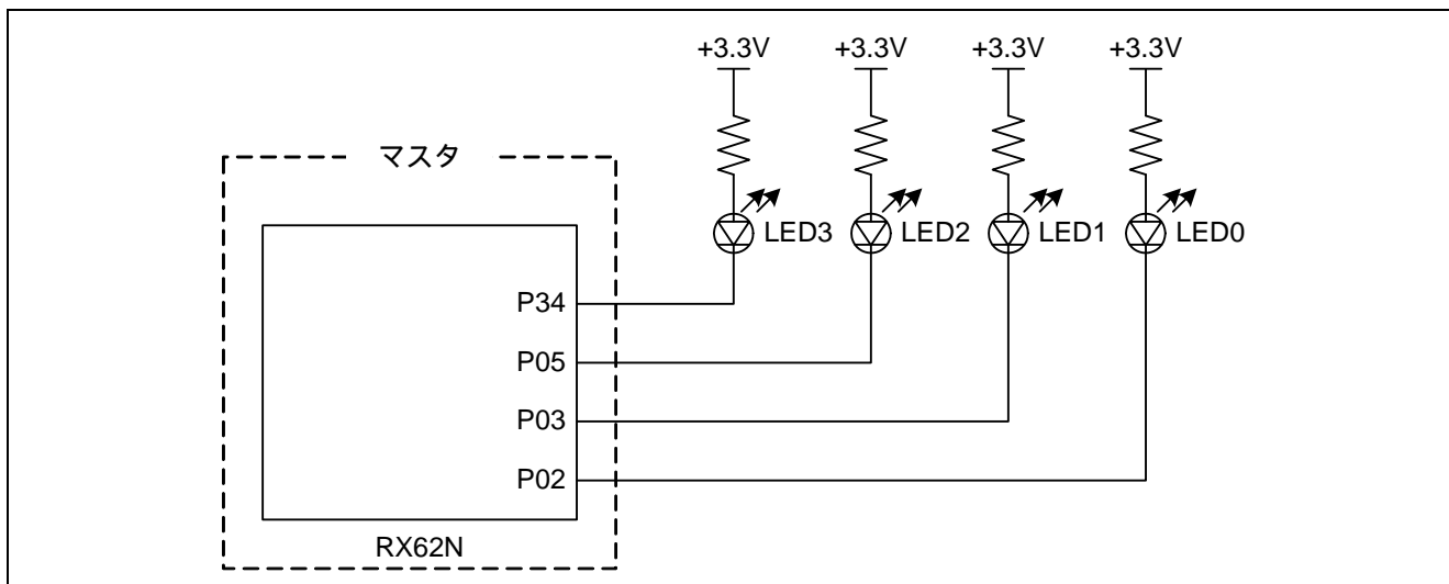
図 9 マスタの LED 接続図
