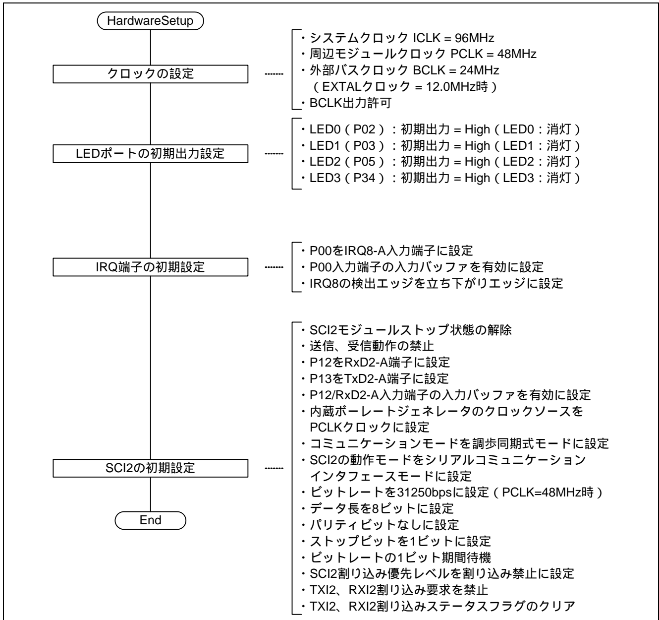
図 13 フローチャート (HardwareSetup) (マスタ)
