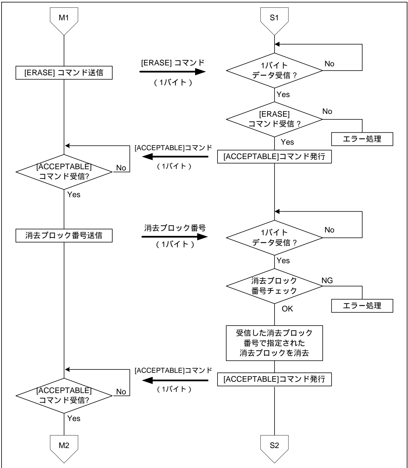
図 4 通信フロー (2)
