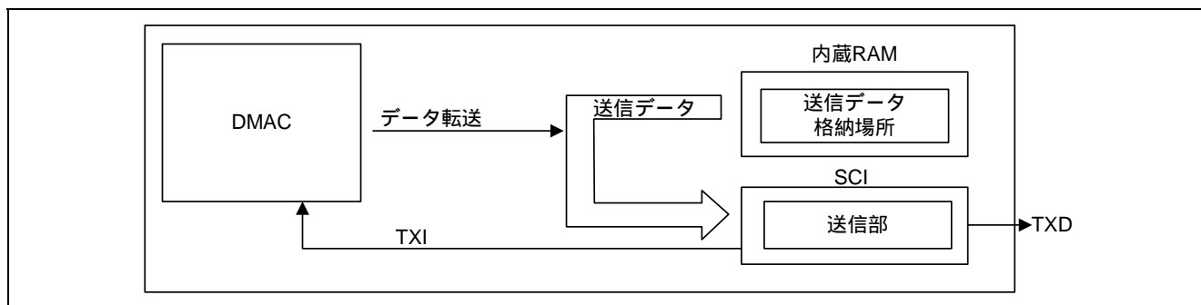
図 1 DMAC を用いた調歩同期式シリアルデータ送信の概要
