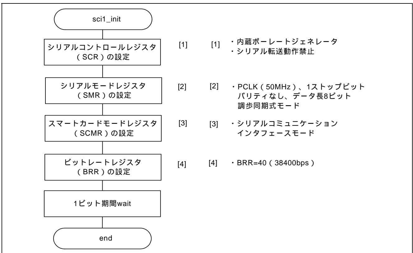
図 10 SCI 初期設定
