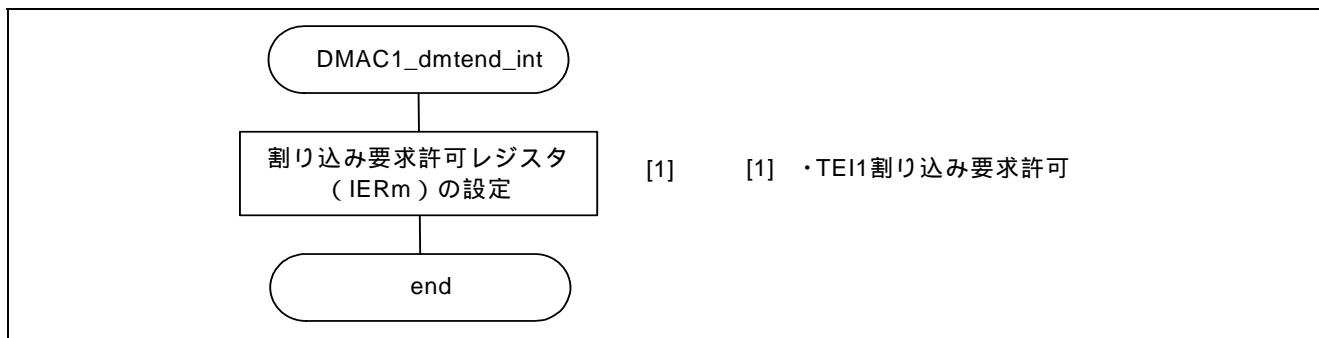
図 11 DMAC1 転送終了割り込み処理
