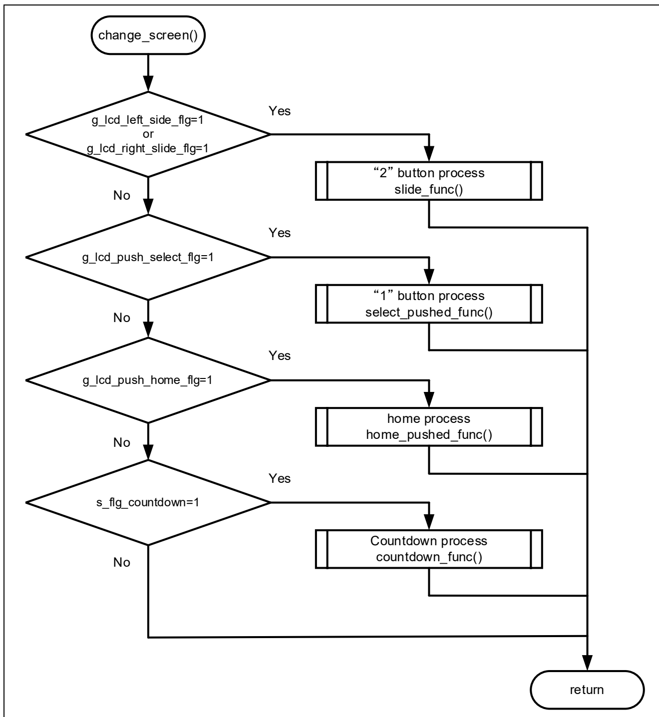
図 4-5 タッチ操作時の処理のフローチャート
