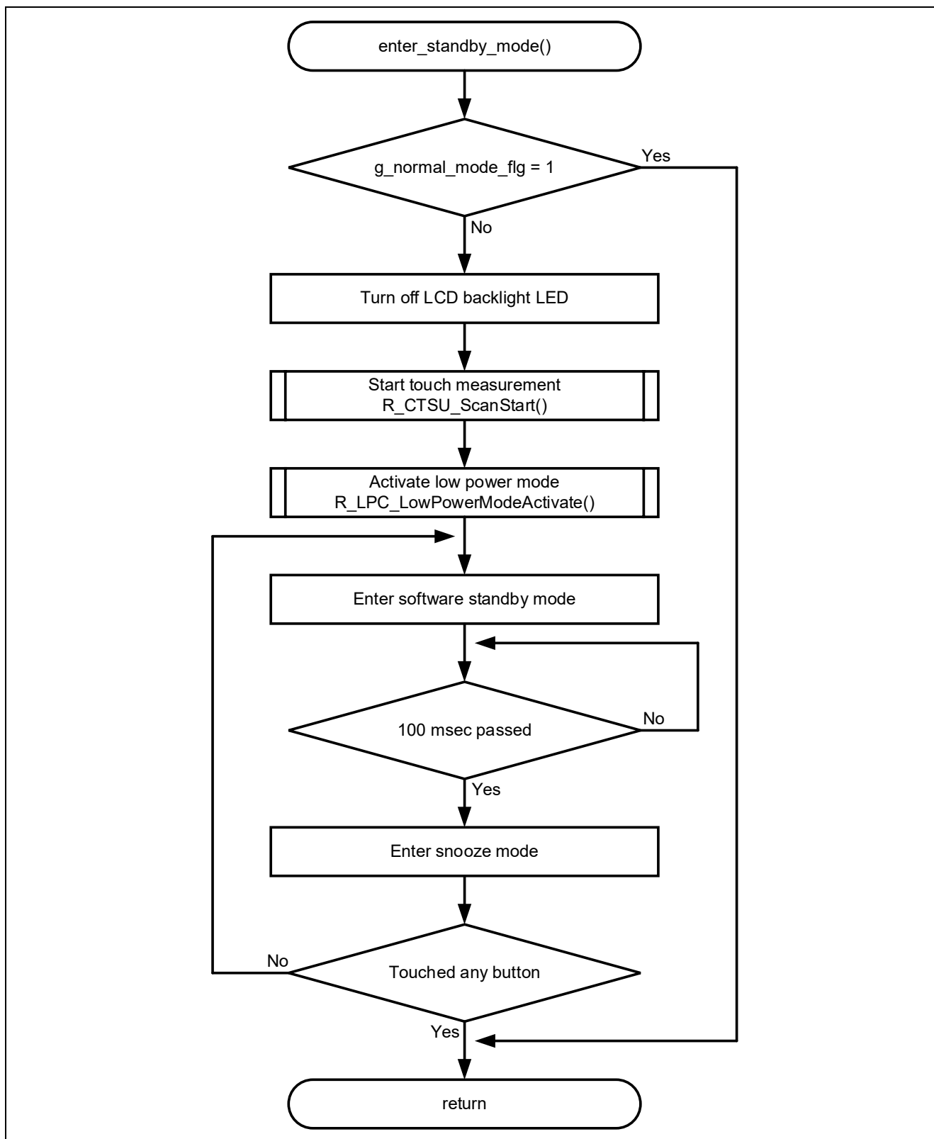
図 4-12 ソフトウェアスタンバイモード遷移と低消費電力計測のフローチャート
