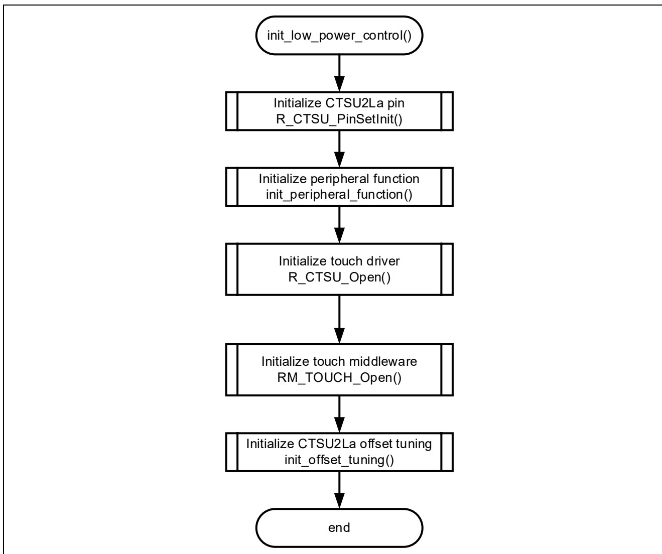
図 4-10 CTSU2SLa 初期化のフローチャート
