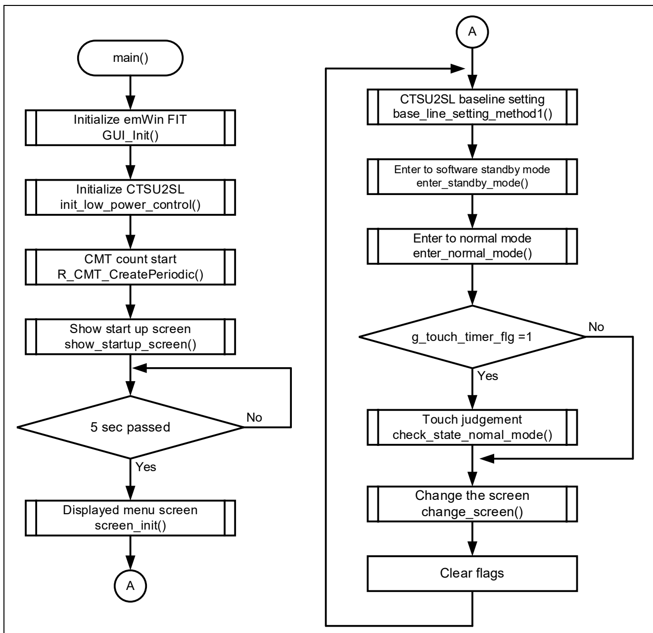
図 4-4 全体フローチャート
