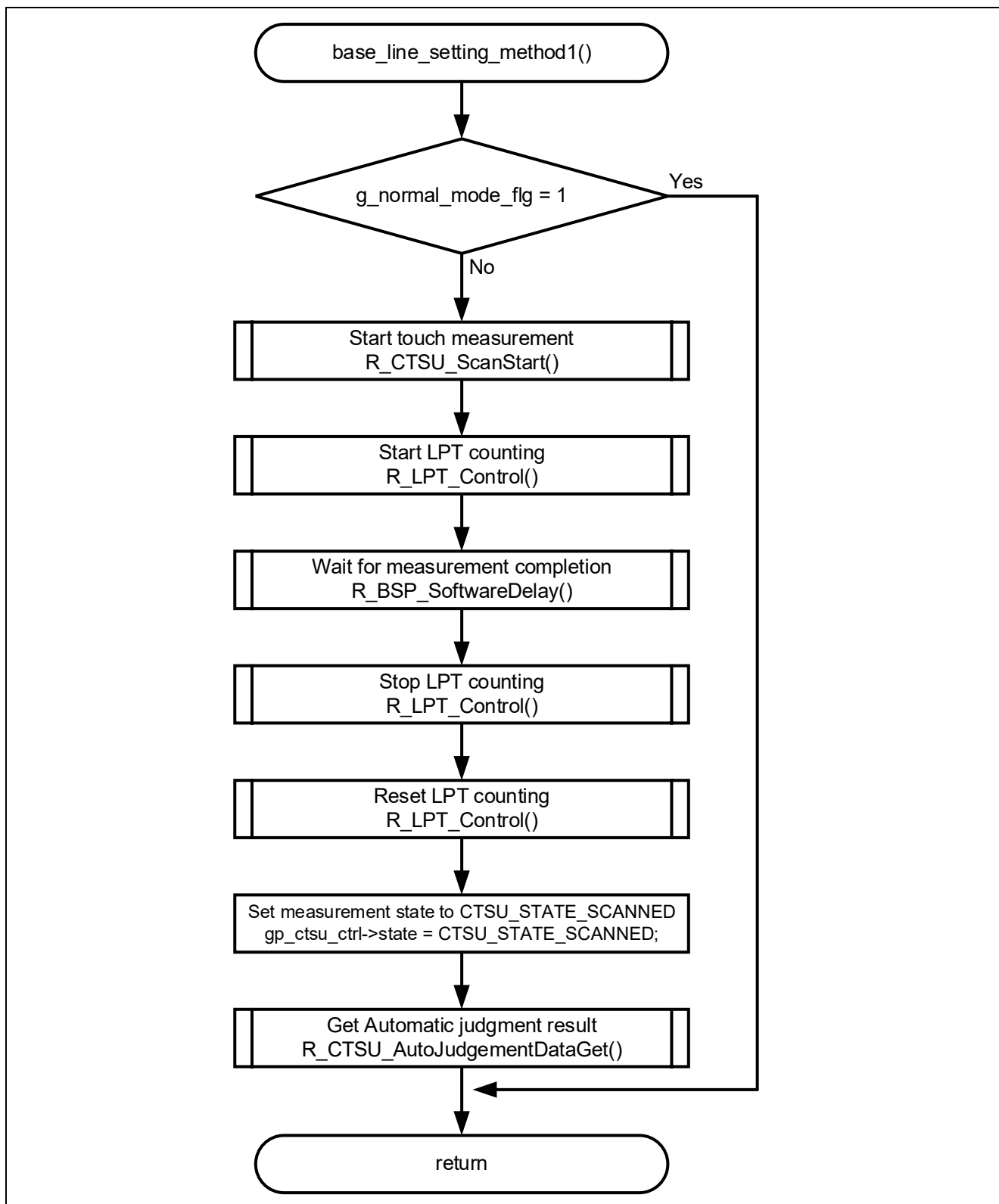
図 4-11 CTSU2SLa ベースライン設定のフローチャート
