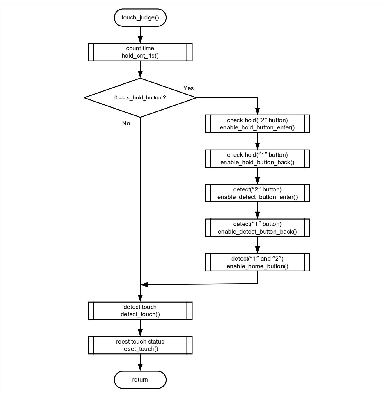
図 4-15 タッチ判定のフローチャート
