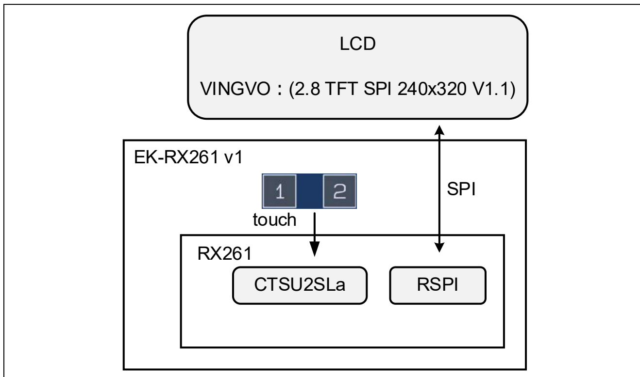
図 1-1 システムの構成
