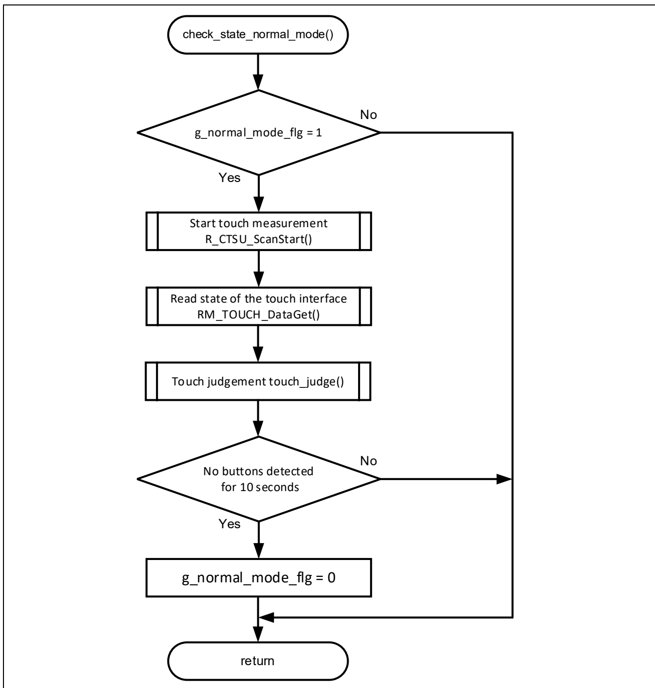
図 4-14 CTSU2SLa 通常計測のフローチャート
