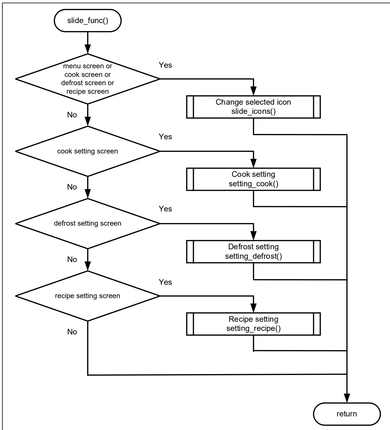
図 4-6 「2」 ボタンタッチ、長押し時のフローチャート
