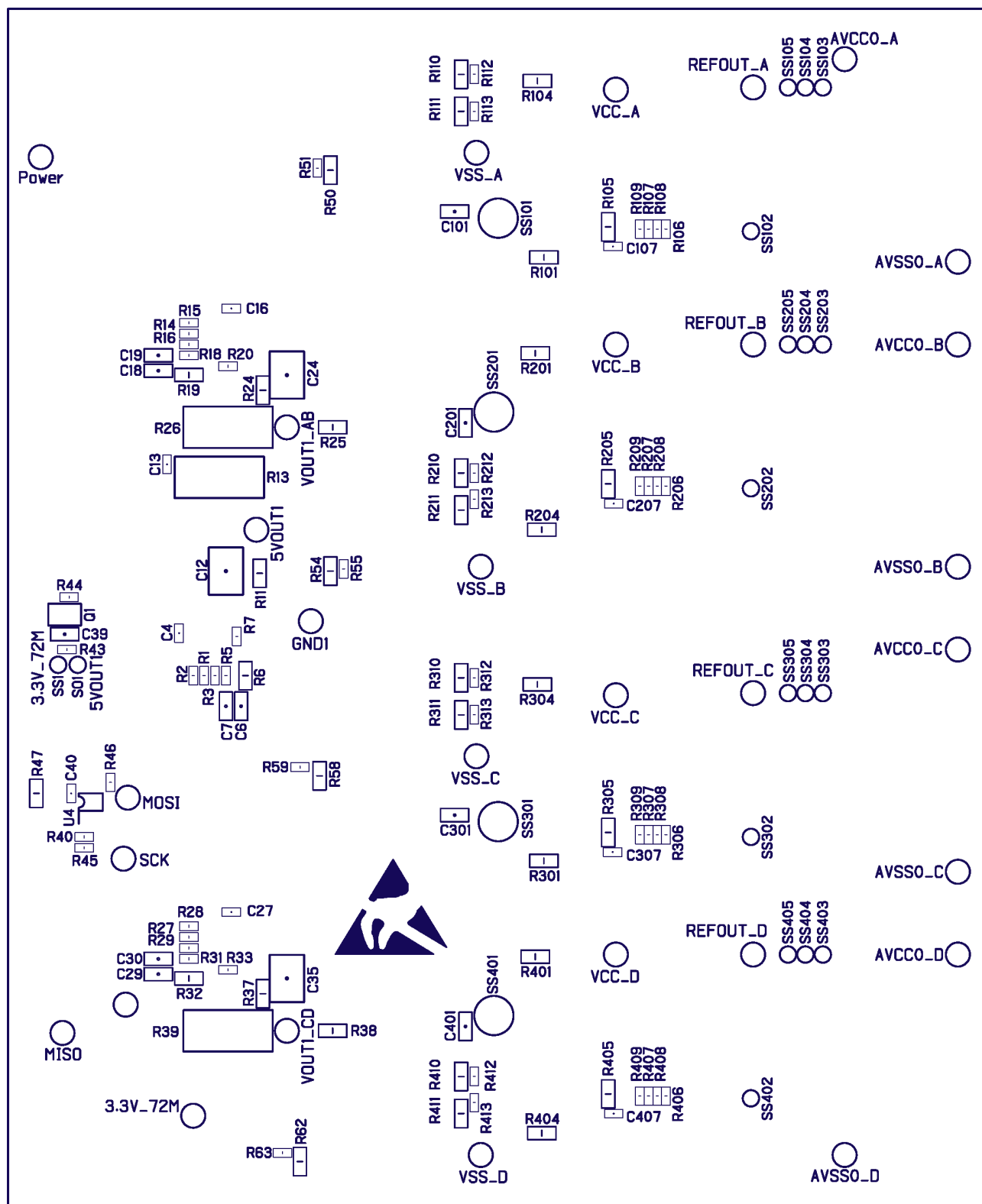
半田面シルク（半田面視）
