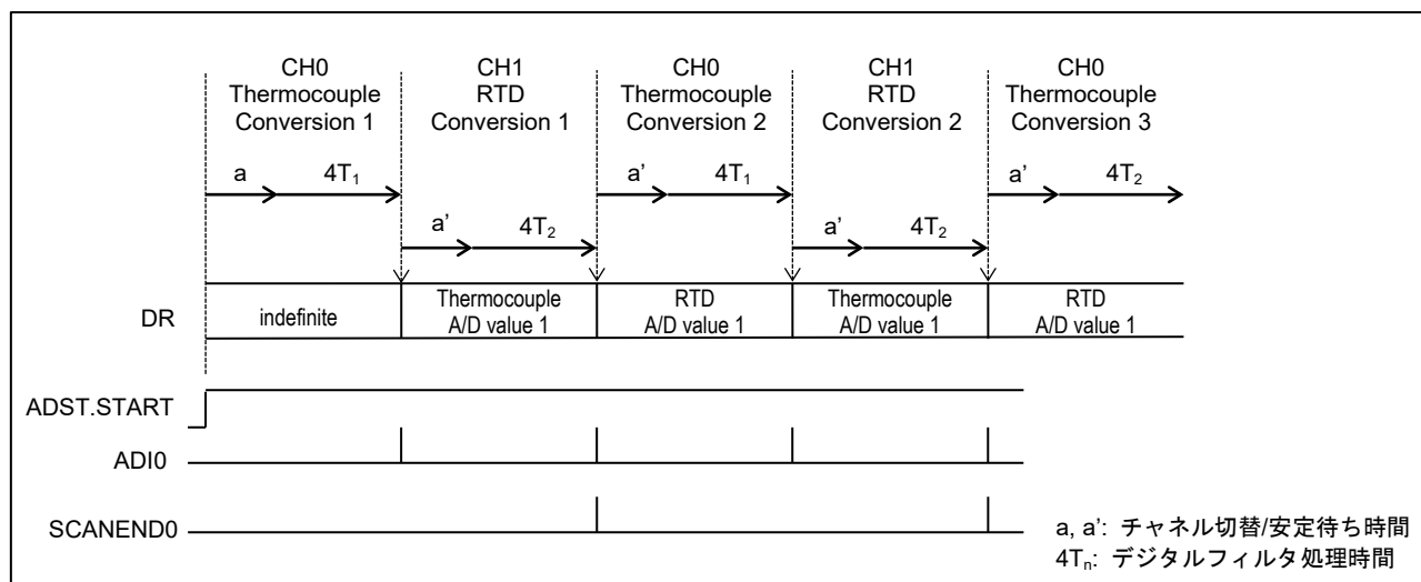
図 6-2 温度計測の A/D 変換シーケンス
