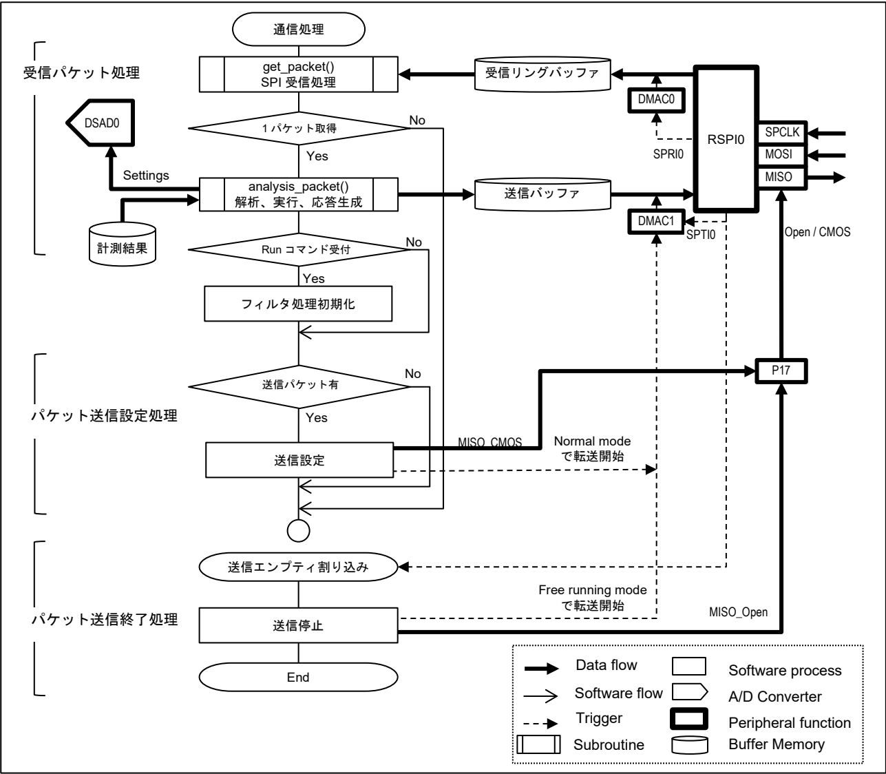
図 7-4 通信処理フロー
