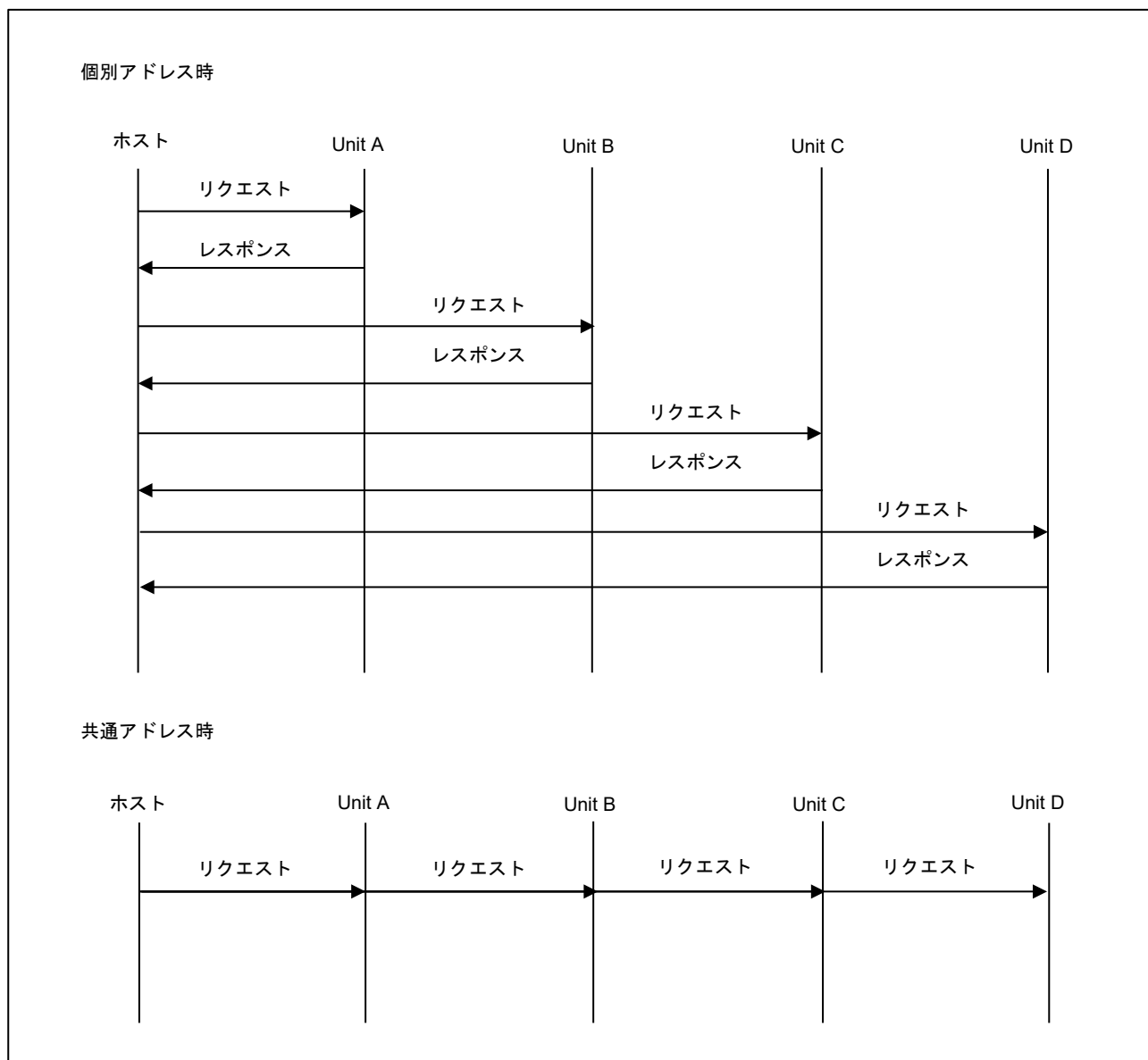
図 7-2 通信シーケンス
