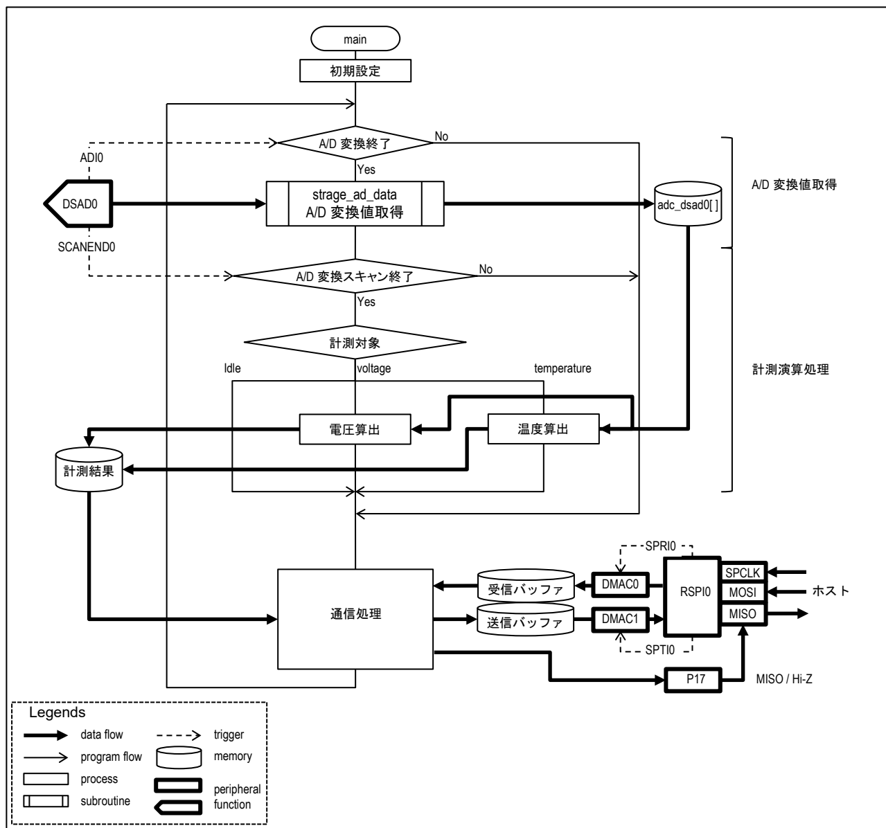
図 7-3 RX23E-A プログラムフロー
