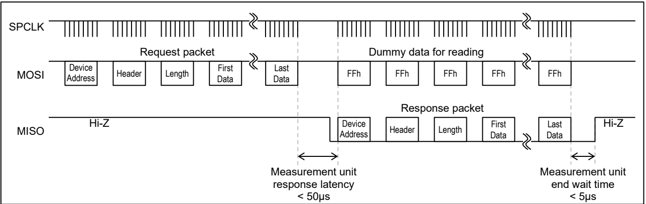
図 7-1 SPI 通信タイミングチャート
