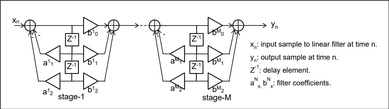
図 6-5 IIR Biquad フィルタ
