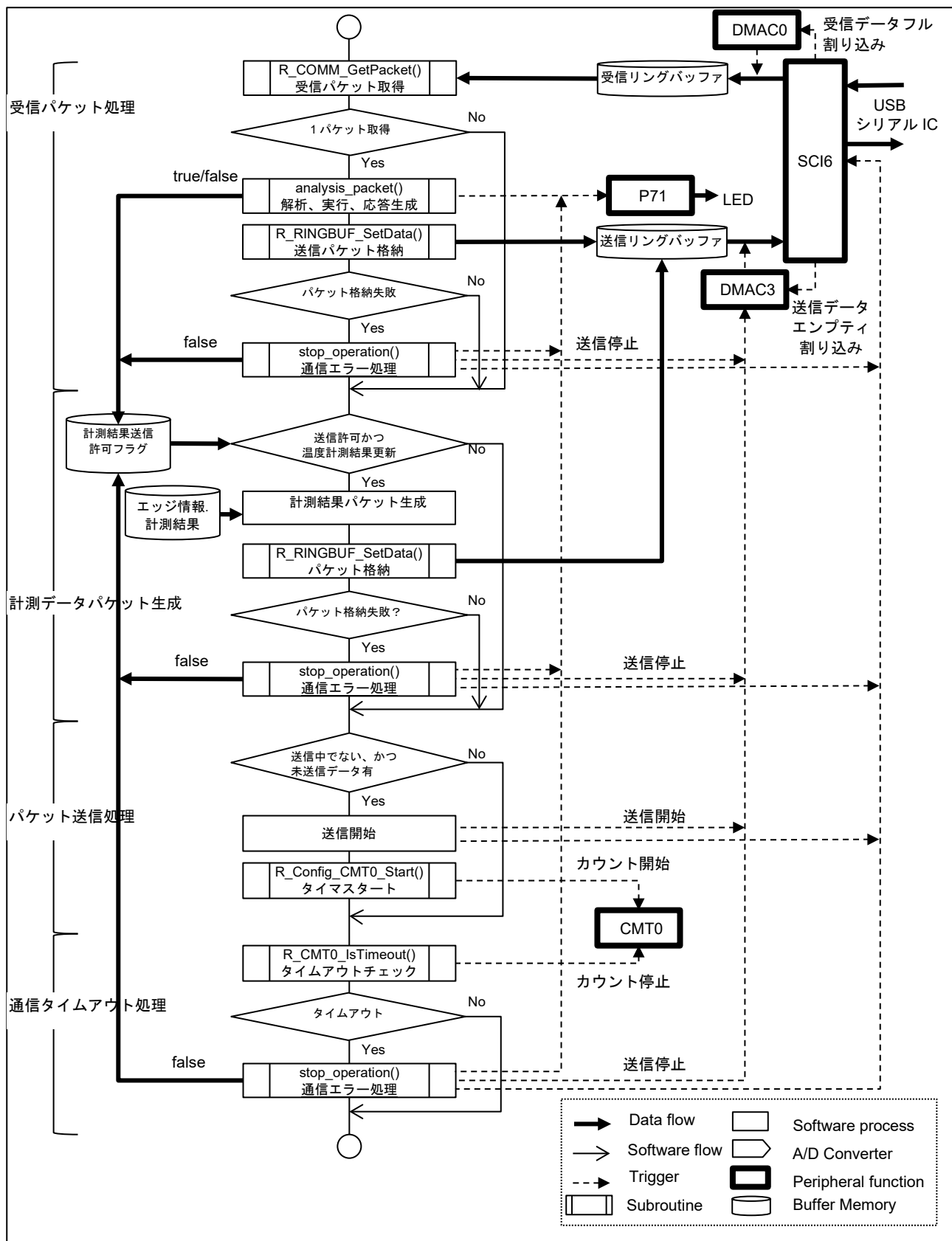
図 7-8 PC ツール通信処理フロー
