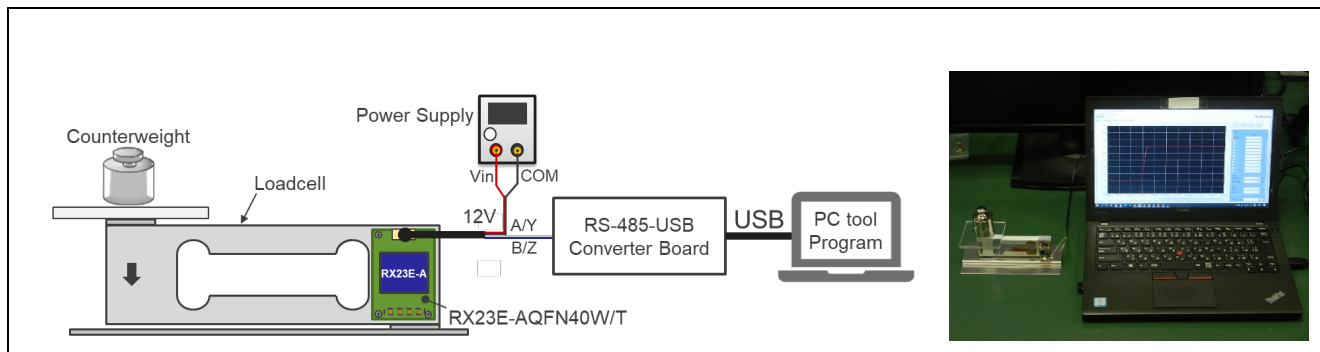
図 3-1 ロードセルによる重量計測の構成と計測時の様子
