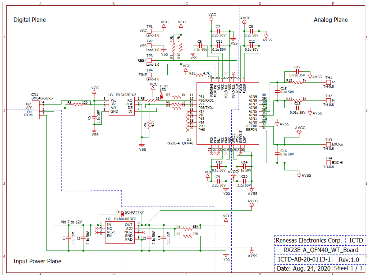
図 2-1 RX23E-AQFN40W/T 回路図
