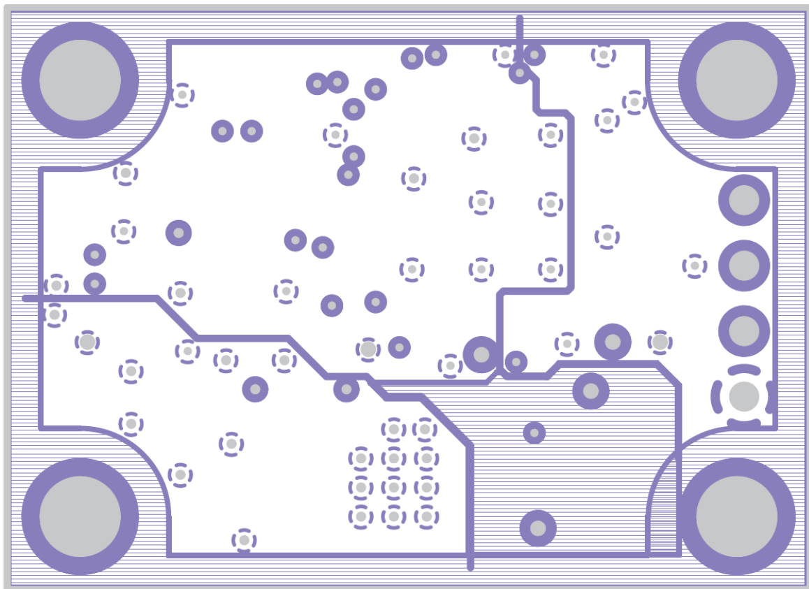
図 2-3 Layer 2
