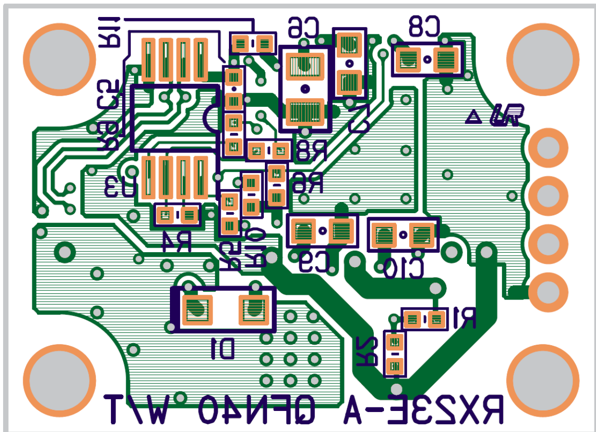
図 2-5 Layer 4
