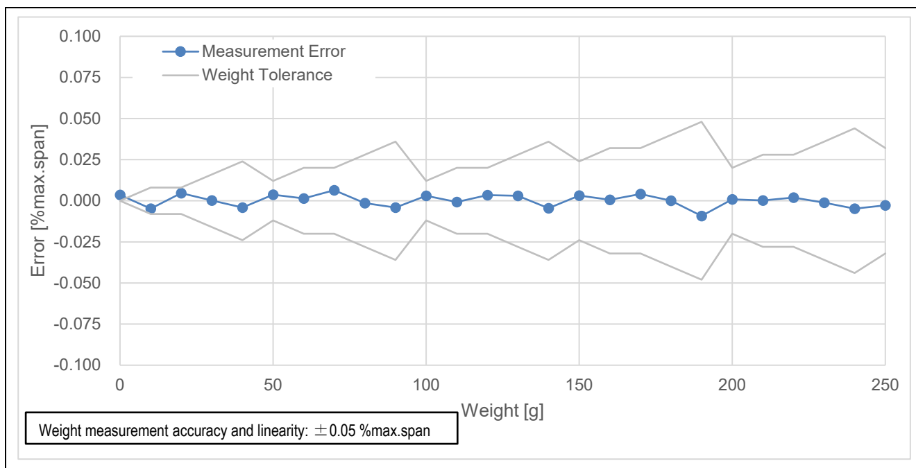
図 3-2 重量計測誤差（周囲温度：25℃）
