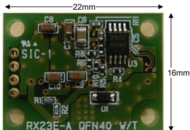
ボード外観
