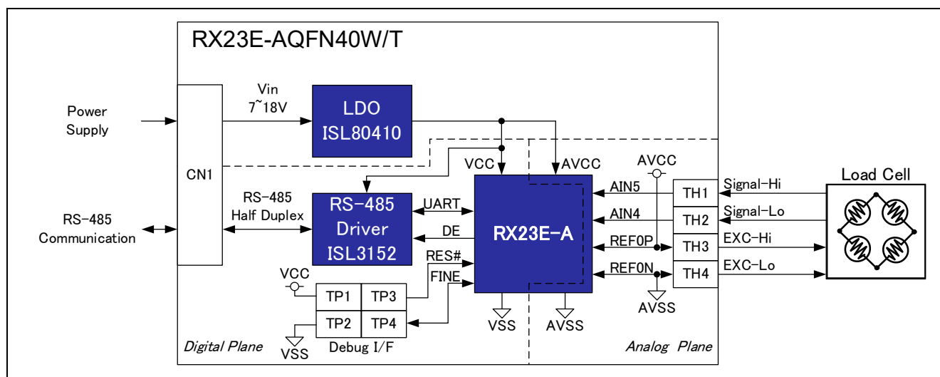
図 1-1 システム構成図
