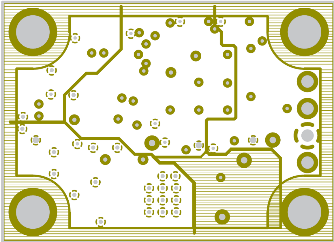
図 2-4 Layer 3
