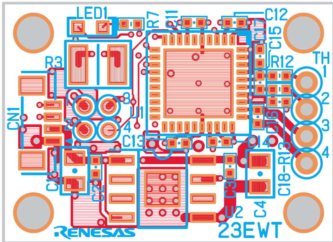
図 2-2 Layer 1
