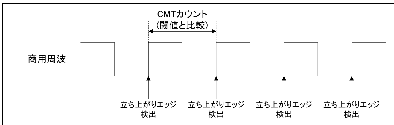
図 1.1 動作概要
