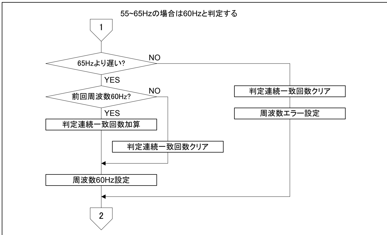
図 5.8 周波数判定 (2/2)
