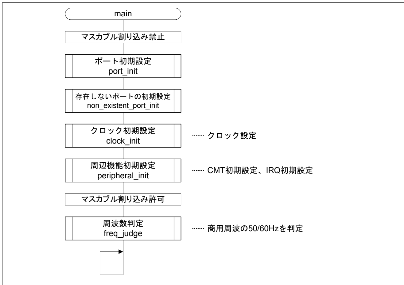
図 5.2 メイン処理
