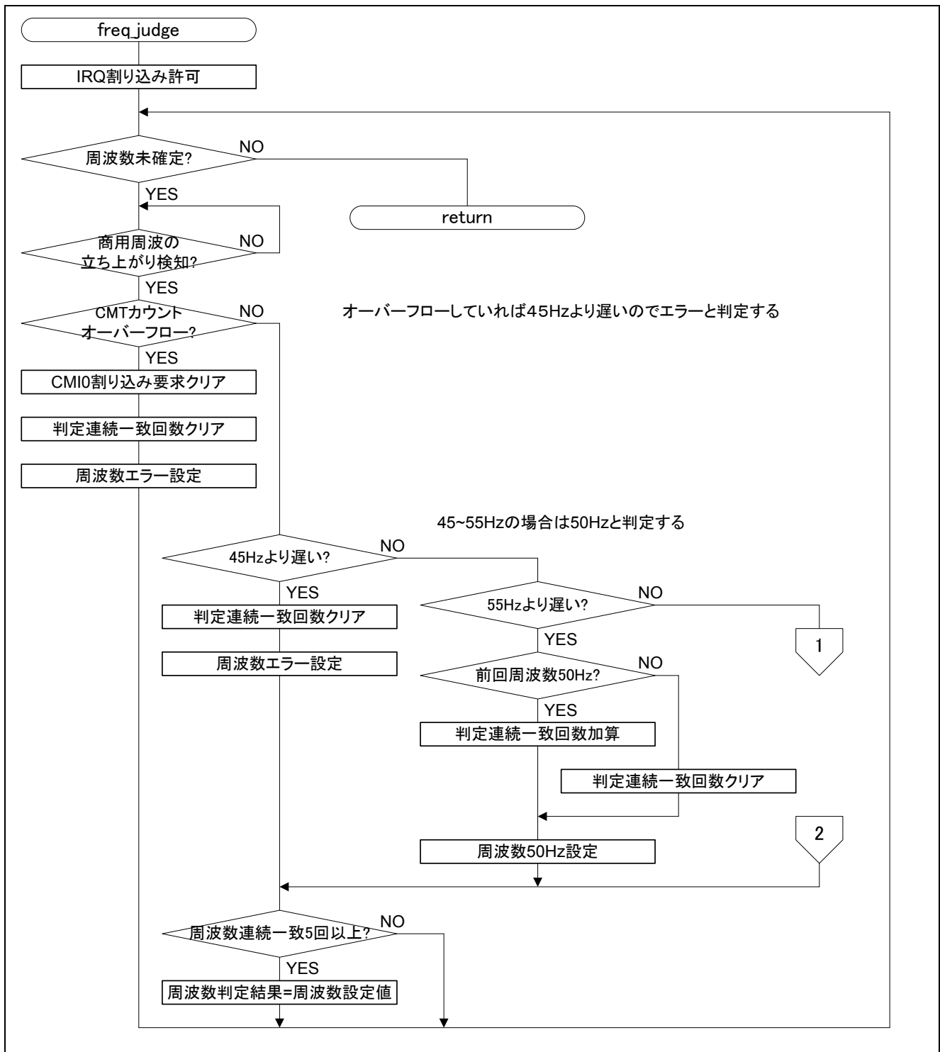
図 5.7 周波数判定 (1/2)
