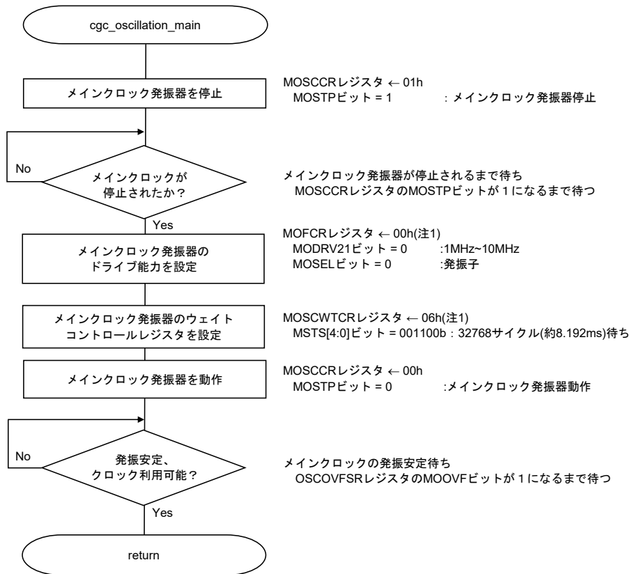
図 3.6 メインクロックの発振設定
