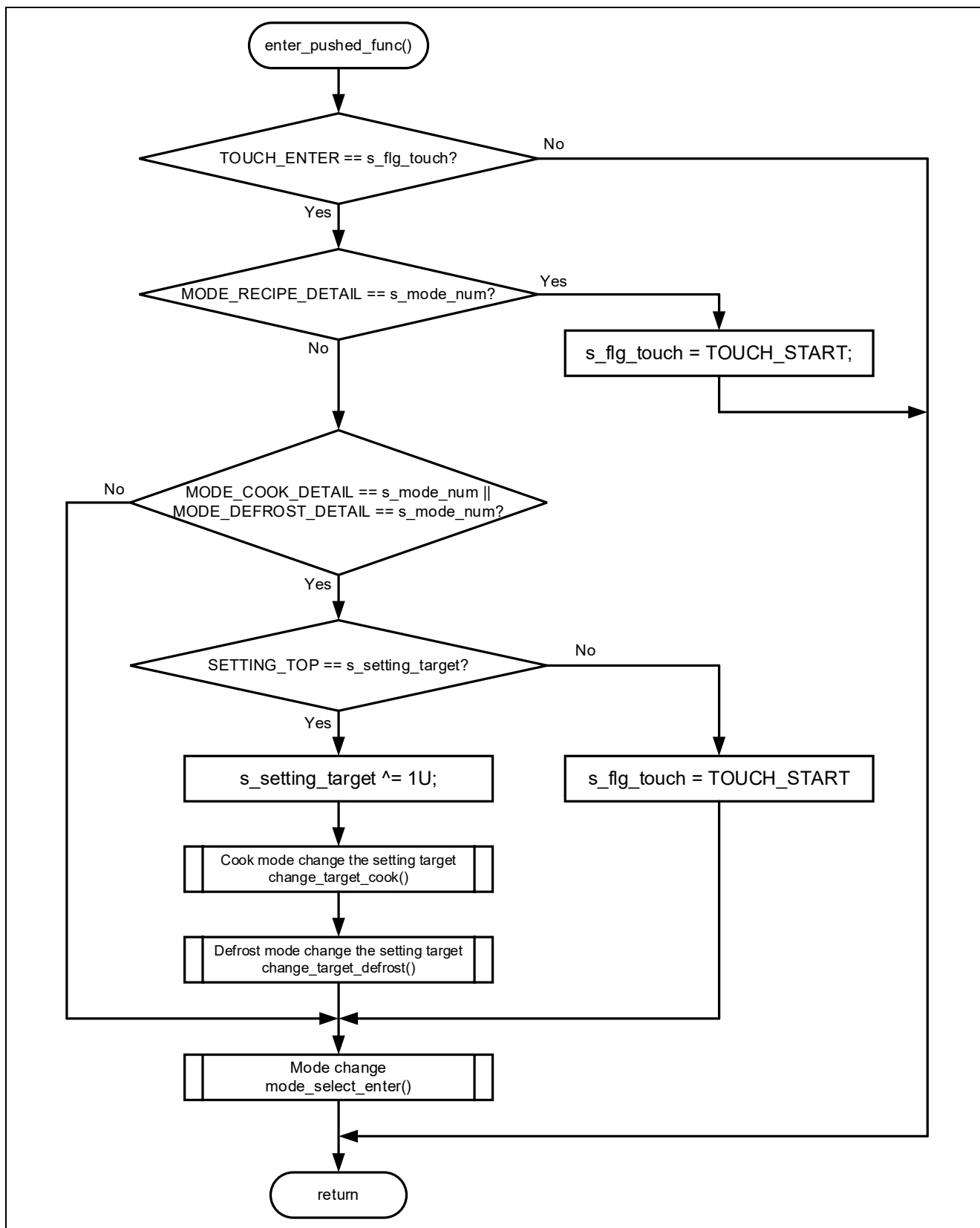
図 4-8 「2」 ボタンタッチ時のフローチャート
