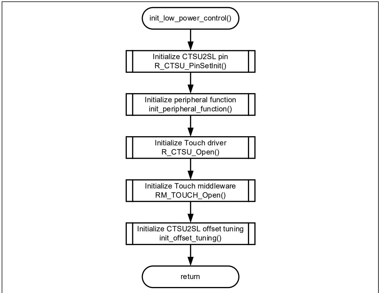
図 4-10 CTSU2SL 初期化のフローチャート
