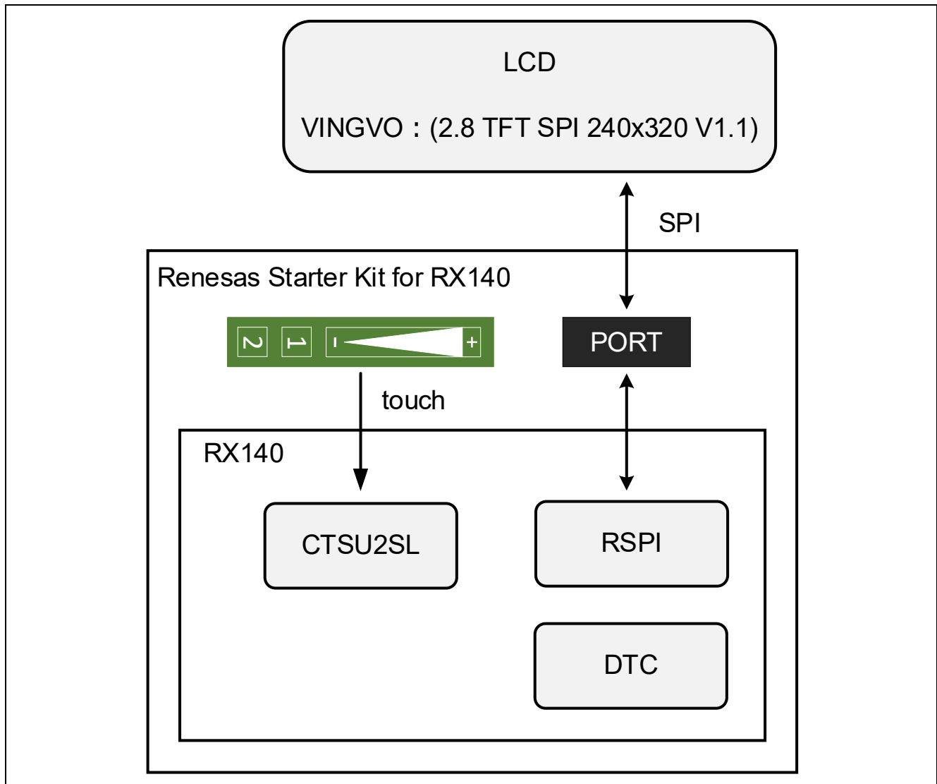
図 1-1 システムの構成
