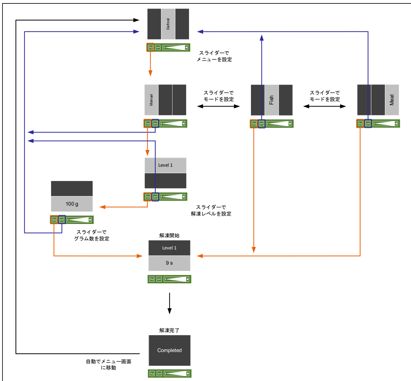
図 4-2 デモ画面のフローチャート (Defrost)
