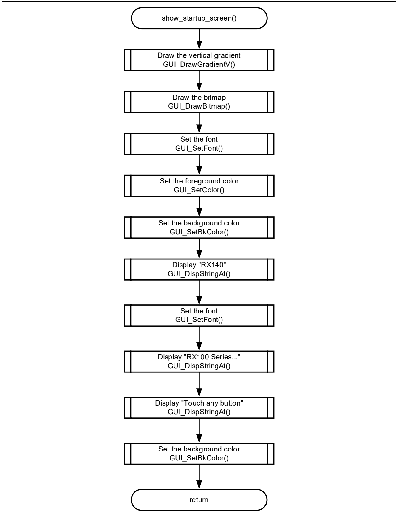
図 4-16 初期画面表示のフローチャート
