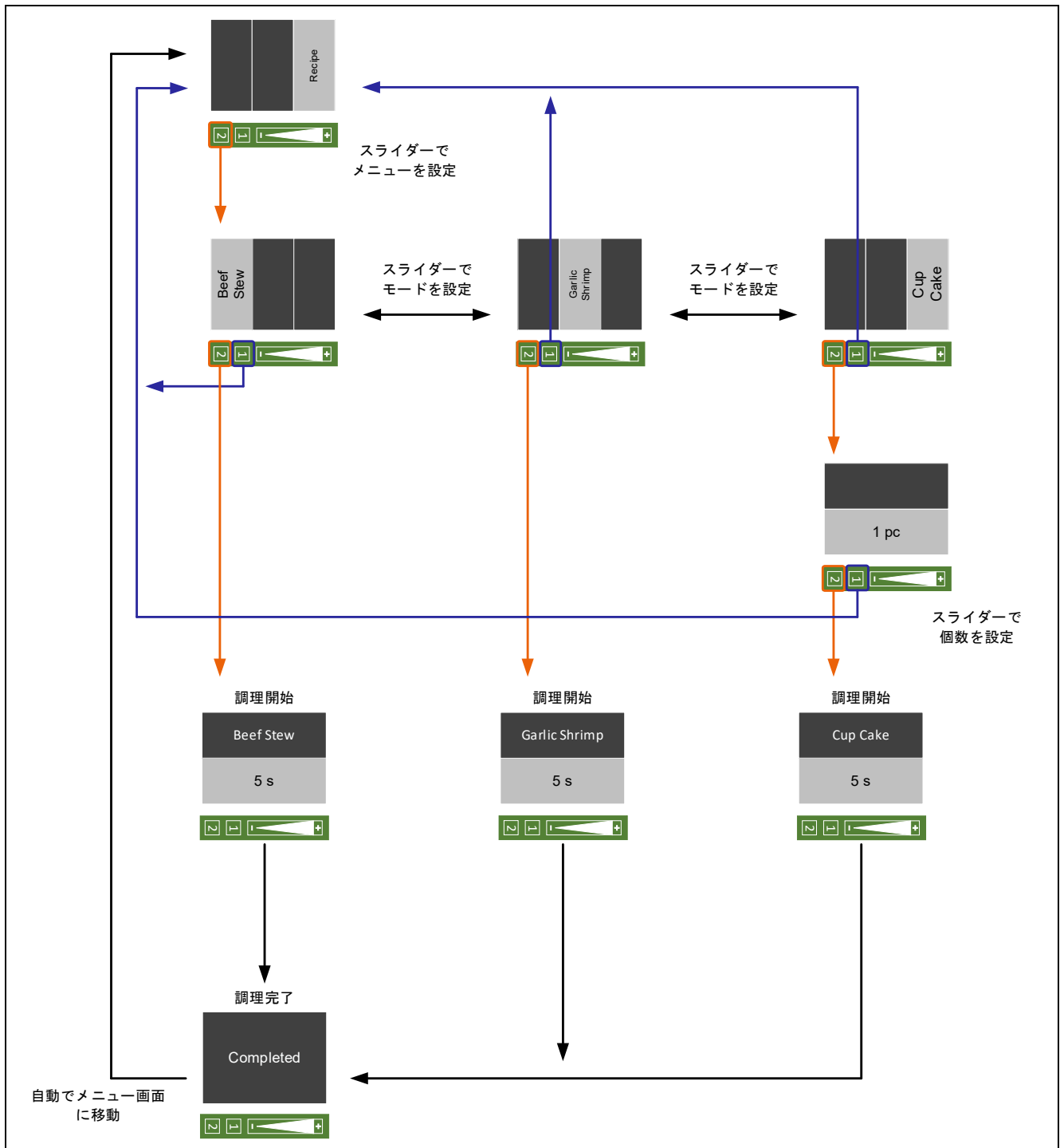
図 4-3 デモ画面のフローチャート (Recipe)
