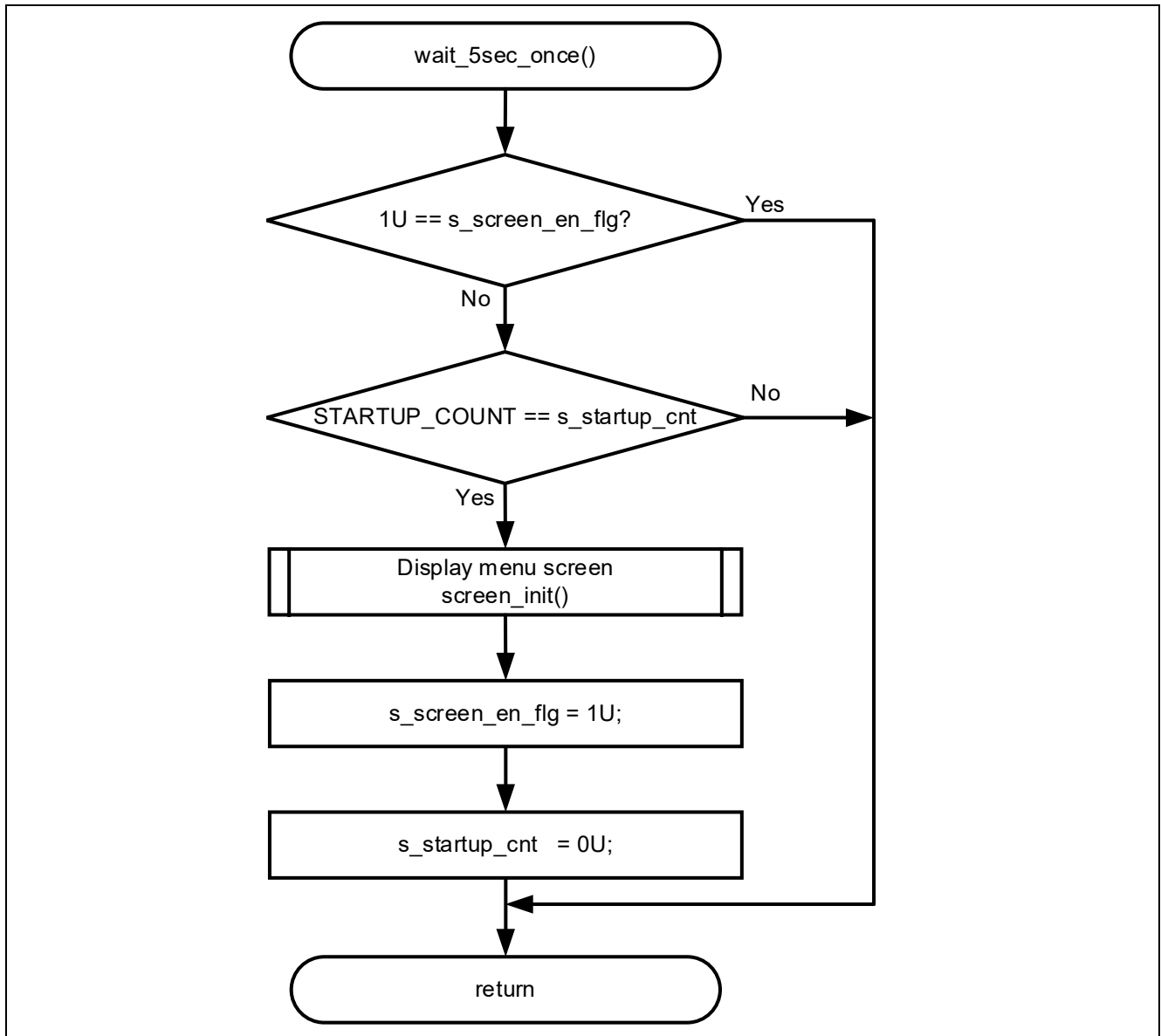
図 4-17 5 秒待機のフローチャート
