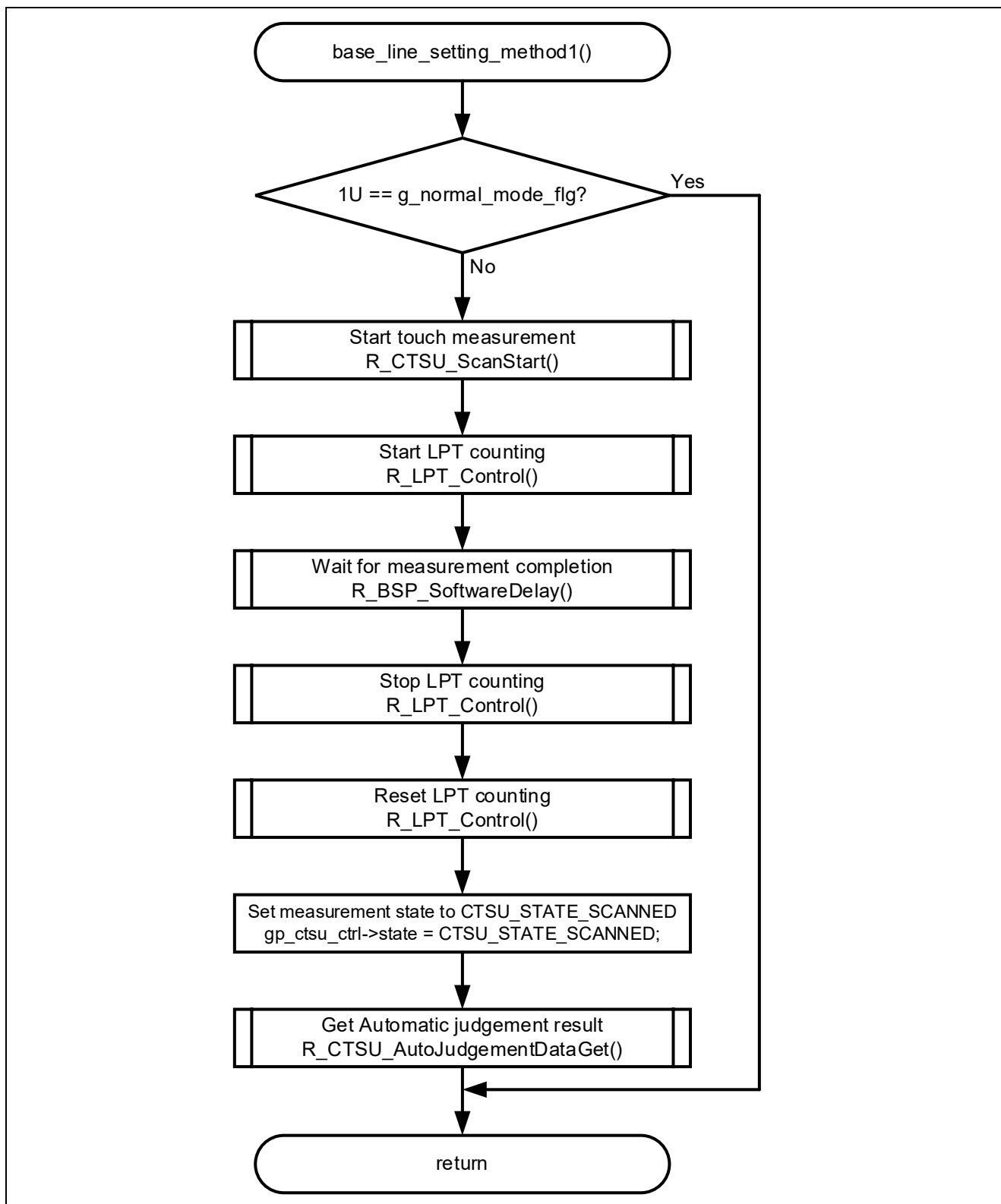
図 4-11 CTSU2SL ベースライン設定のフローチャート
