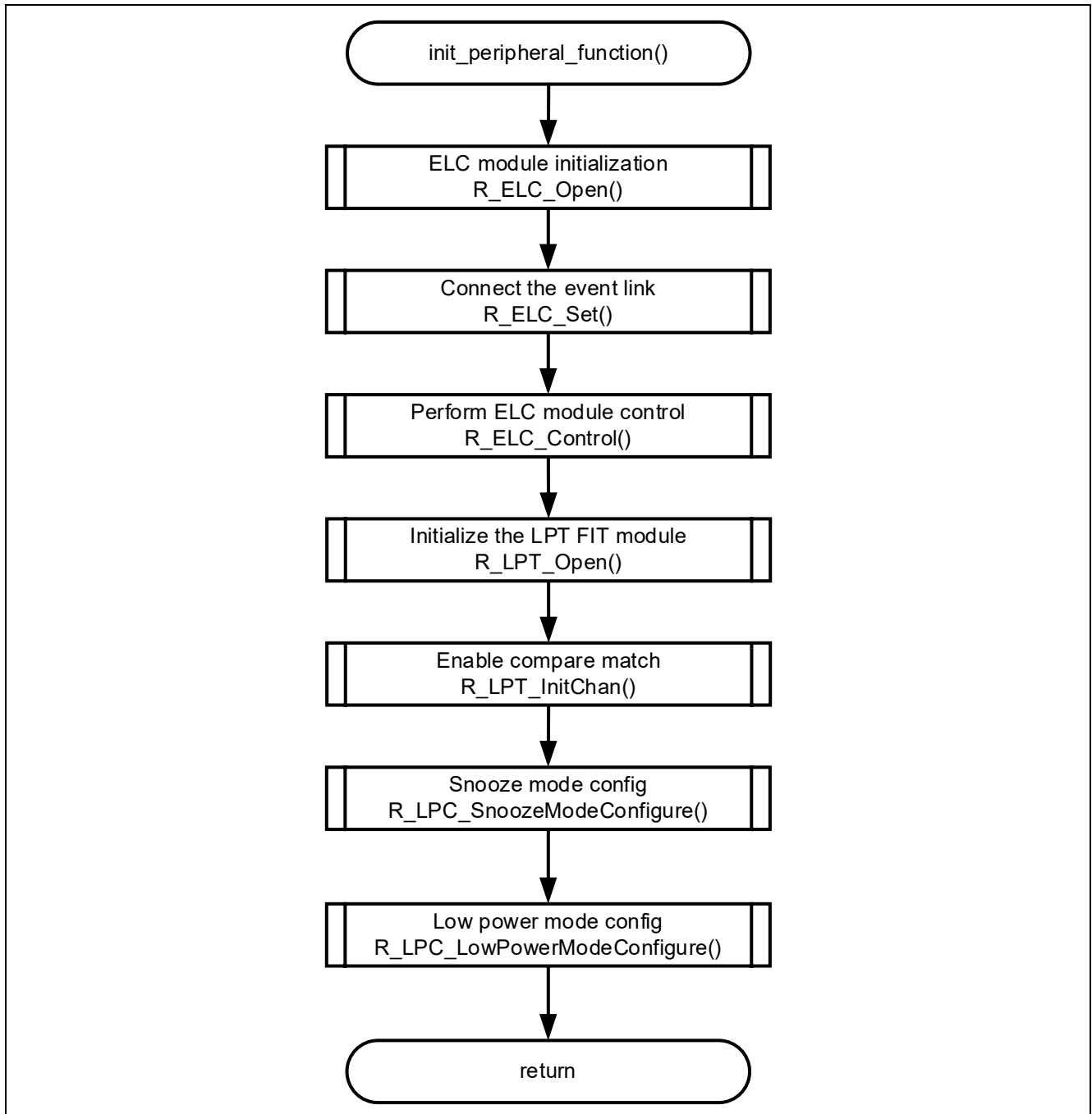
図 4-19 周辺機能初期化のフローチャート
