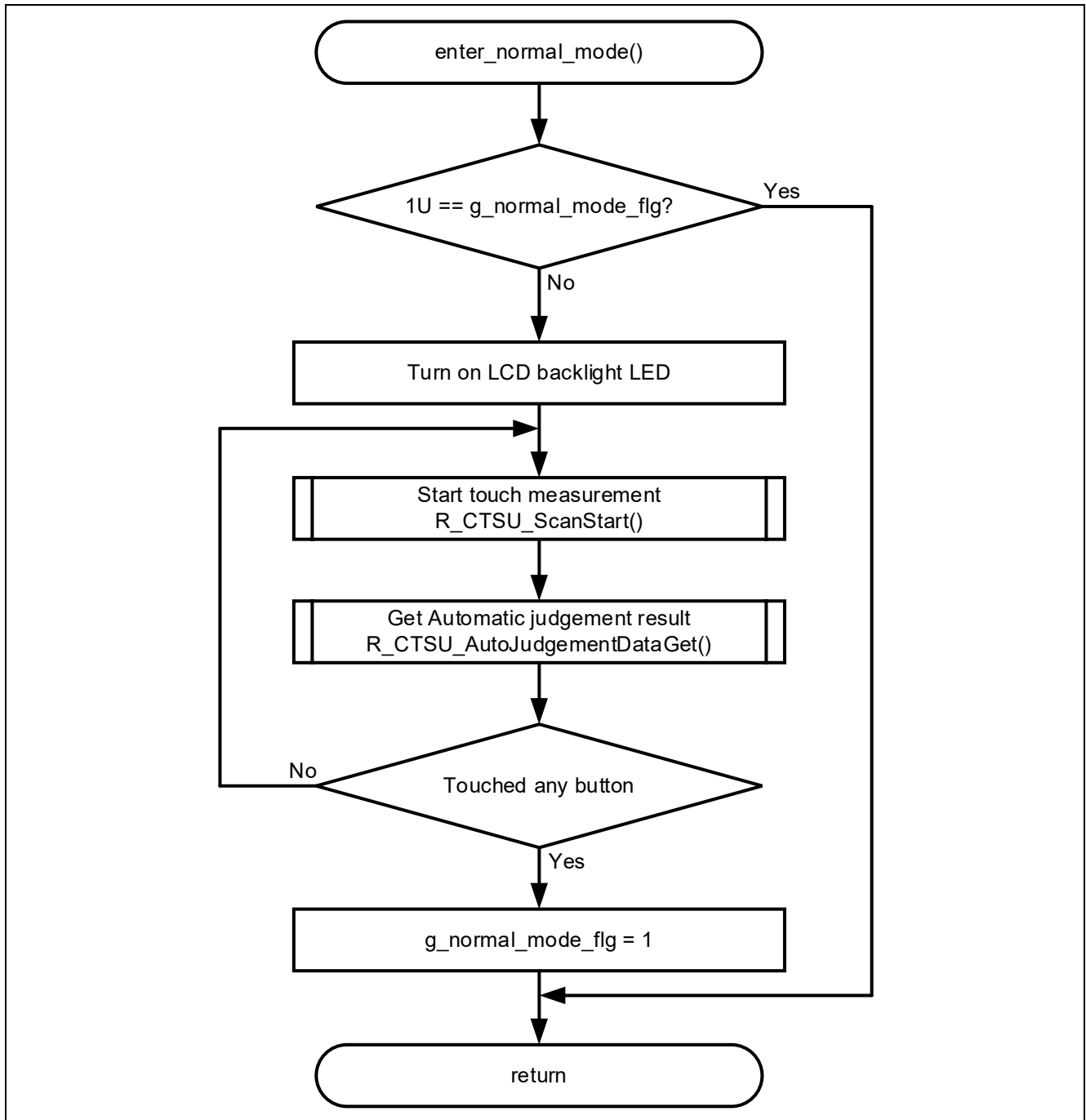
図 4-13 通常動作モード遷移のフローチャート
