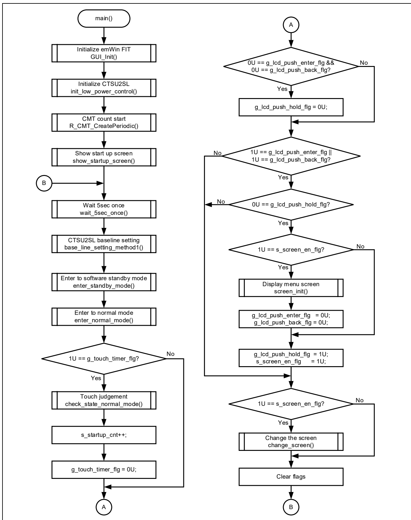
図 4-4 全体フローチャート
