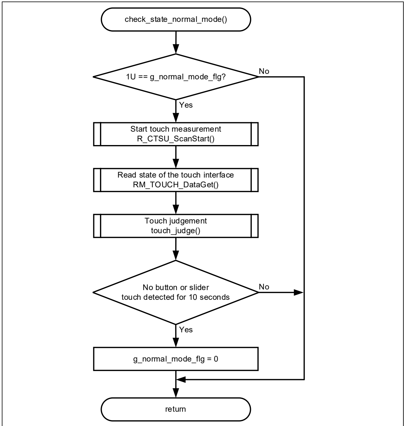
図 4-14 CTSU2SL 通常計測のフローチャート
