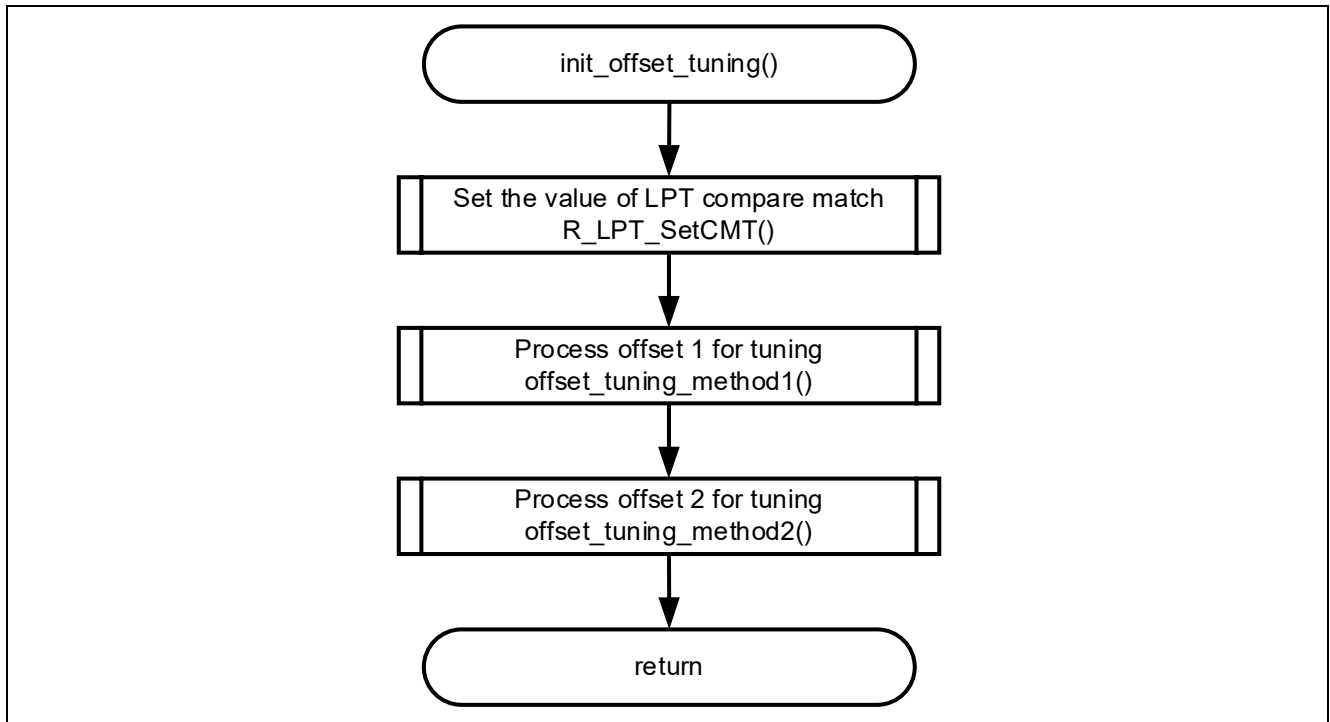
図 4-20 チューニング用オフセットの初期化フローチャート
