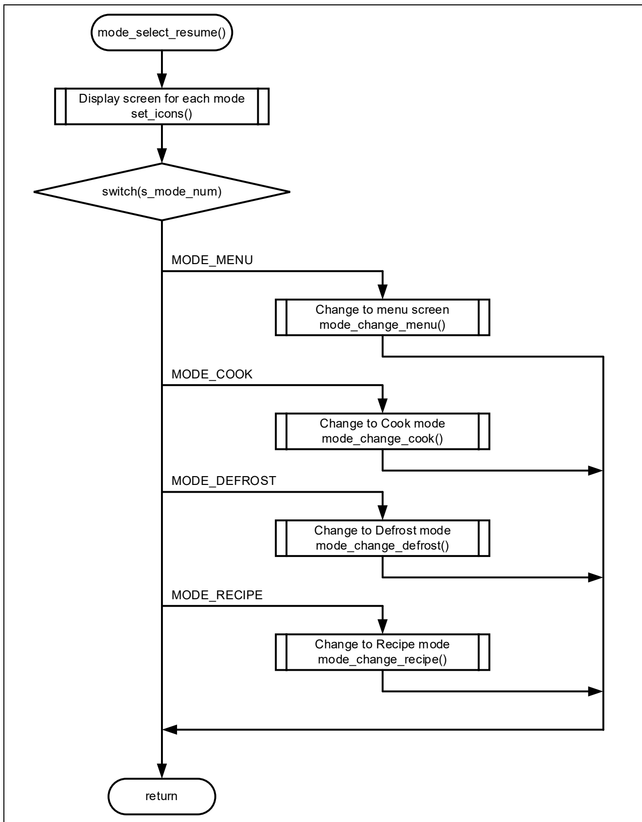
図 4-21 メニュー表示再開のフローチャート
