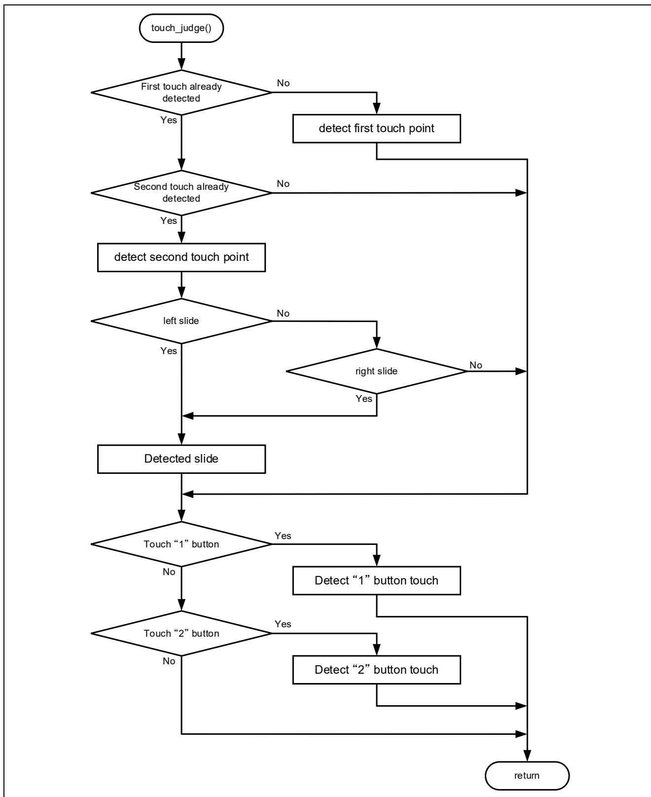
図 4-15 タッチ判定のフローチャート
