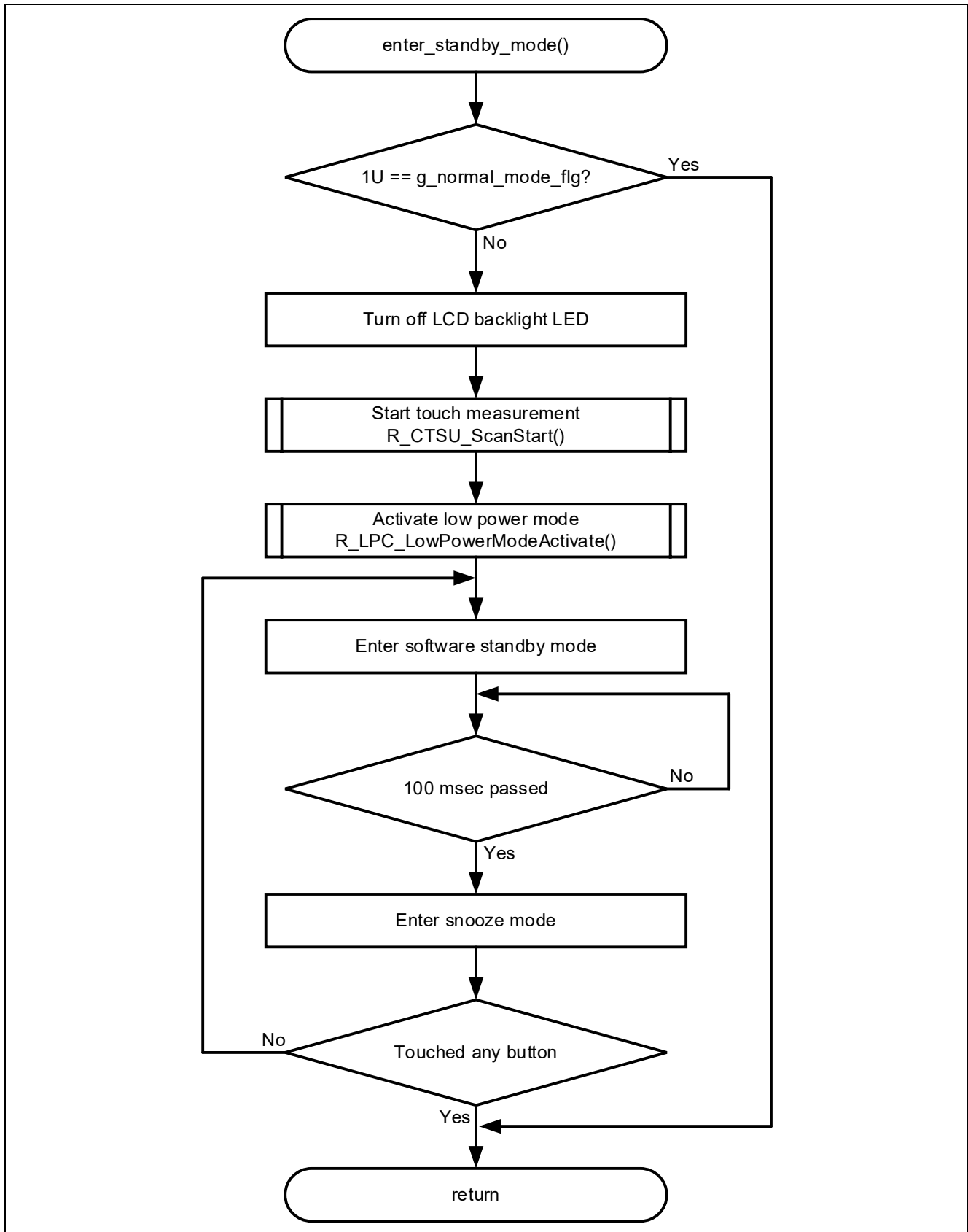
図 4-12 ソフトウェアスタンバイモード遷移と低消費電力計測のフローチャート
