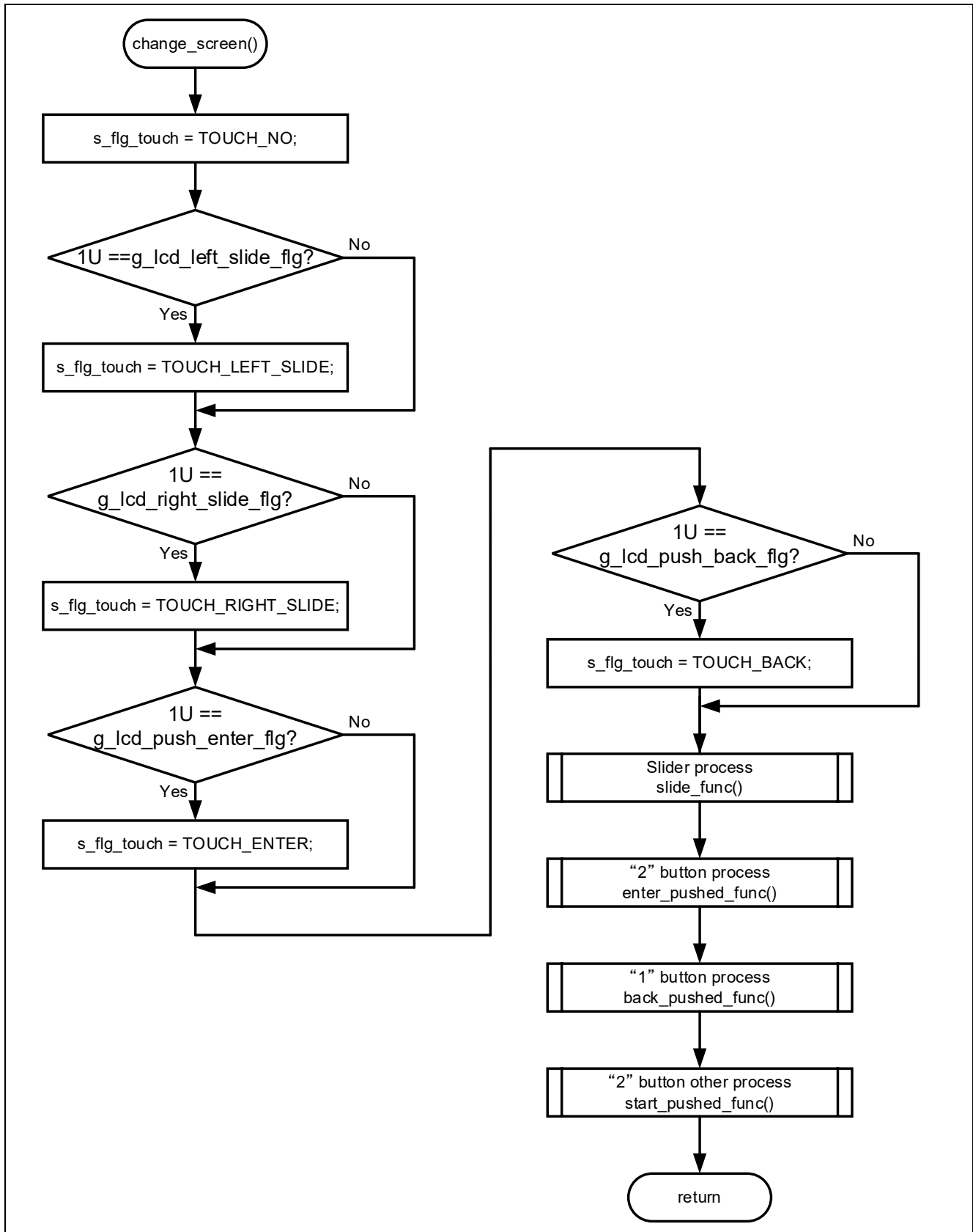
図 4-5 タッチ操作時の処理のフローチャート
