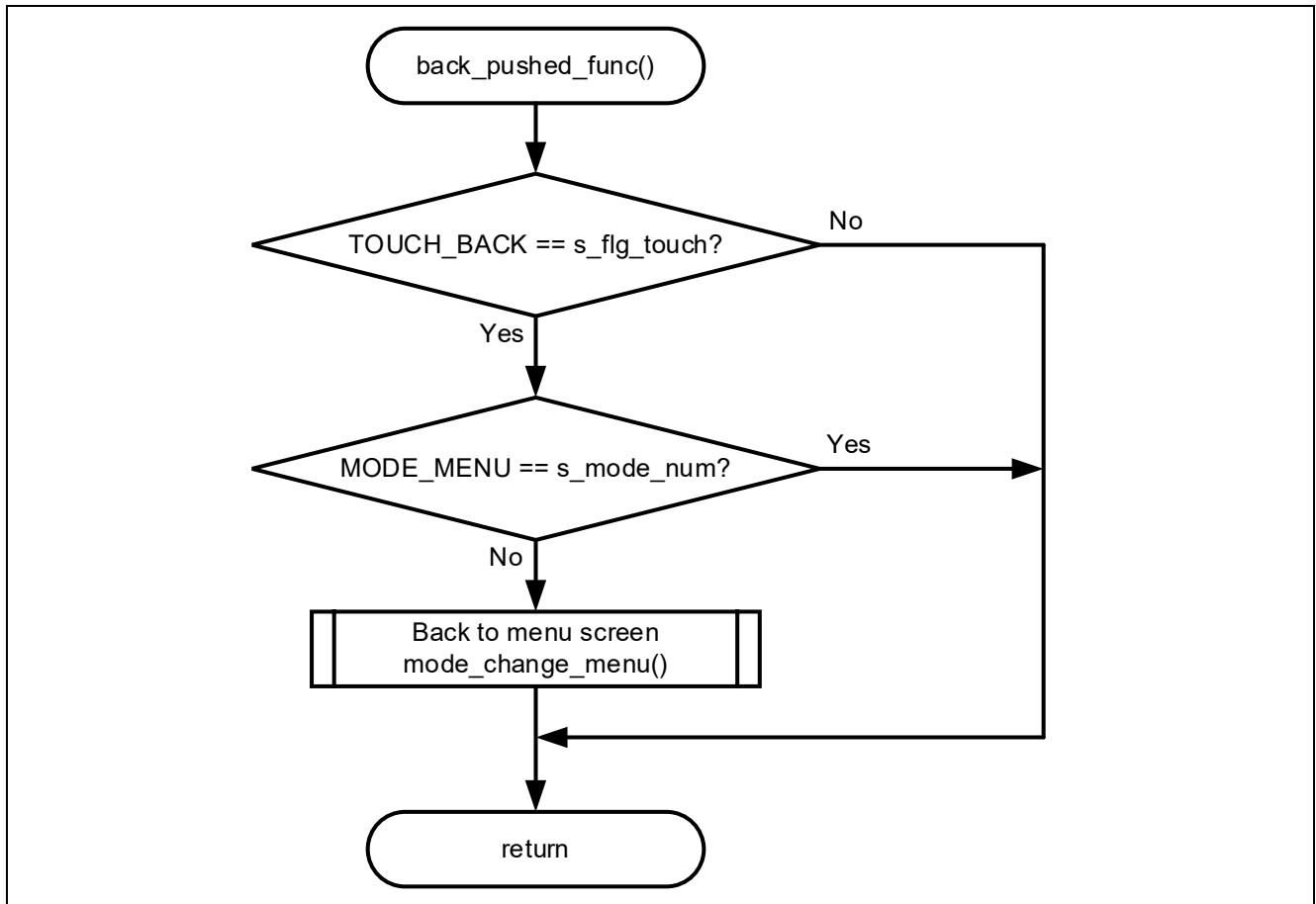
図 4-7 「1」 ボタンタッチ時のフローチャート
