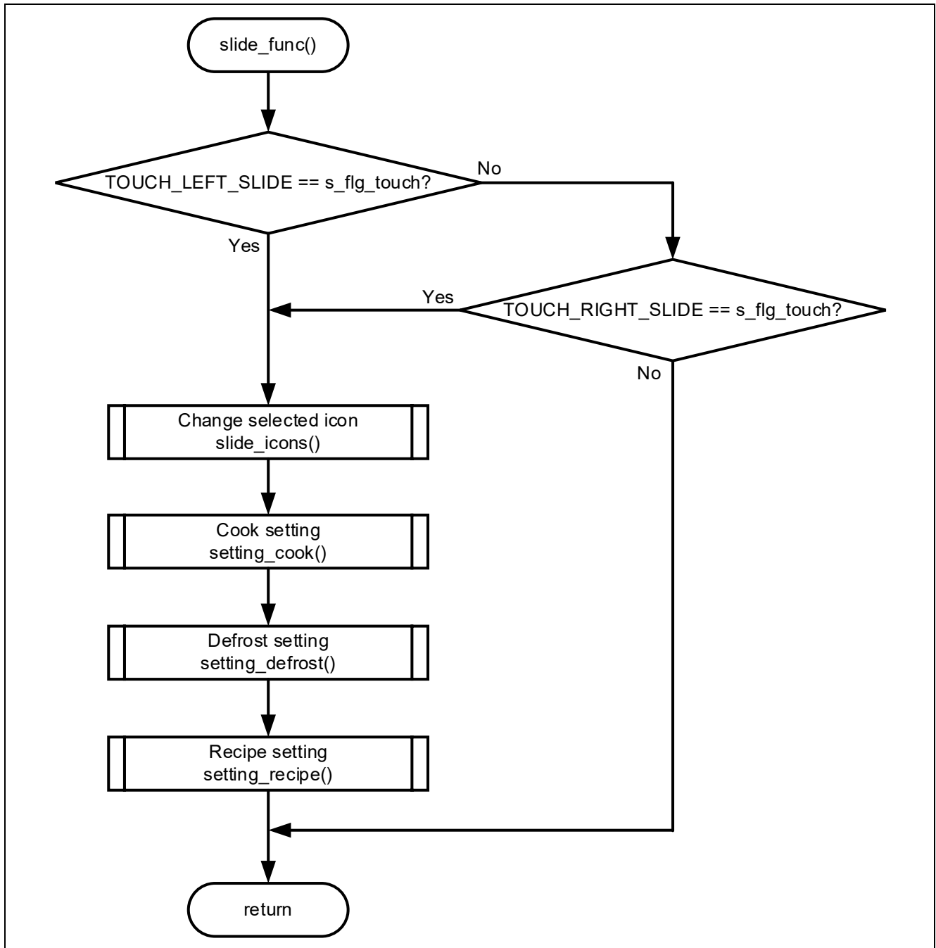
図 4-6 タッチスライダ操作時のフローチャート
