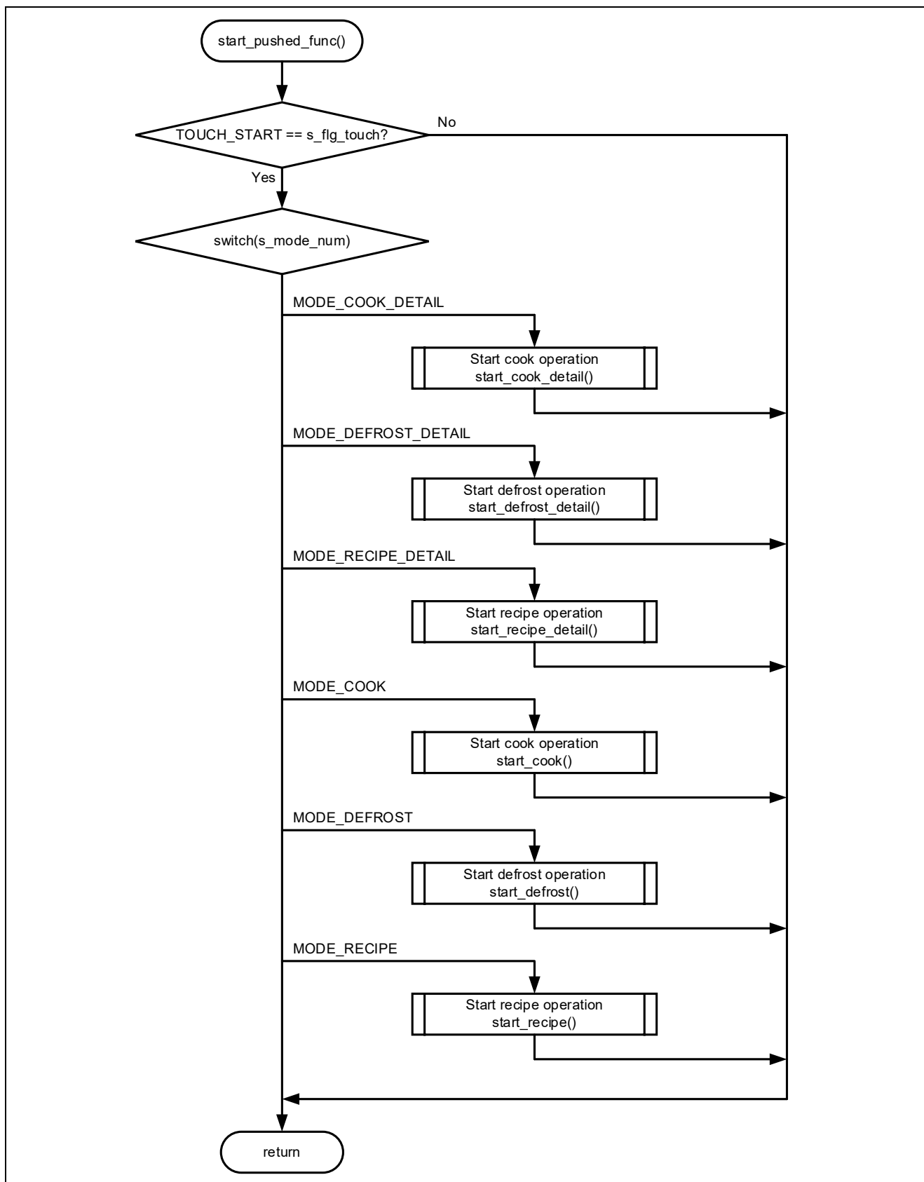
図 4-9 「2」 ボタンタッチ時のフローチャート
