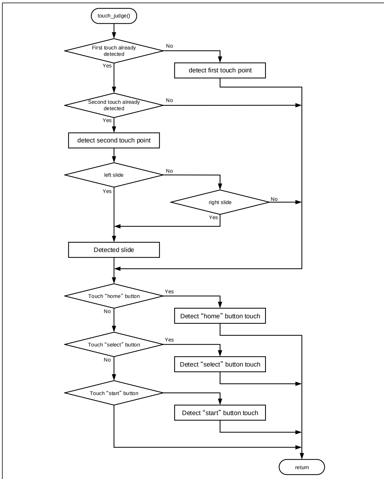
図 3-15 タッチ判定のフローチャート
