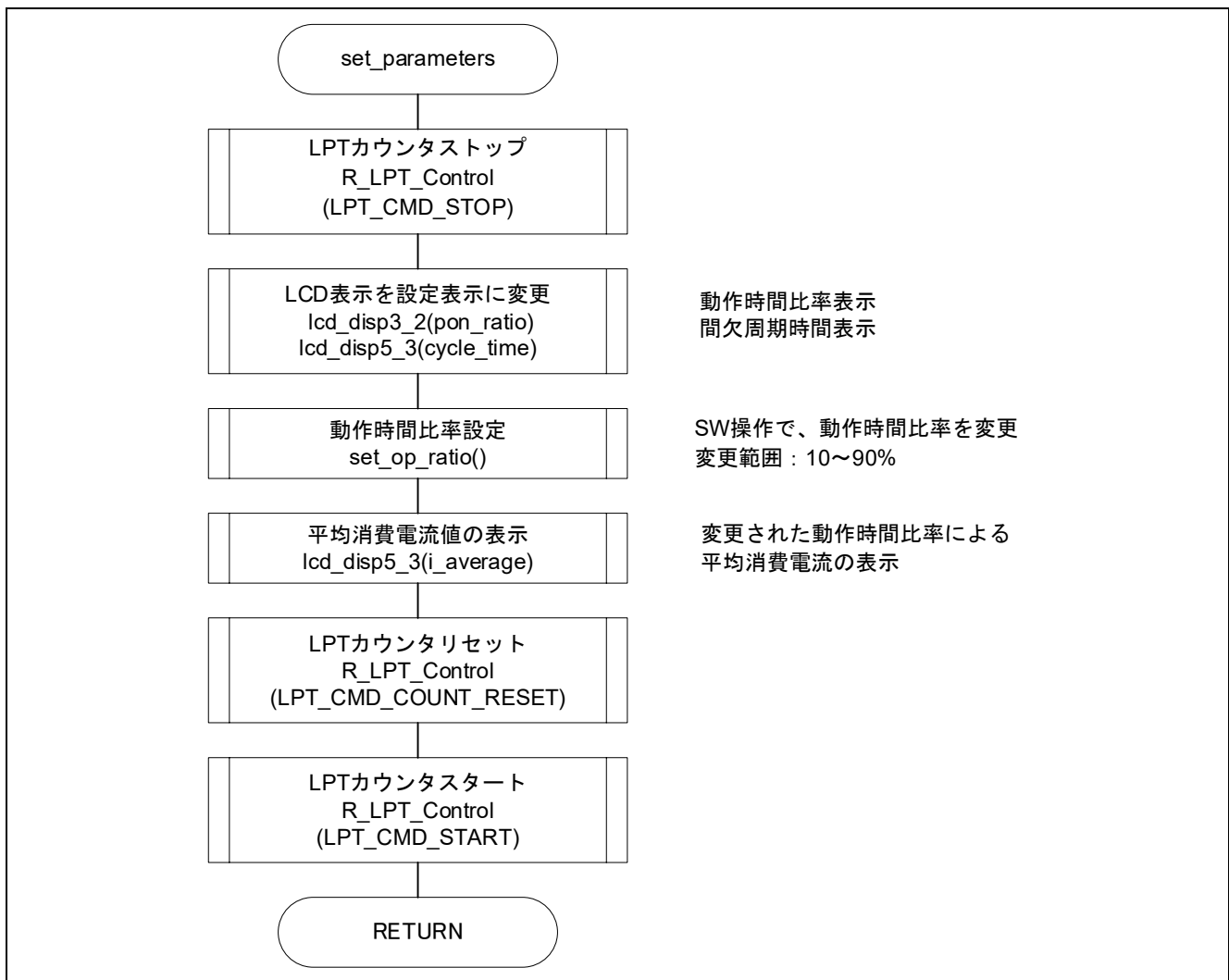
図 4.4 間欠動作設定関数
