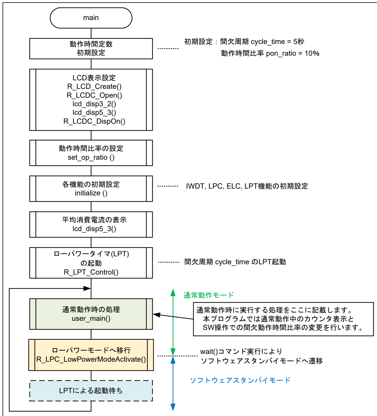
図 4.1 main 関数
