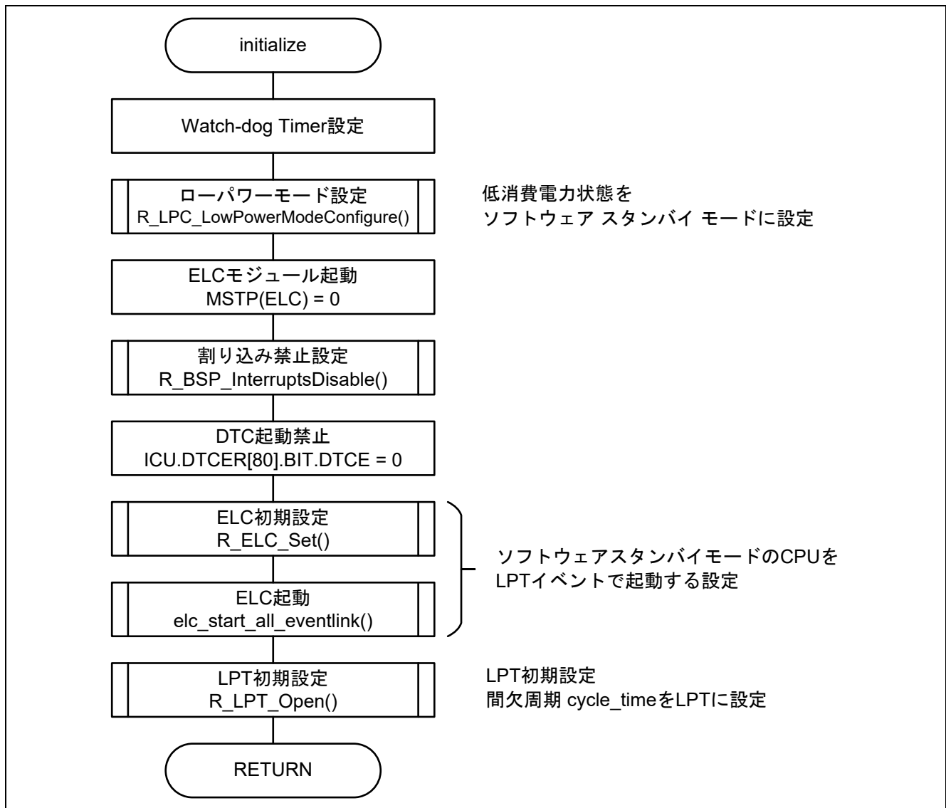
図 4.2 initialize 関数
