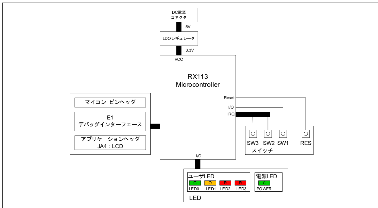
図 2.2 ボード内接続
