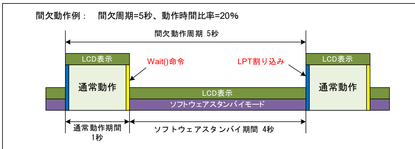
図 1.2 間欠動作例
