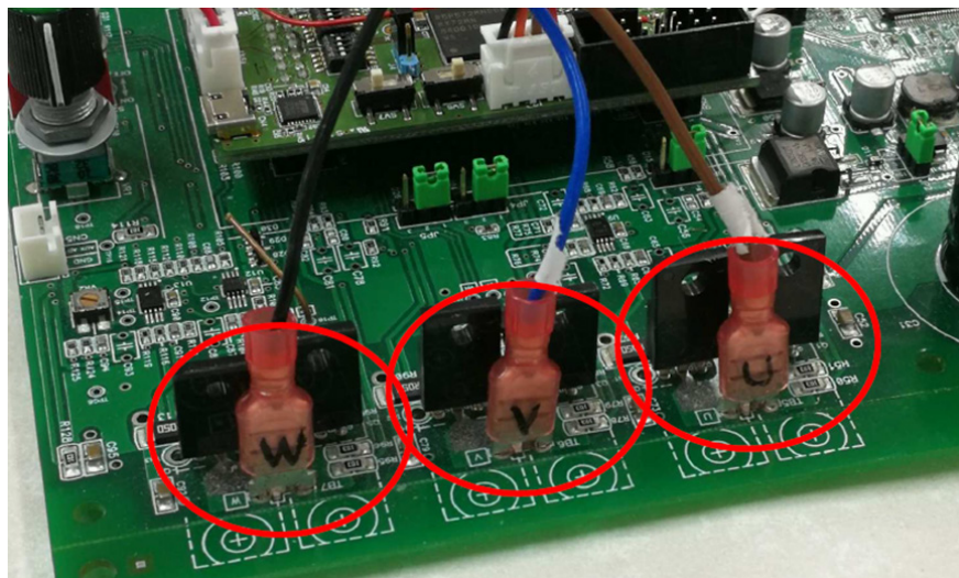
図 6-1 三相電源線の接続
