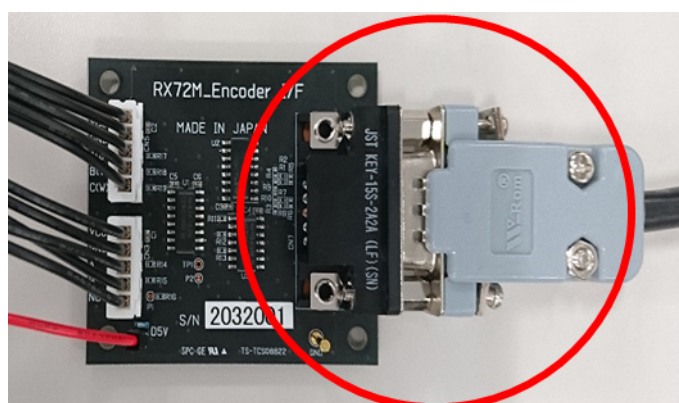
図 6-2 エンコーダー I/F 基板の接続
