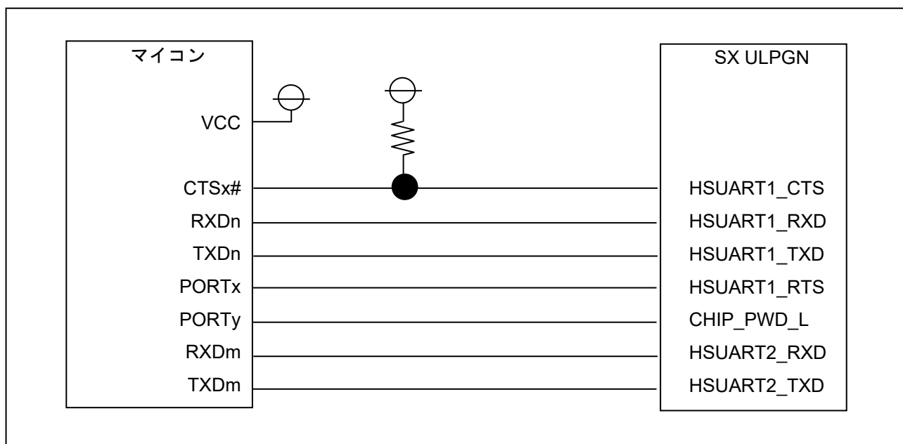
図 1.2 2CH 通信モード時の接続例
