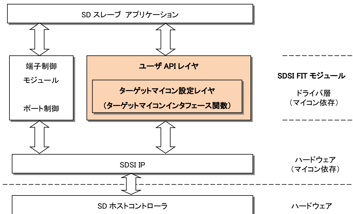
図 1-3 ソフトウェア構成
