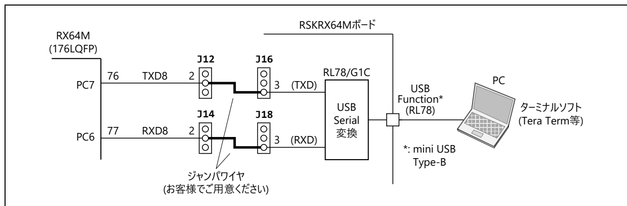
図 5.1 RSKRX64M ボードのジャンパ設定（概略図）
