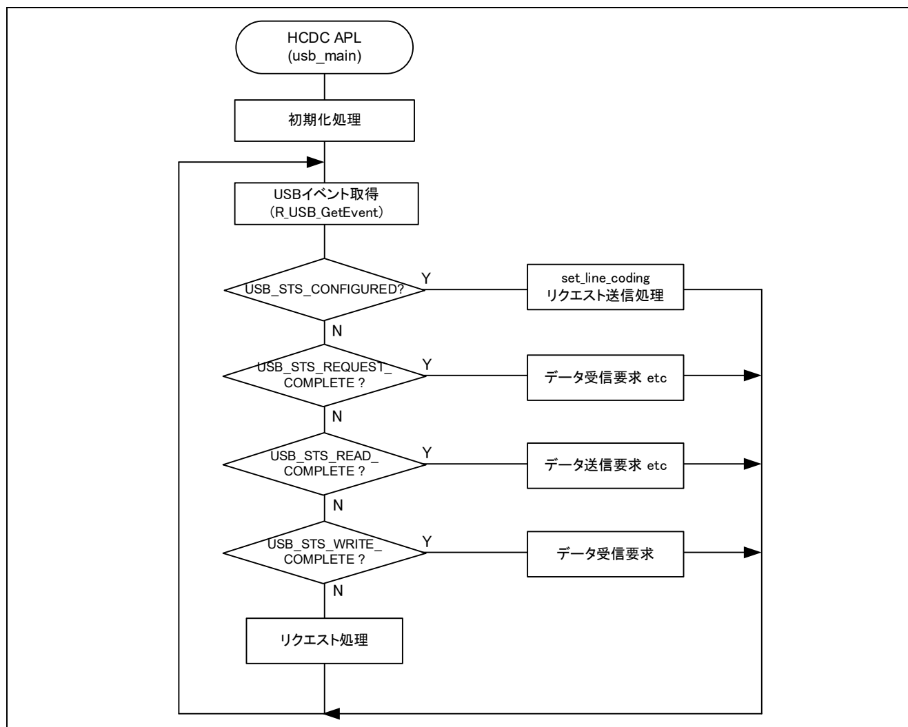
Figure 4-2 メインループ処理 (Non-OS)
