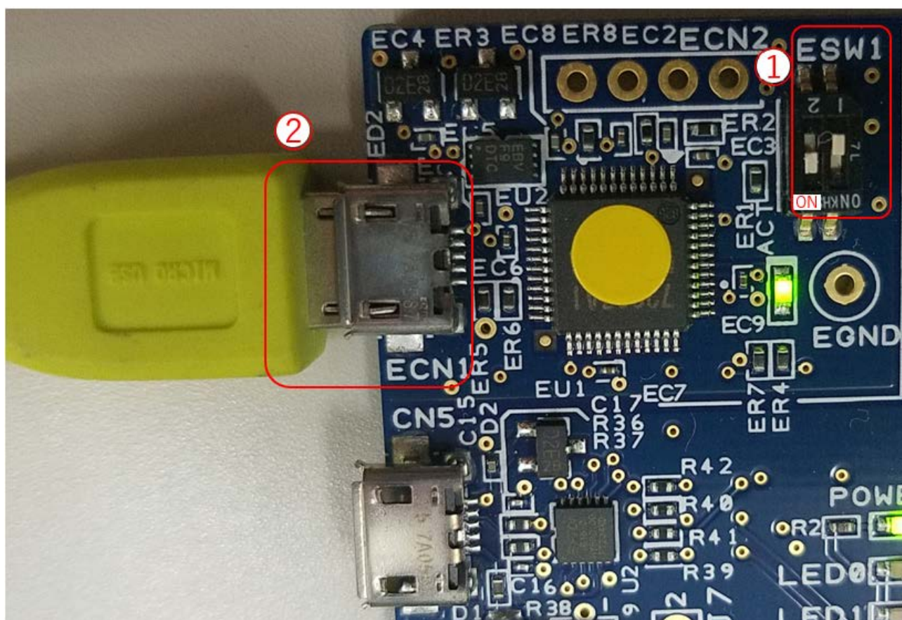
図 4-1 通信先 Target Board for RX23W の接続
