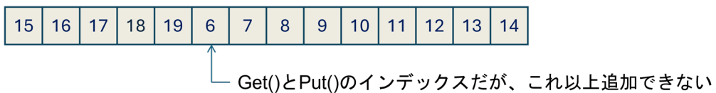
図 1-4 オーバーフィルを試行する際のキューの状態
