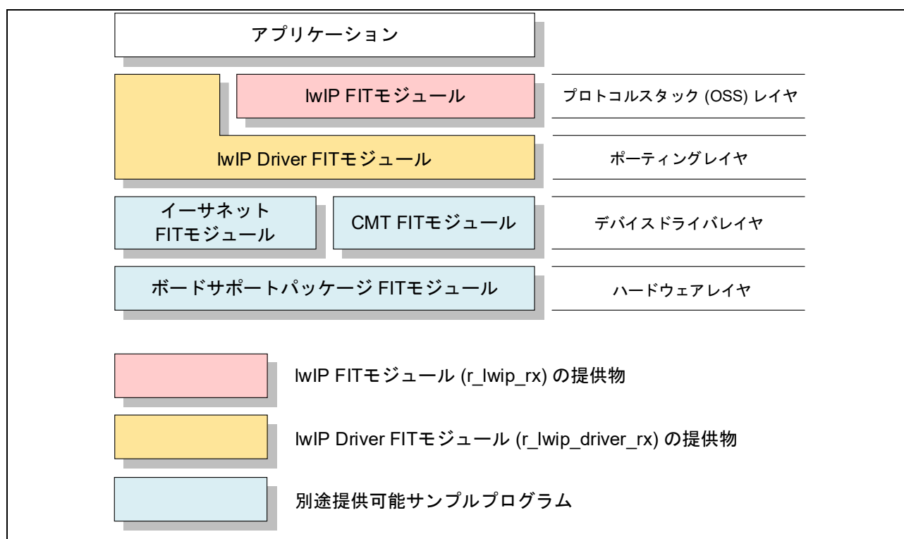
図 1 ソフトウェア構成図
