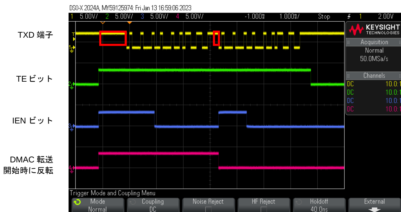
図 3.11 サンプルプログラムの波形
