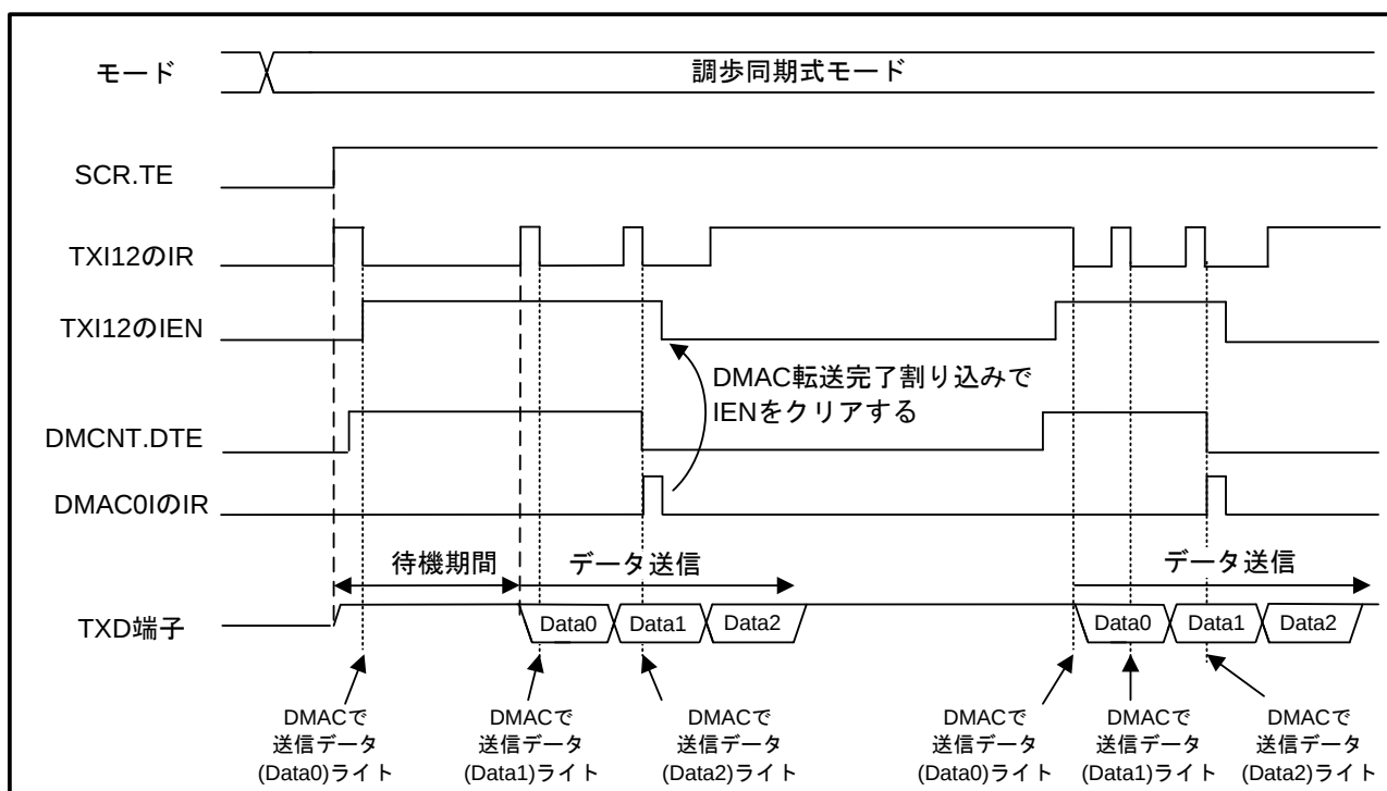
図 3.7 修正後のタイミング図（DMAC 転送にて送信データを書き込む場合）
