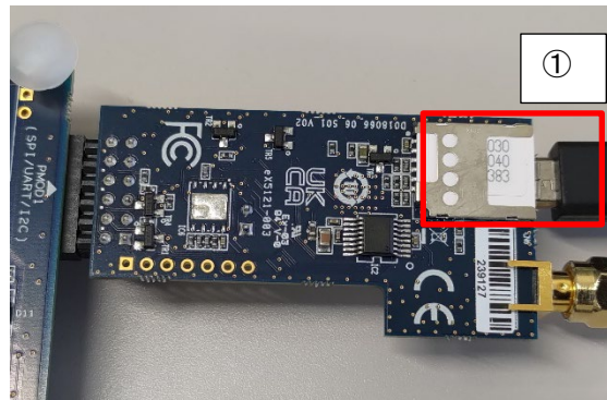
図 2-1 RYZ014A PMOD 裏面
