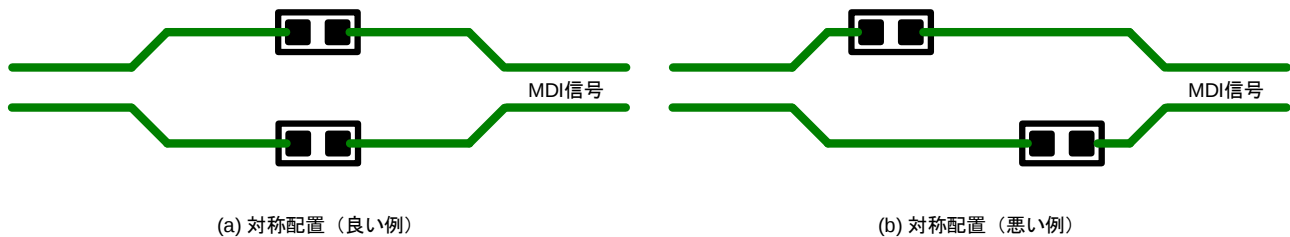
図 7 差動信号伝送路上の部品配置
