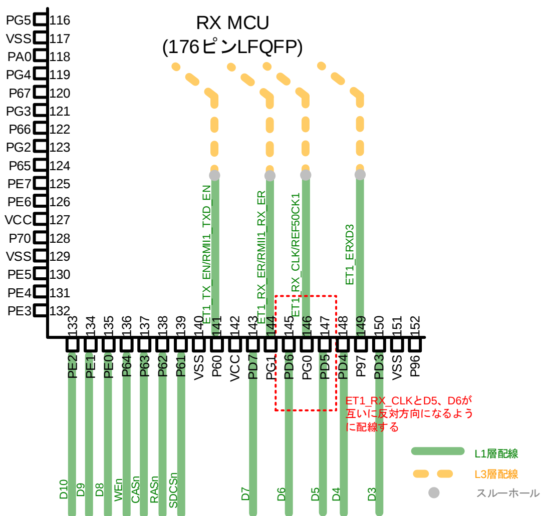
図5 配線例
