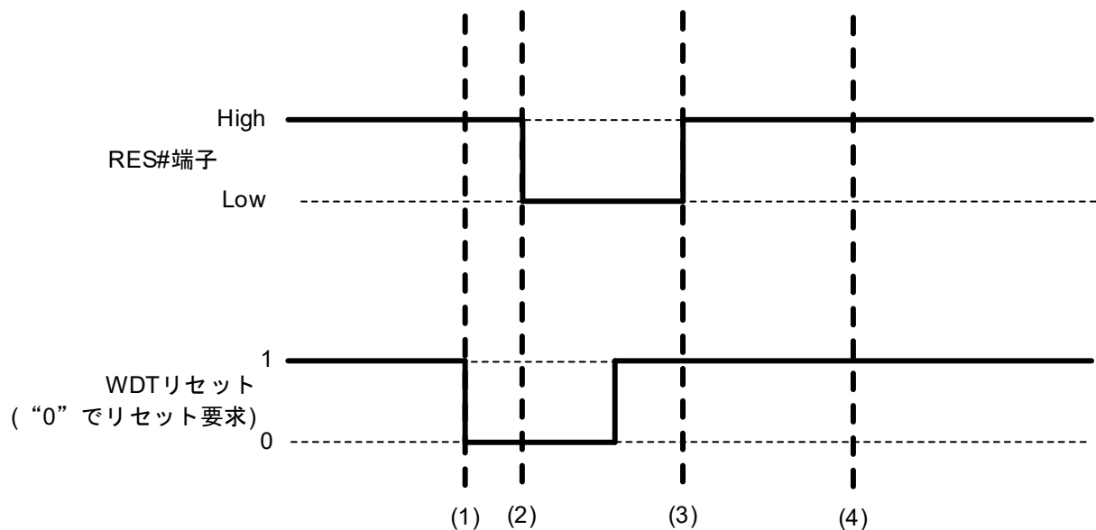
図 3.13 ウォッチドックタイマリセットと RES#端子リセットが発生した場合の例
