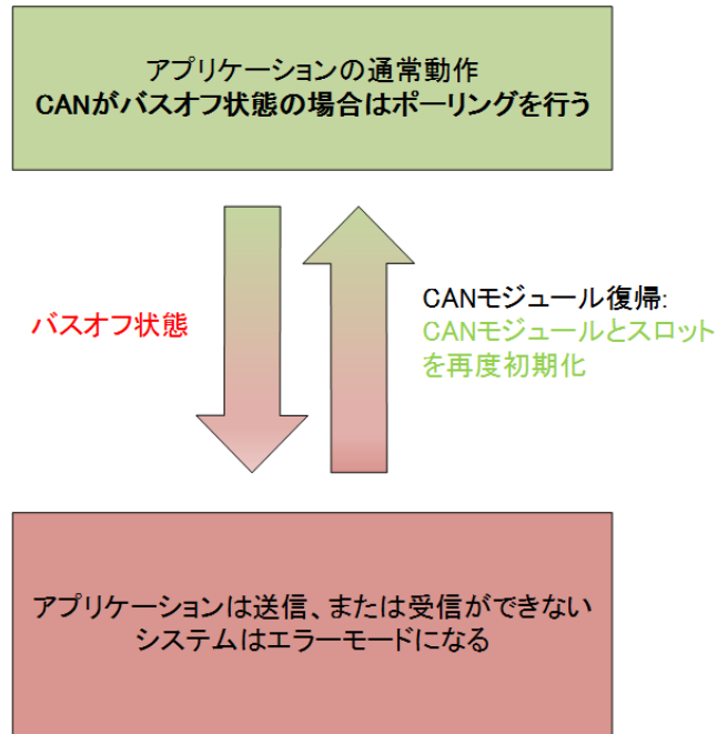
図 4 アプリケーションのバスオフ復帰の対応（バスオフ復帰はMCUで検出）
