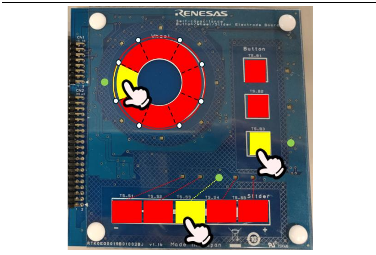
図 5.11 タッチボタン電極の動作範囲例
