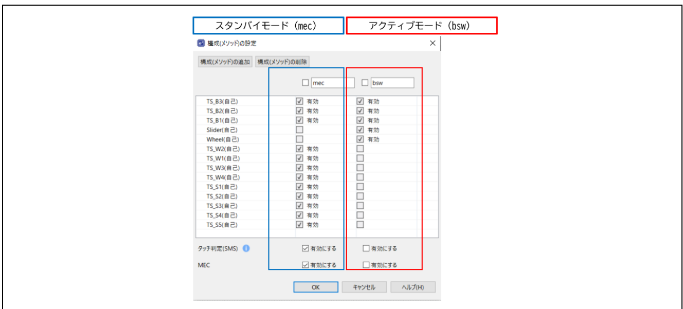
図 4.2 構成(メソッド)の設定画面
