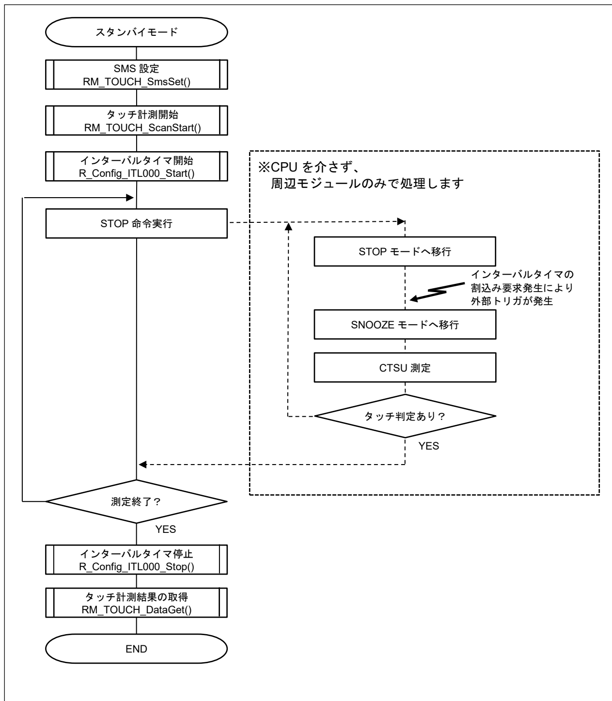
図 5.9 スタンバイのフローチャート
