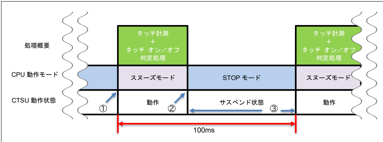
図 5.8 CPU 動作モードと CTSU 動作状態のイメージ
