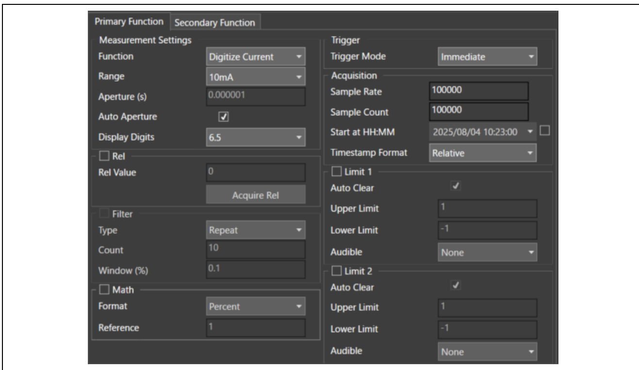
図 7.4 KEITHLEY/KickStart ・消費電流計測設定
