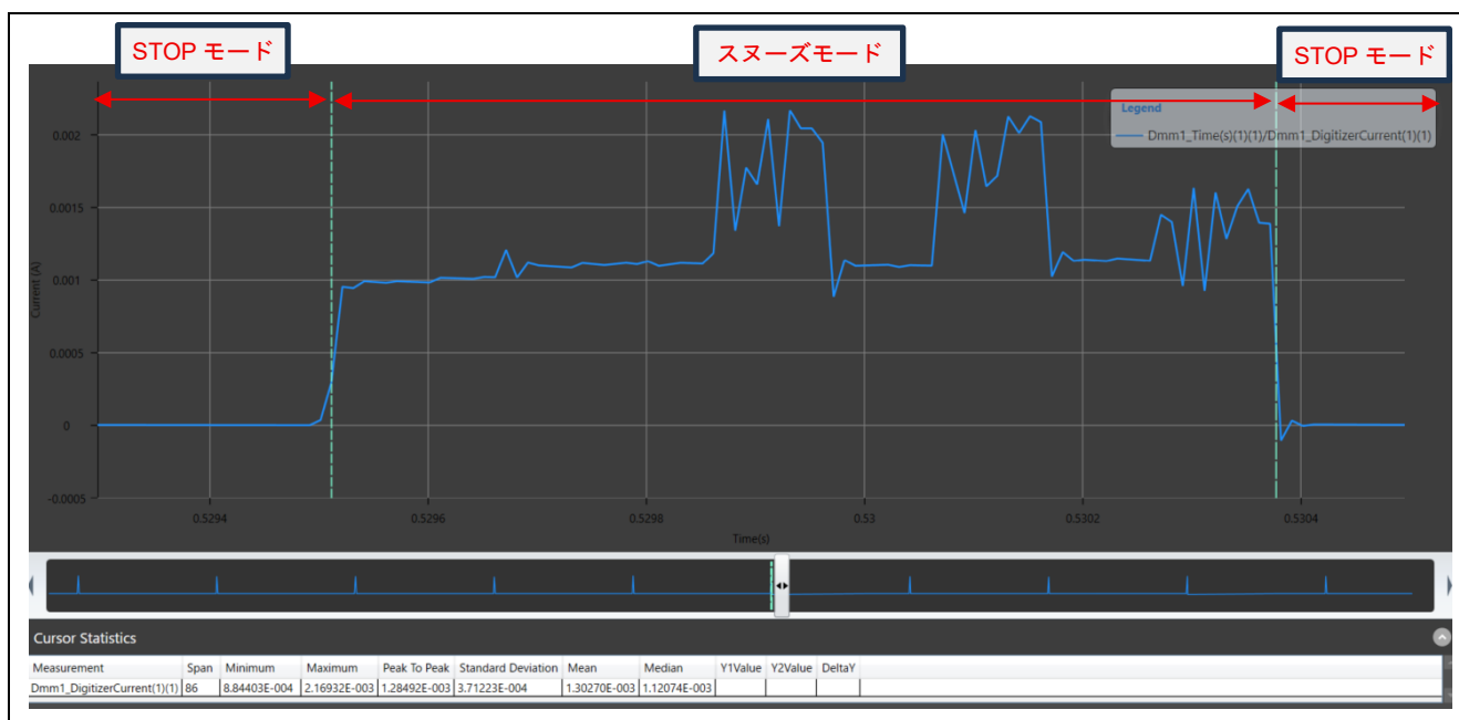
図 7.6 スタンバイモードの消費電流波形 (2/2)
