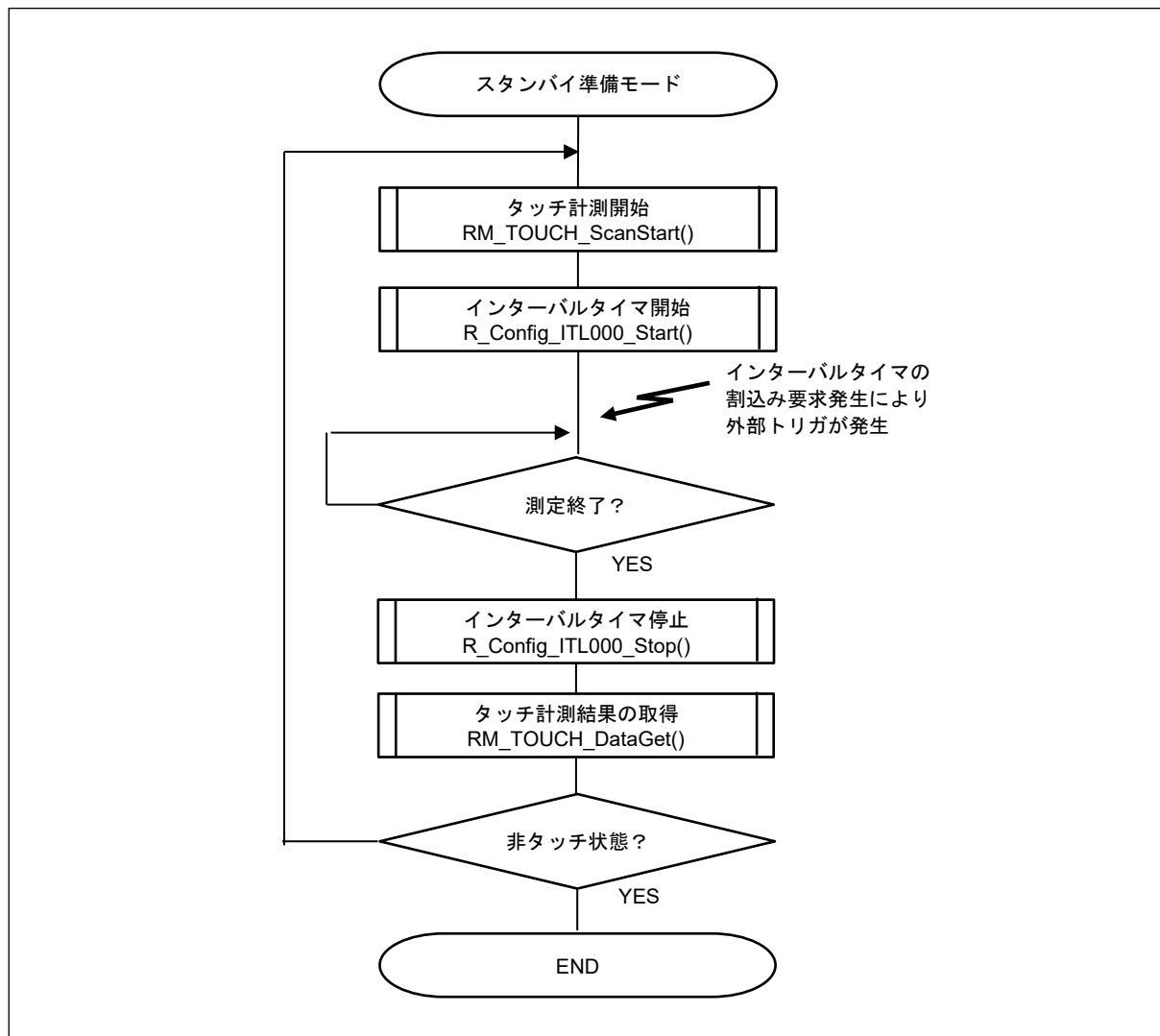
図 5.6 スタンバイ準備のフローチャート
