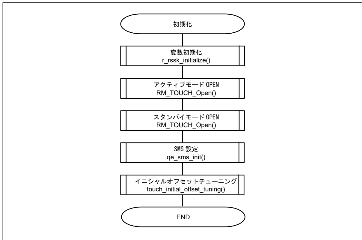
図 5.5 初期設定処理のフローチャート
