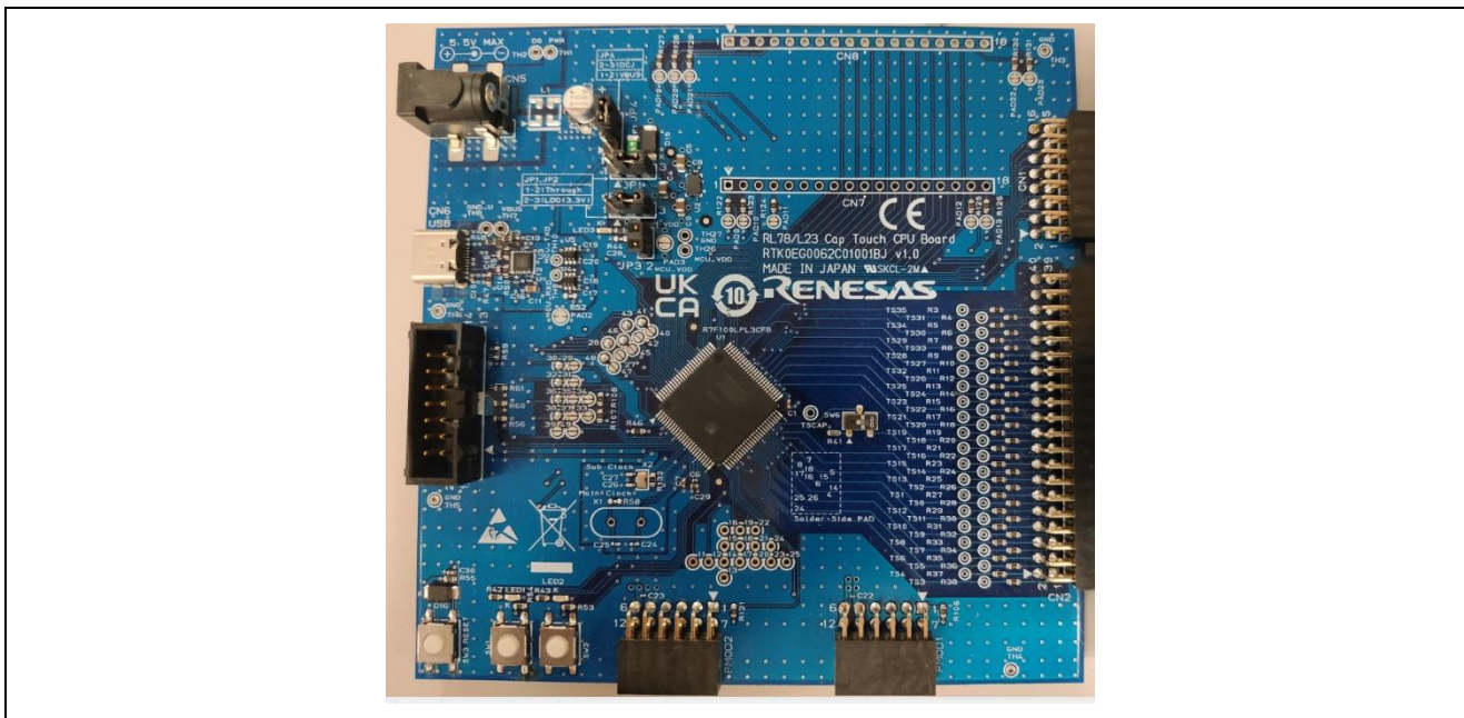
図 7.1 CPU ボード・前面
