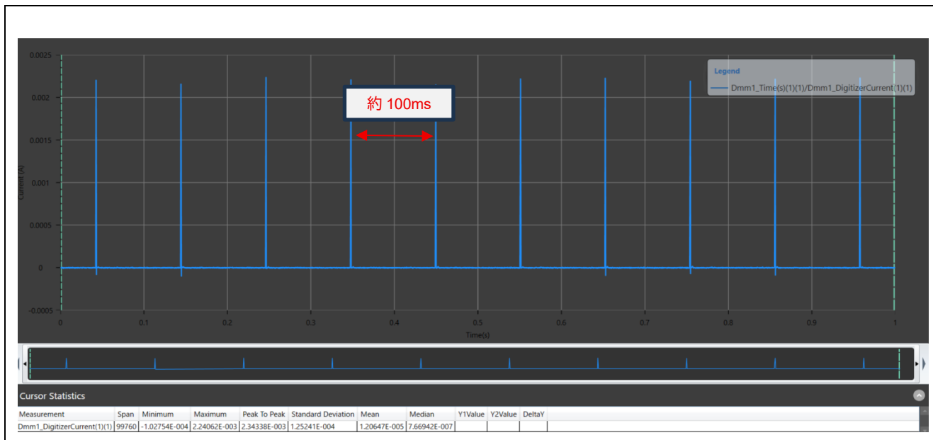
図 7.5 スタンバイモードの消費電流波形 (1/2)
