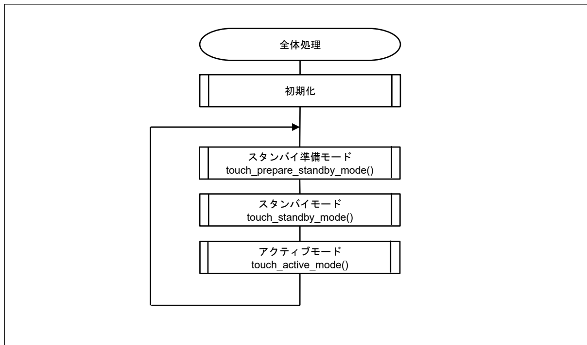
図 5.3 全体フロー
