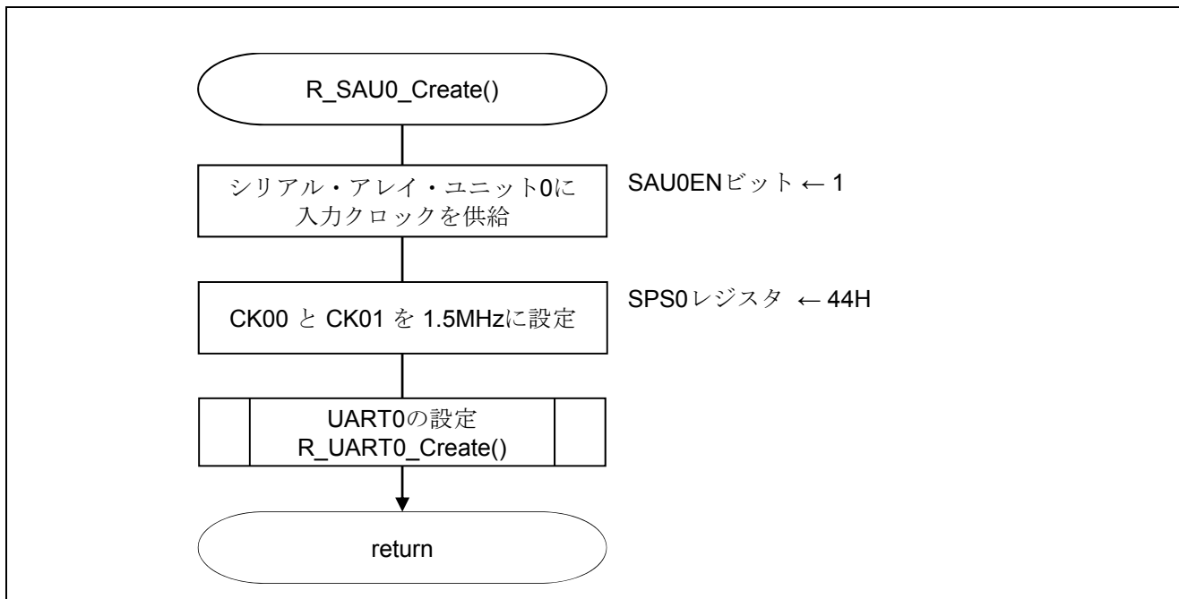
図 5.6 シリアル・アレイ・ユニットの設定
