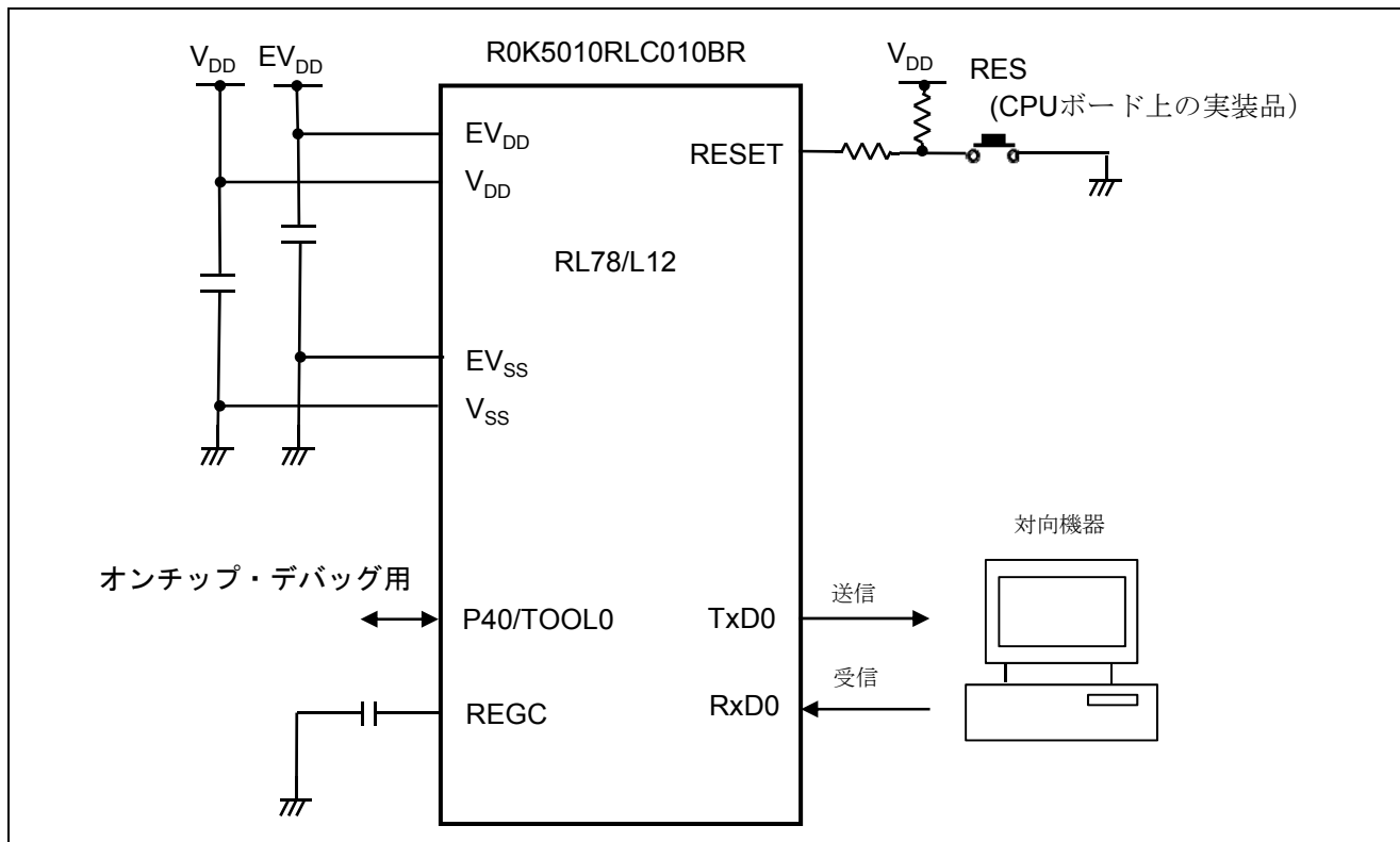
図 4.1 ハードウェア構成
