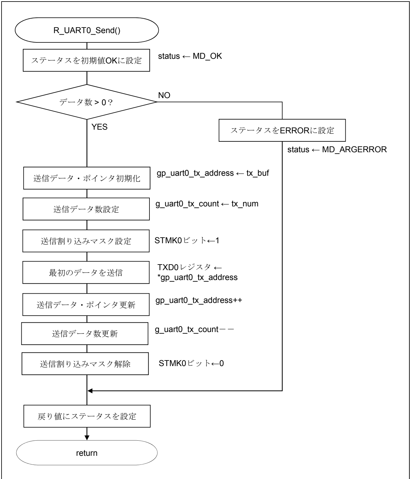
図 5.17 UART0 データ送信関数
