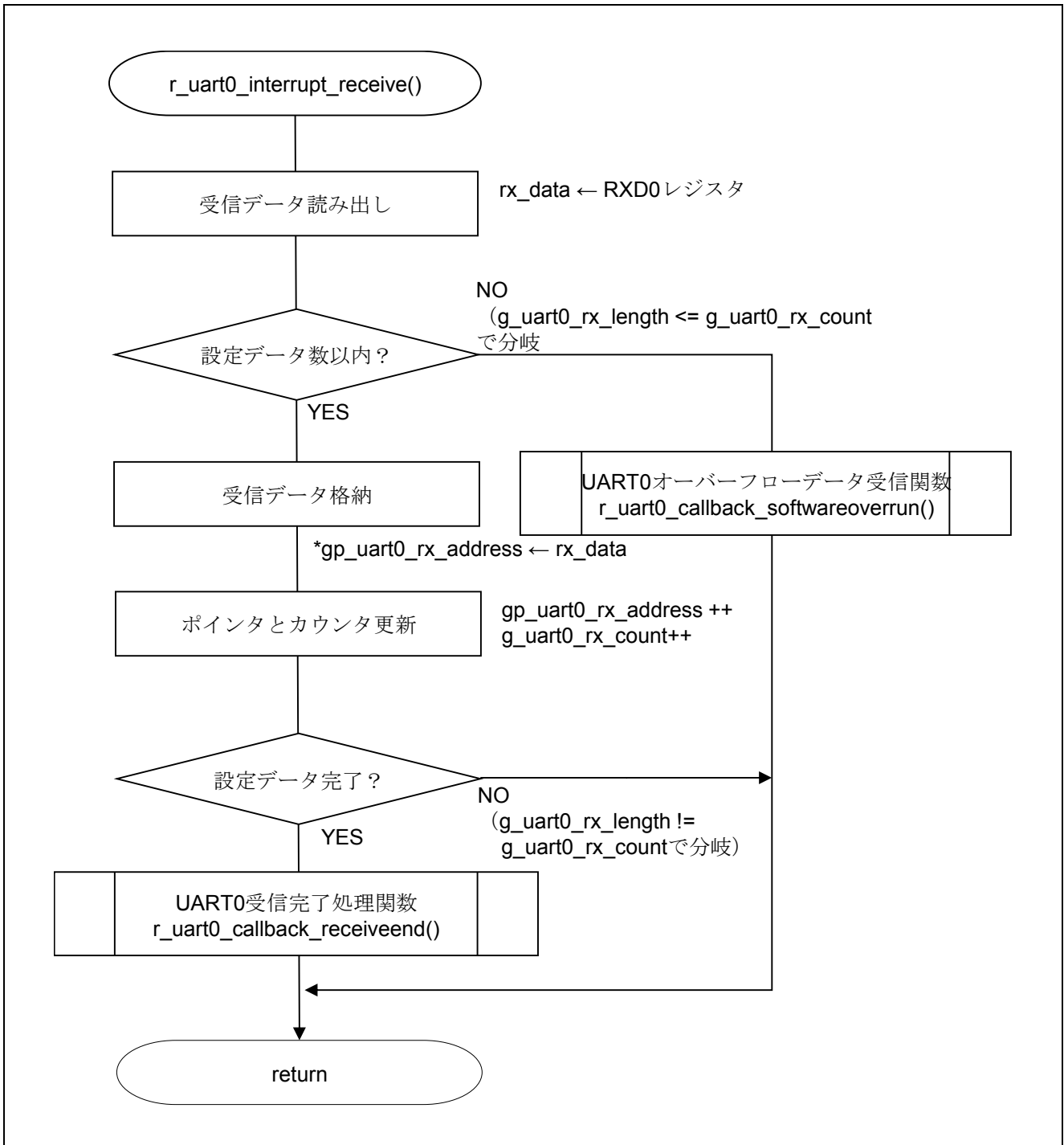
図 5.15 INTSR0 割り込みサービスルーチン
