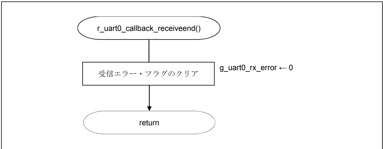
図 5.16 UART0 受信完了処理関数
