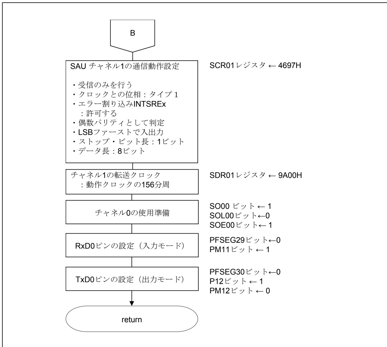
図 5.9 UART0 の設定 (3/3)
