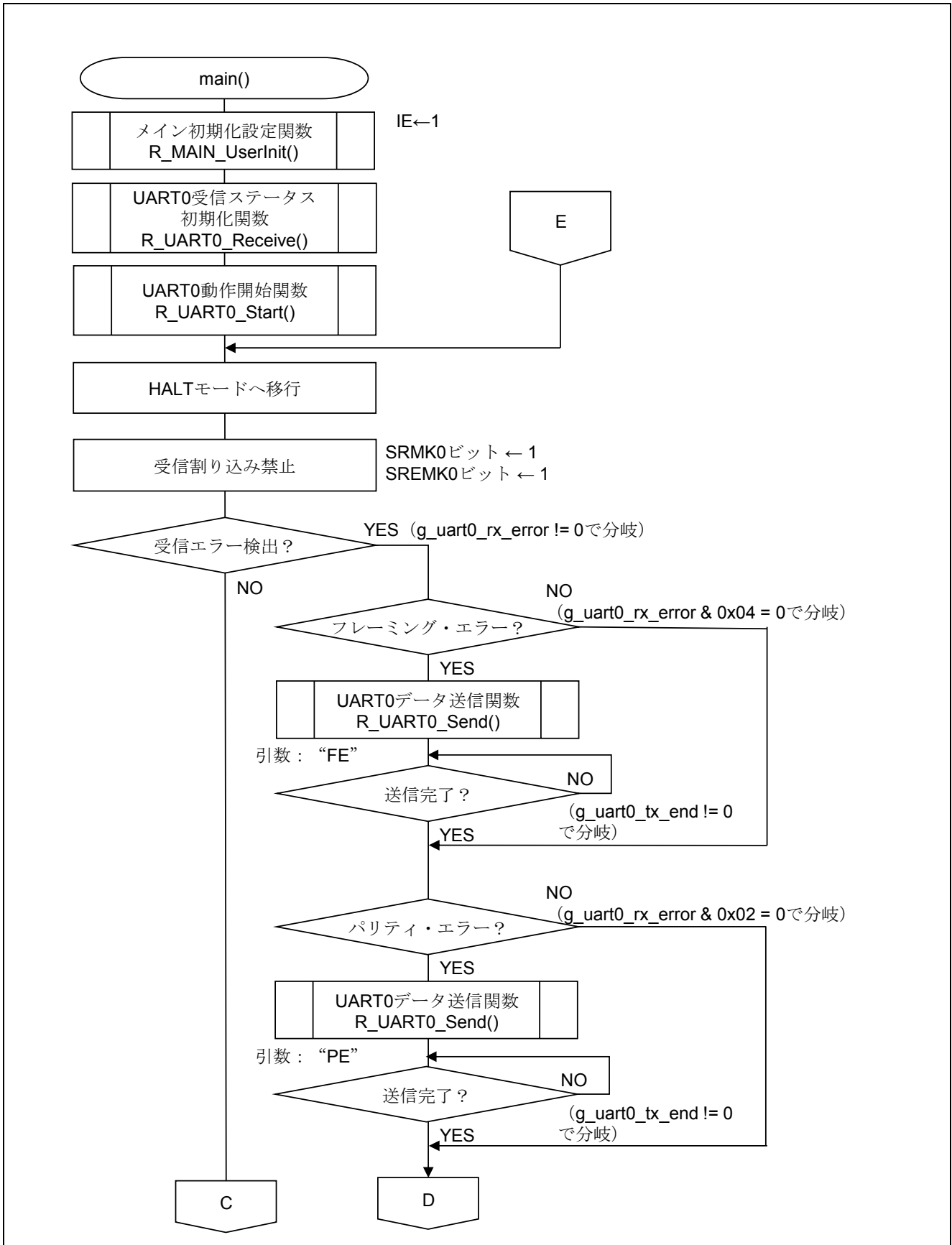
図 5.10 メイン関数 (1/2)
