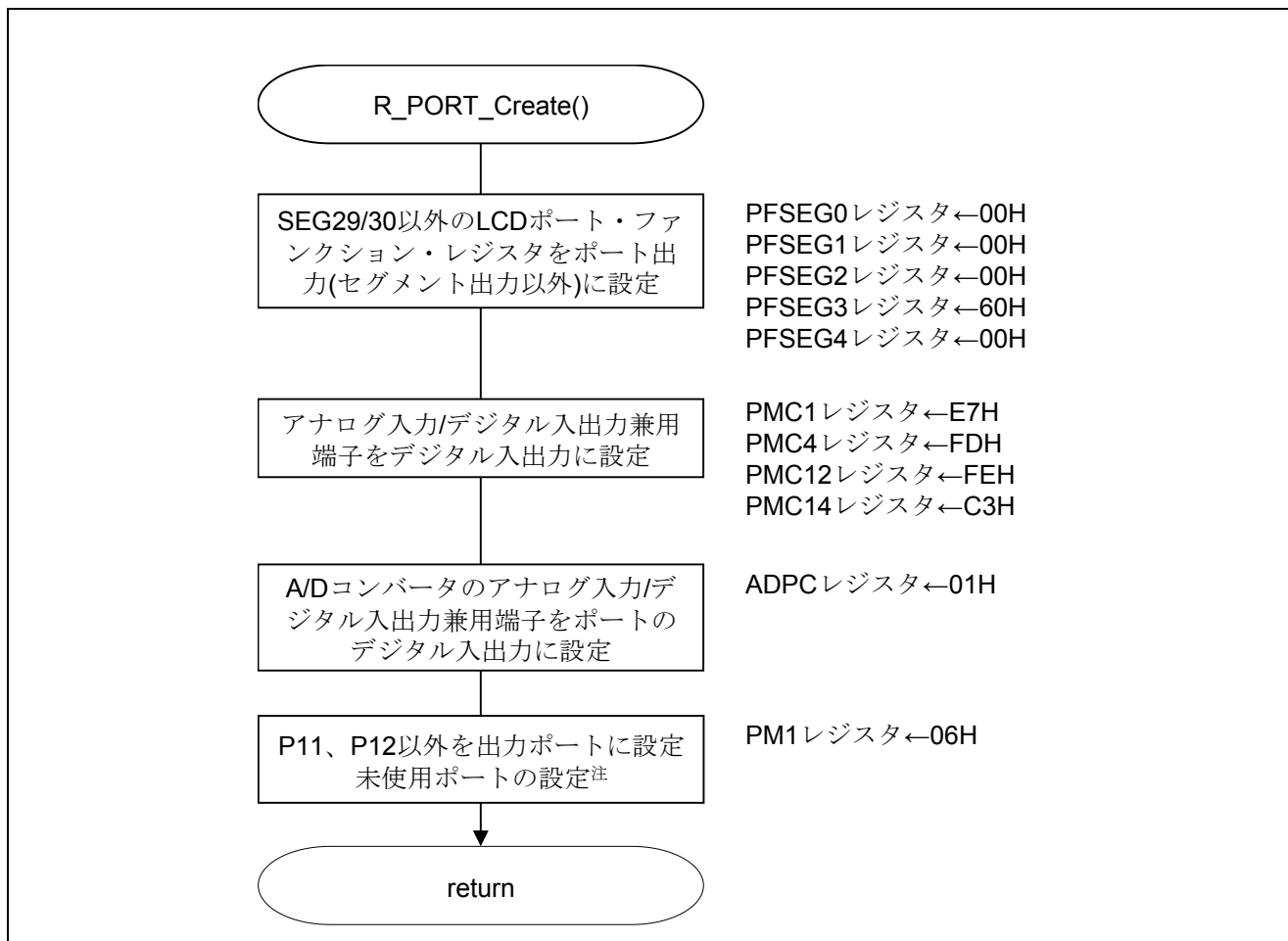
図 5.4 入出力ポートの設定
