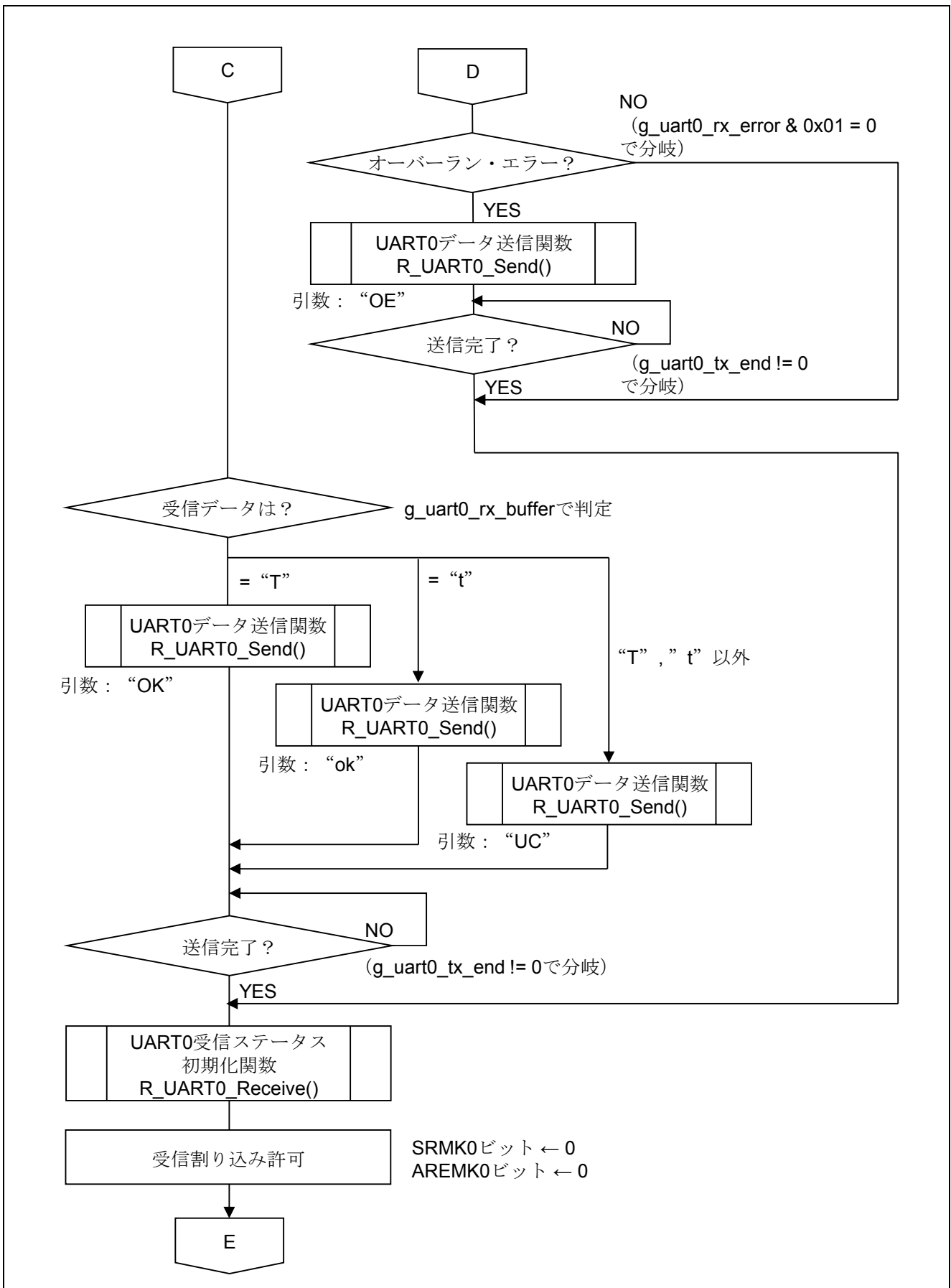
図 5.11 メイン関数 (2/2)
