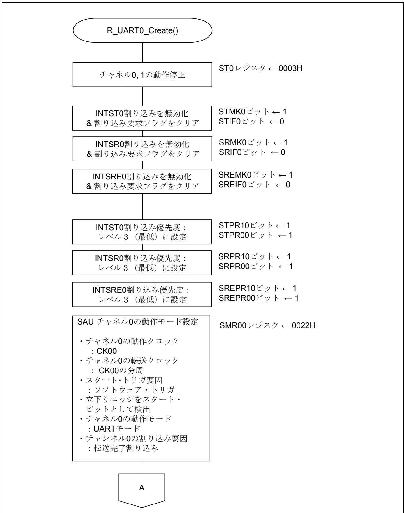
図 5.7 UART0 の設定 (1/3)
