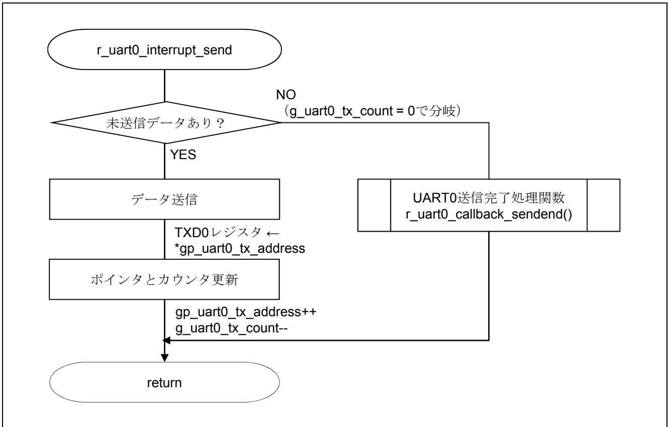
図 5.20 INTST0 割り込みサービスルーチン
