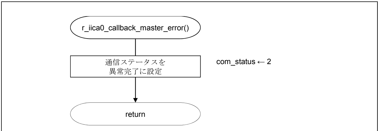
図 5.20 エラー・フラグ返却処理
