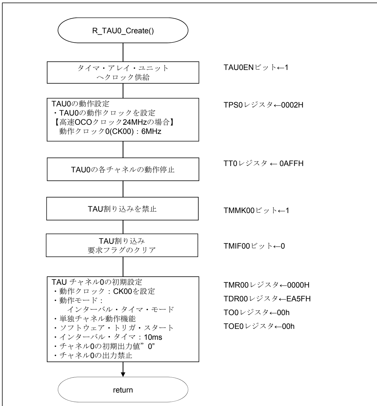
図 5.7 タイマ・アレイ・ユニットの設定
