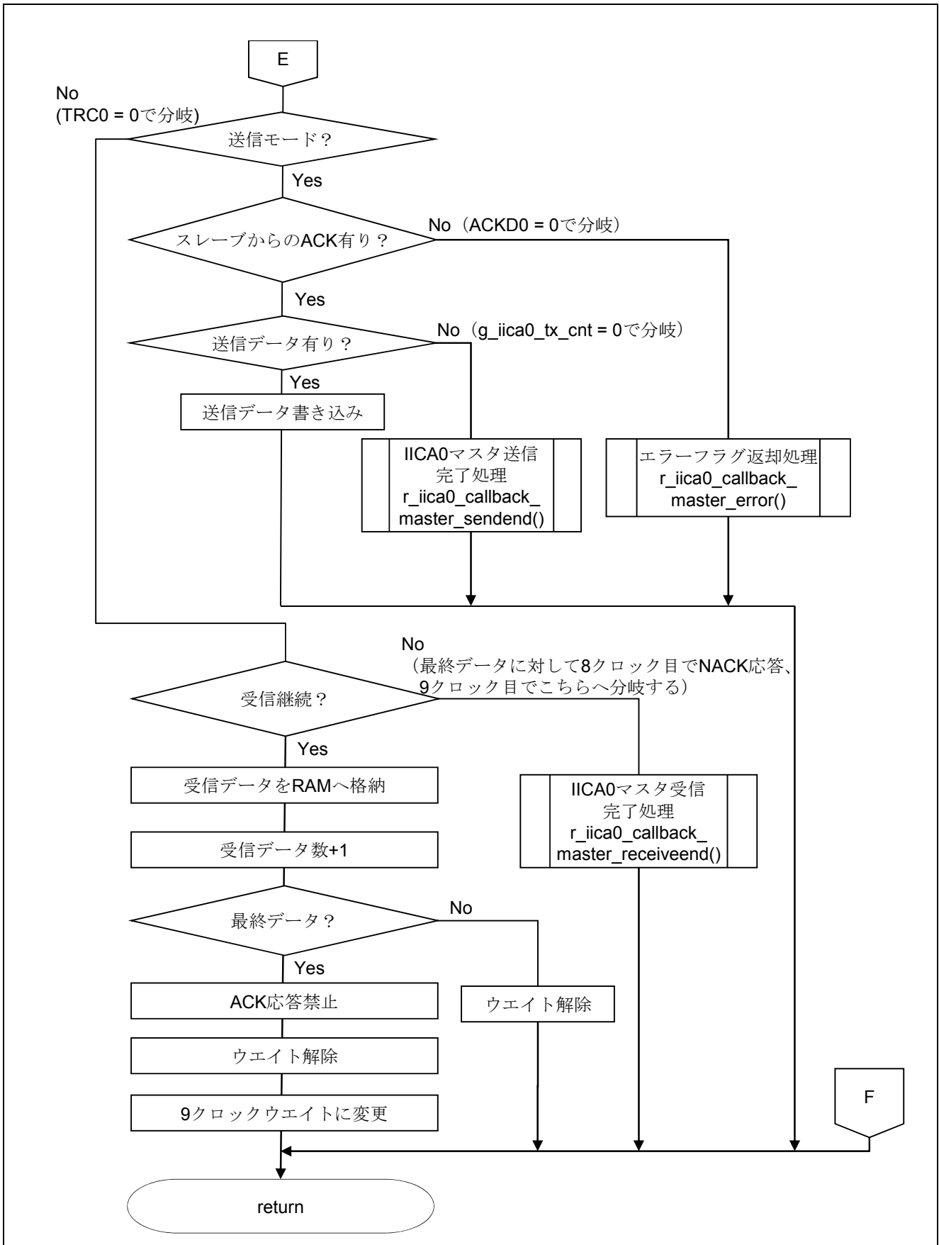
図 5.17 IICA0 マスタ通信処理 (2/2)
