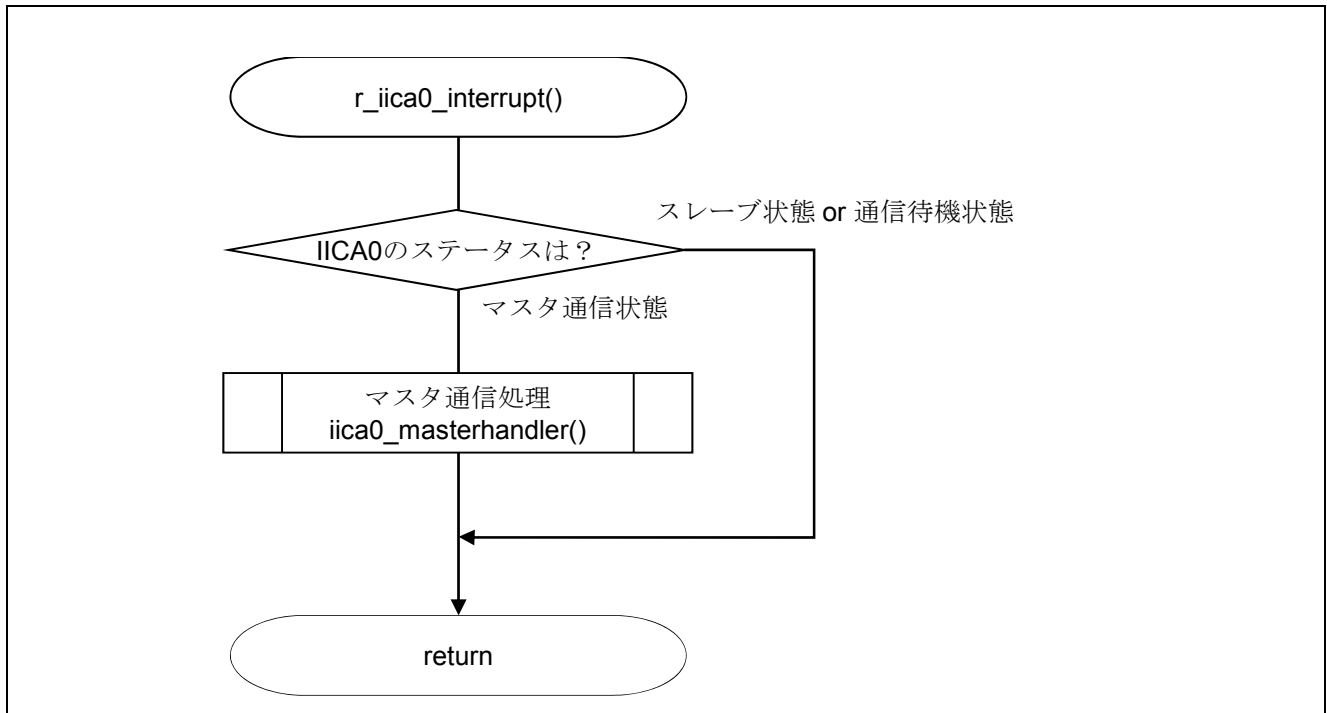
図 5.15 IICA0 割り込み処理
