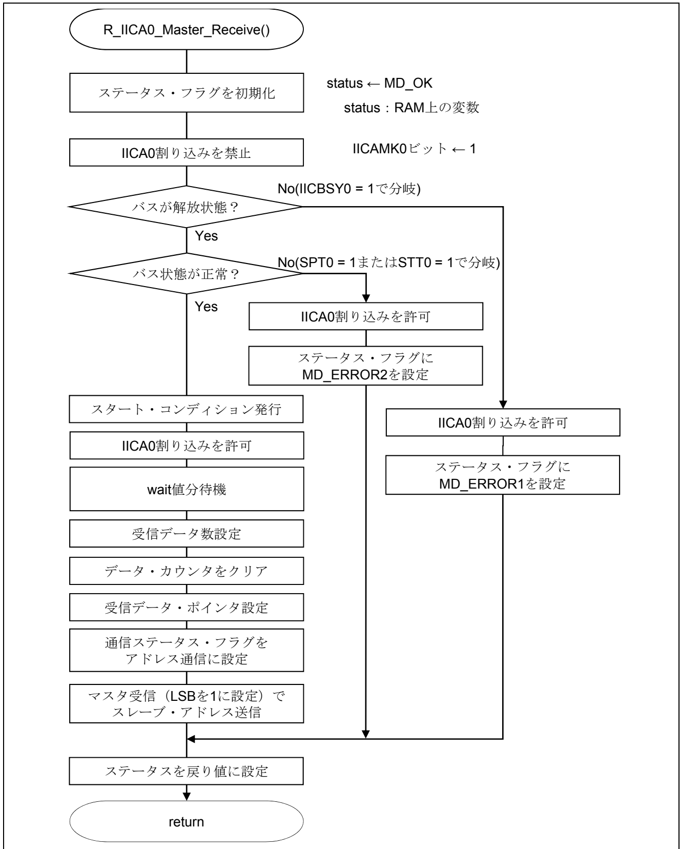
図 5.14 マスタ受信開始要求処理
