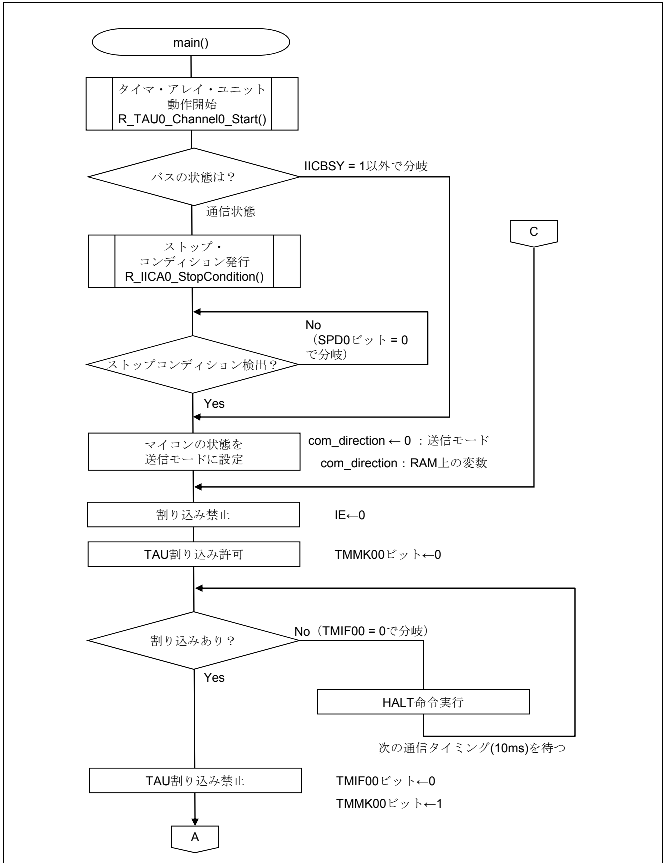
図 5.8 メイン関数 (1/3)
