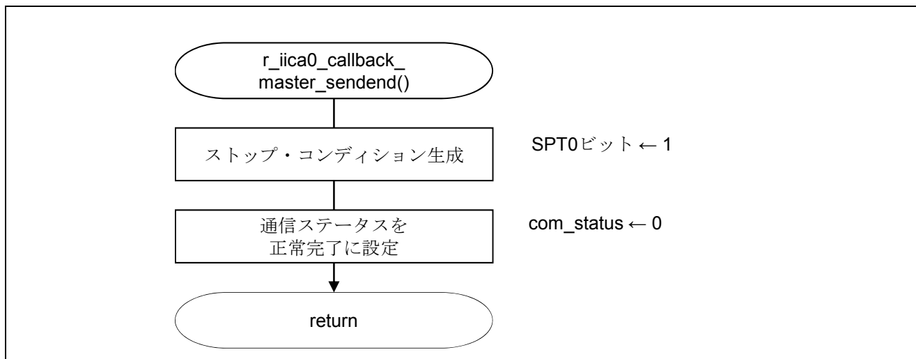
図 5.19 IICA0 マスタ送信完了処理
