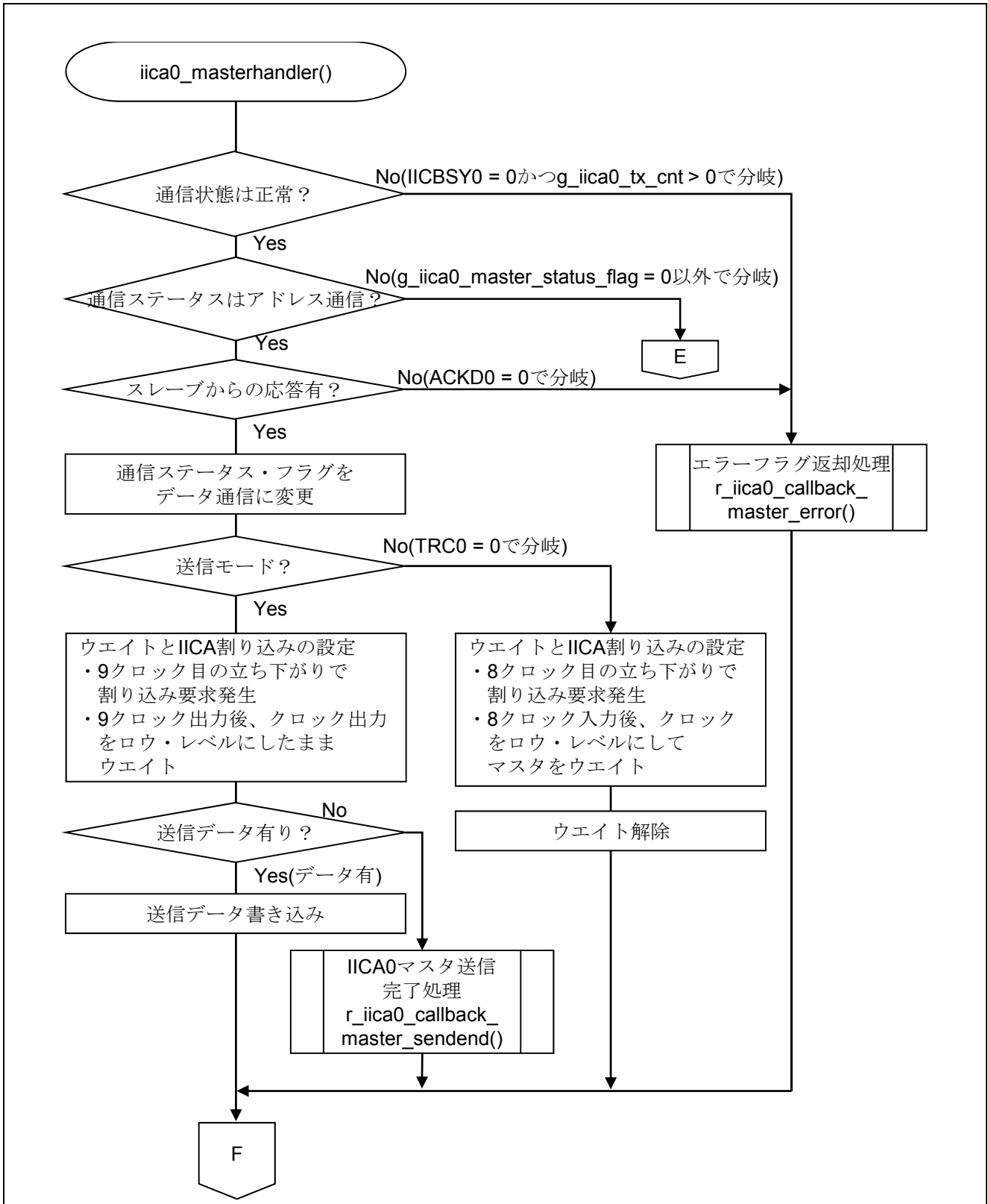
図 5.16 IICA0 マスタ通信処理 (1/2)
