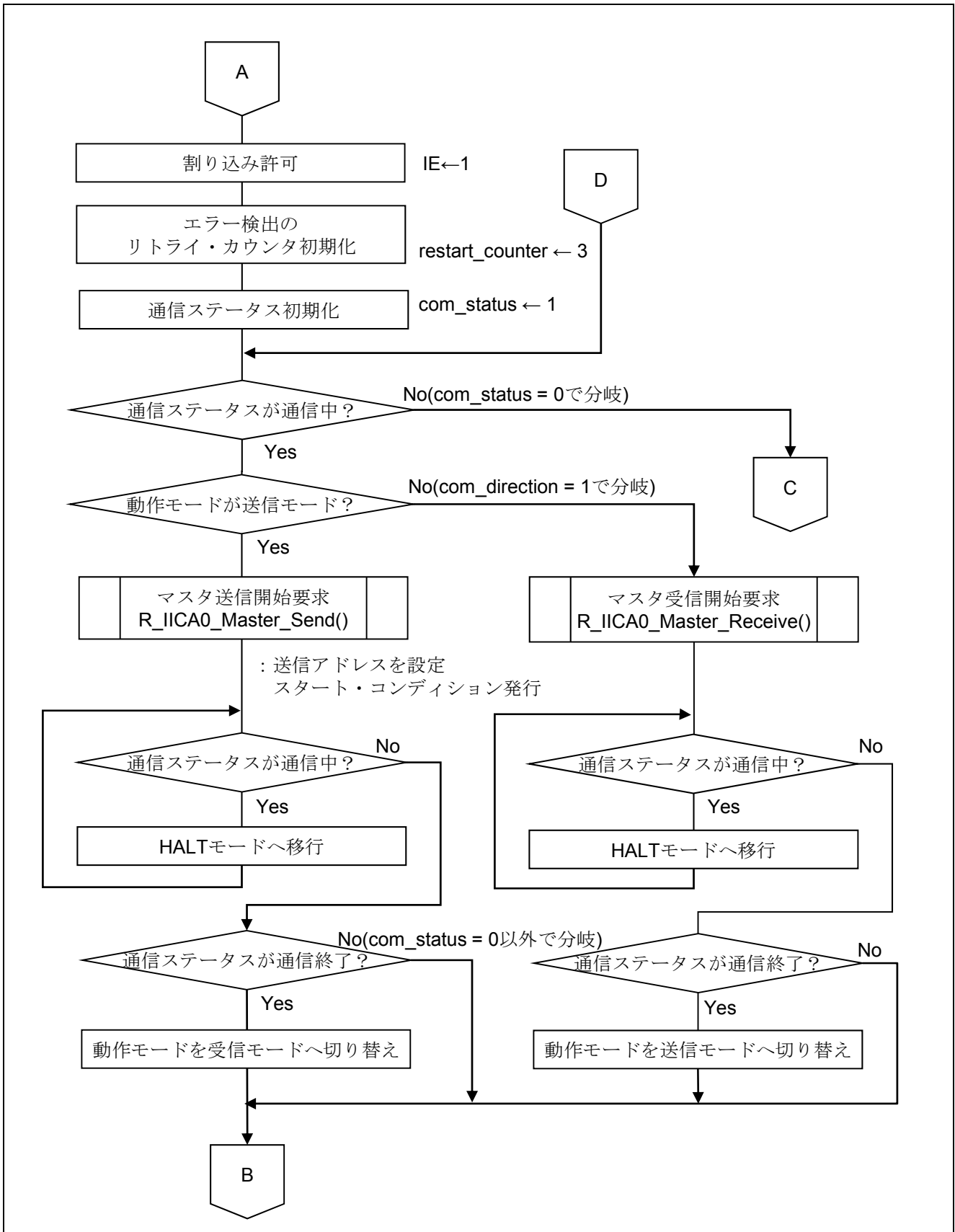
図 5.9 メイン関数 (2/3)
