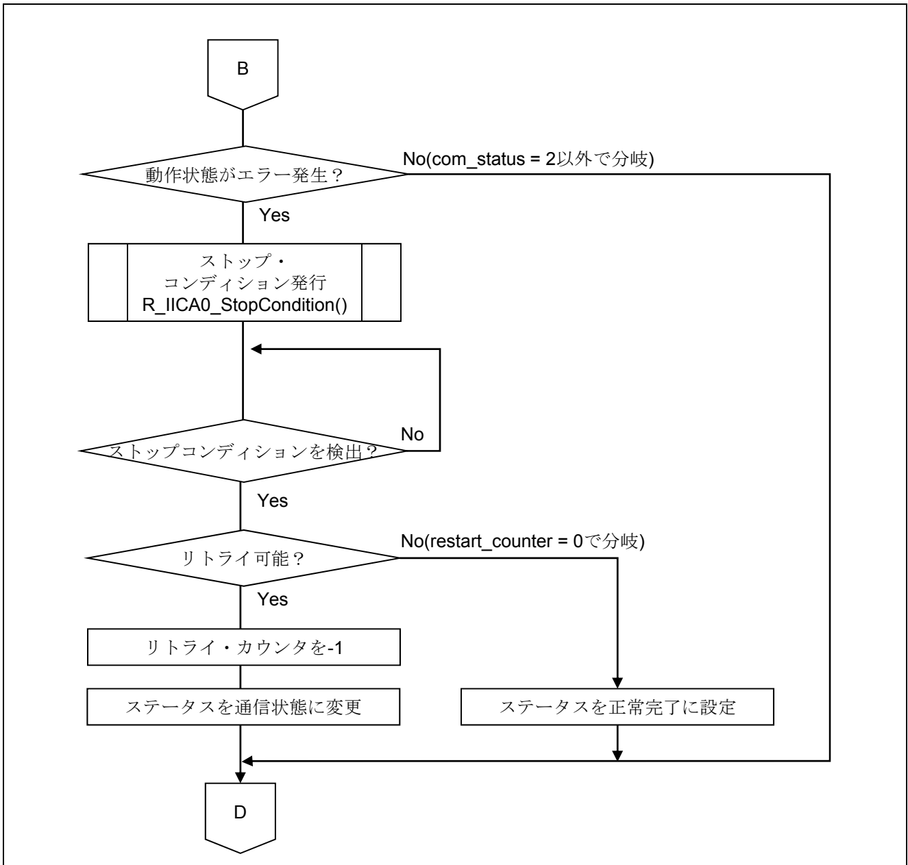
図 5.10 メイン関数 (3/3)
