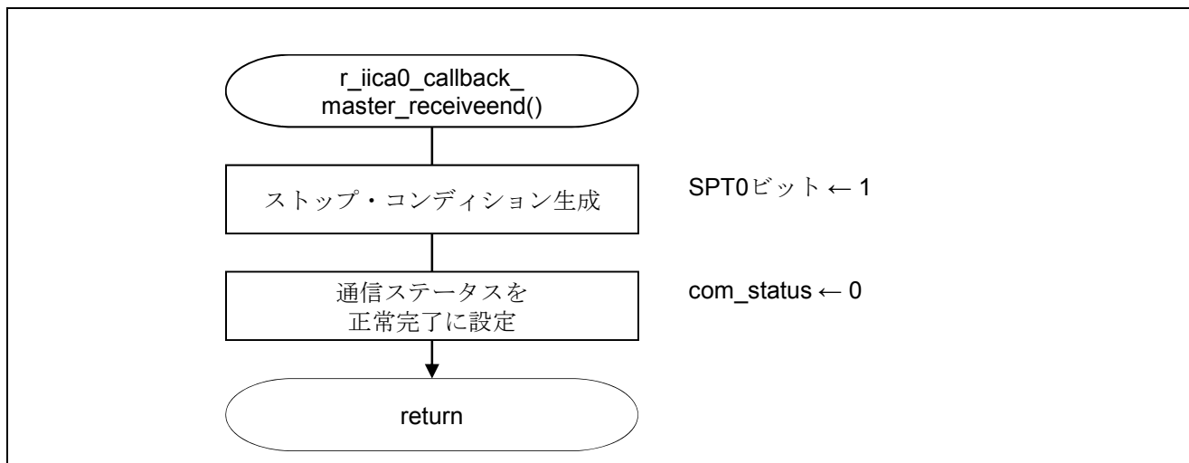
図 5.18 IICA0 マスタ受信完了処理
