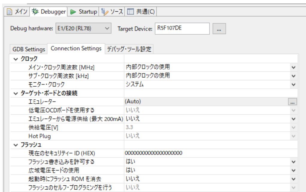
図 4-5 デバッグ画面設定内容
