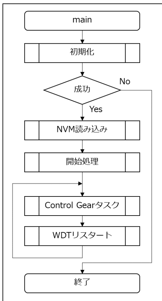
図 4-13 メインフロー図
