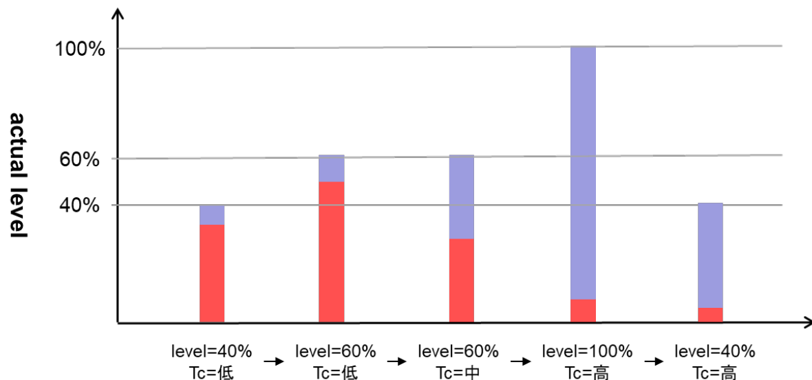
図 4-10 総調光率 (actual level)と各温度域 LED の調光率の比
