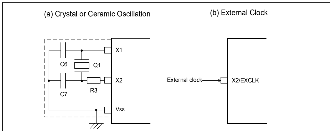
図 8. メイン・システム・クロックの接続
