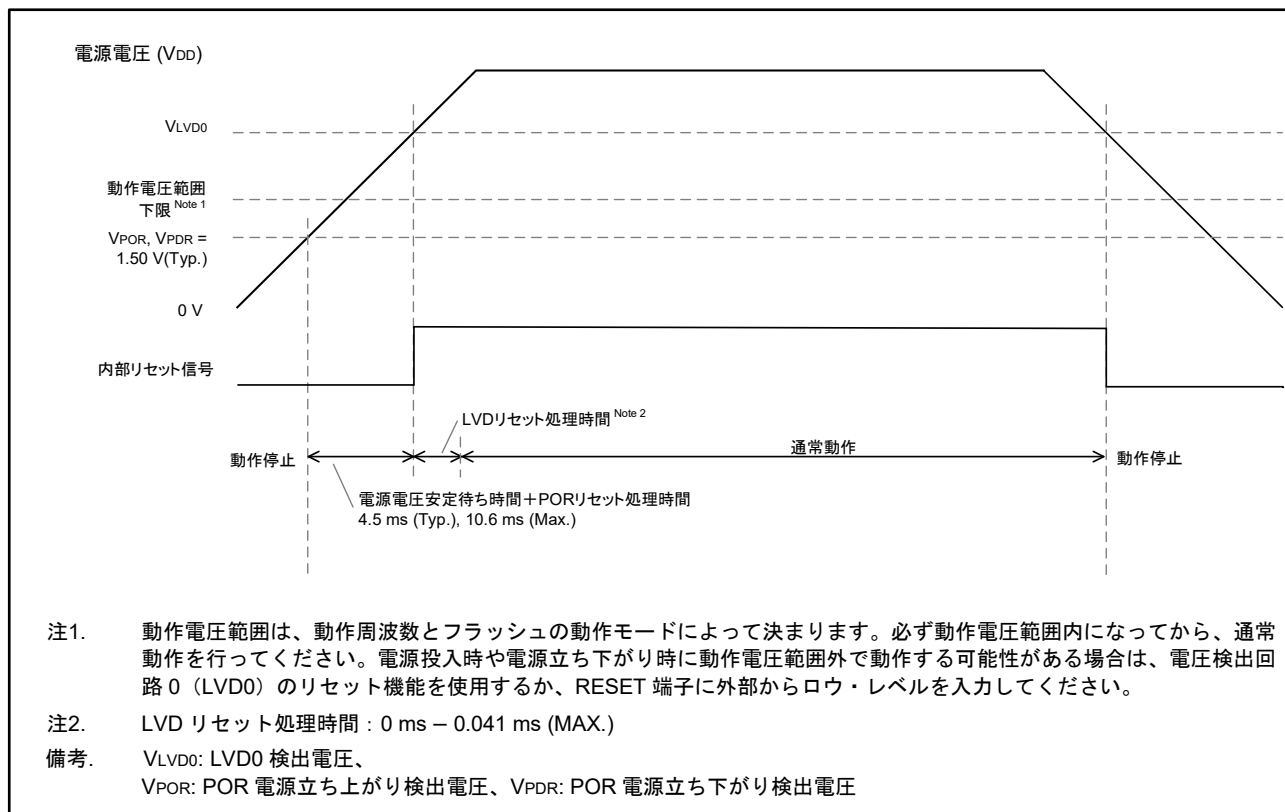
図 4. LVD0 使用時の電源供給タイミング
