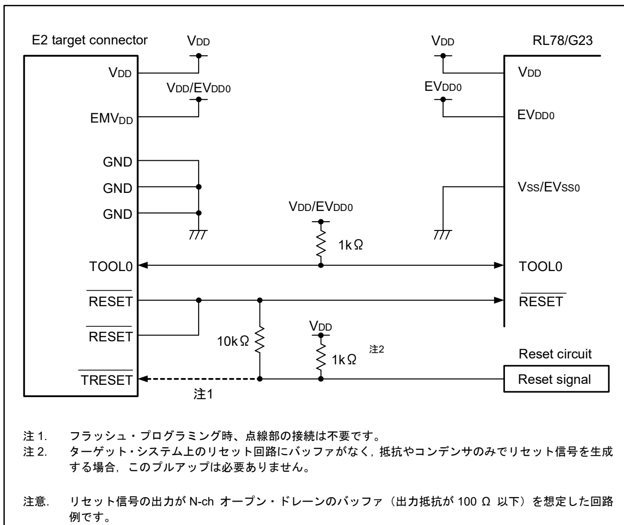
図 15. RL78/G23 と E2 エミュレータの接続例
