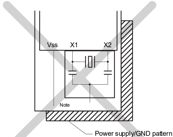
(d) X1, X2 配線の下に電源/GND パターンがある
