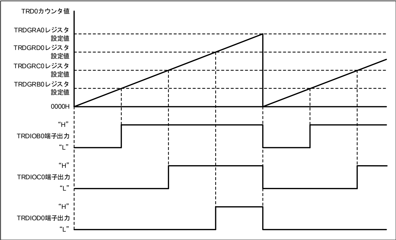
図 1-1 PWM の出力波形
