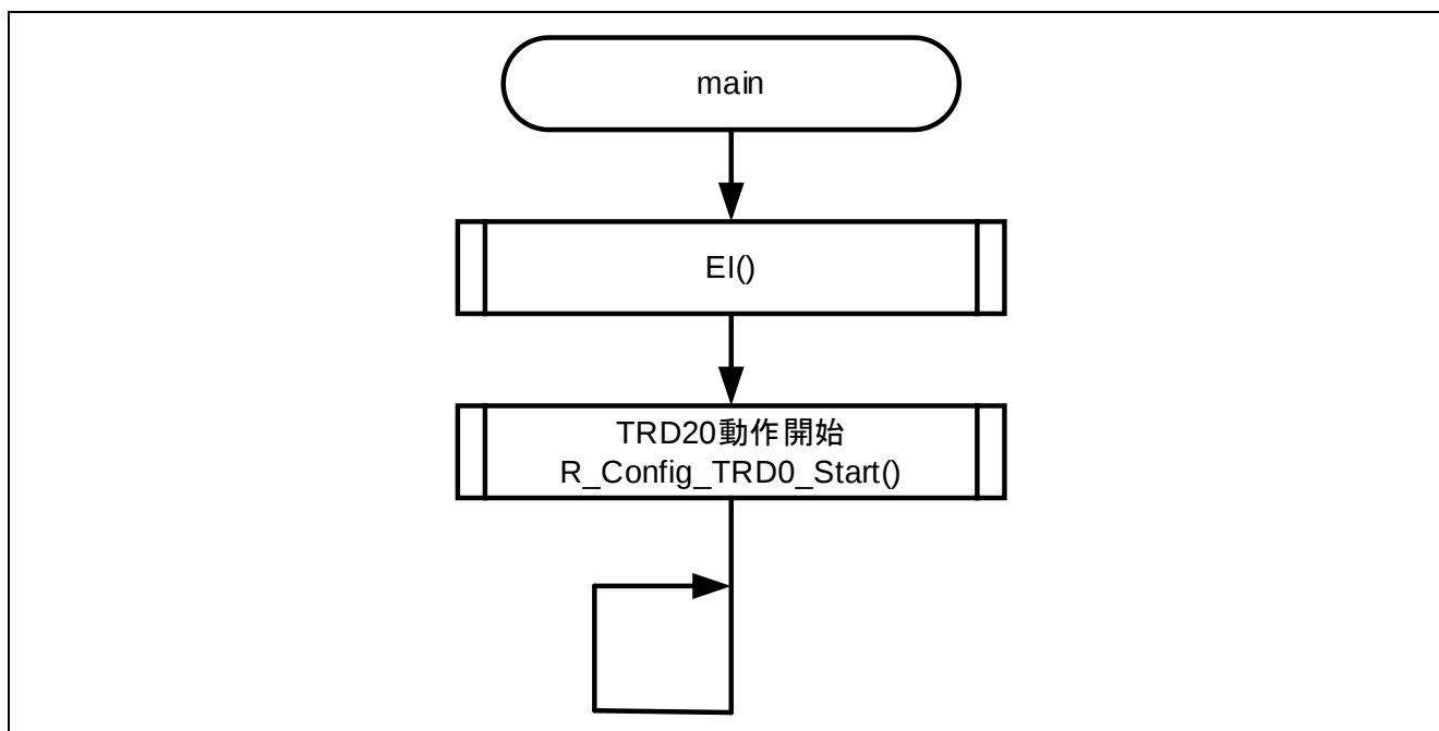
図 4-4 メイン処理
