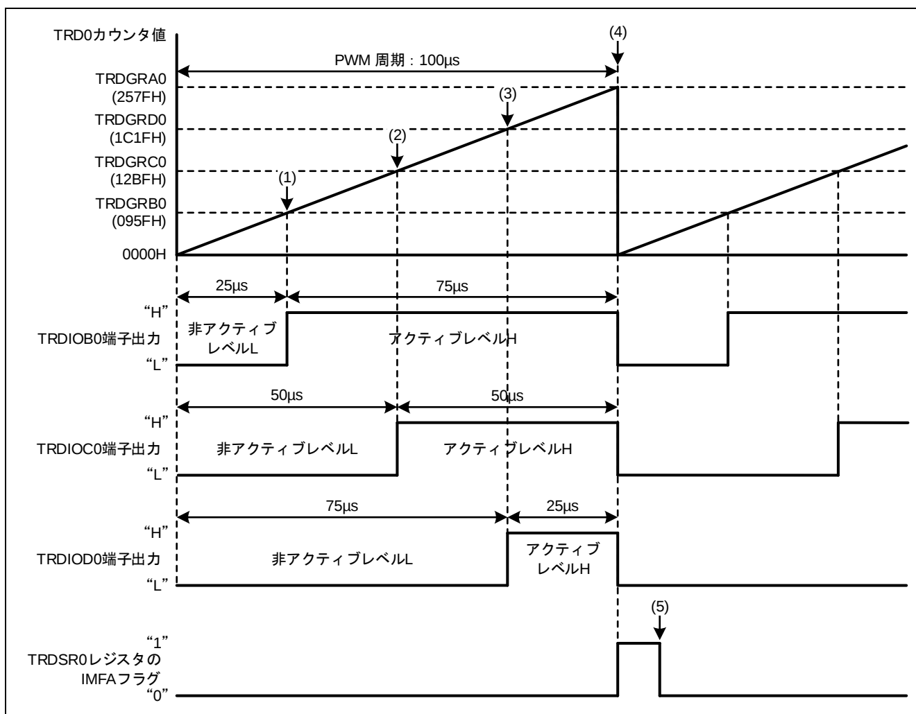
図 1-2 タイマ RD2 の PWM 機能のタイミング
