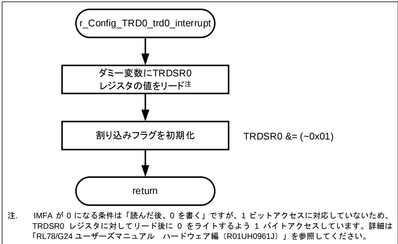
図 4-5 r_Config_TRD0_trd0_interrupt 関数
