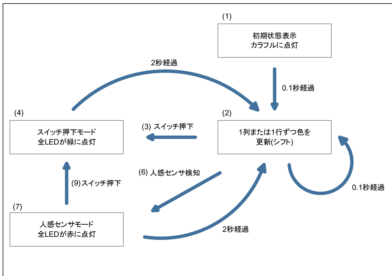
図 4-3 動作概要
