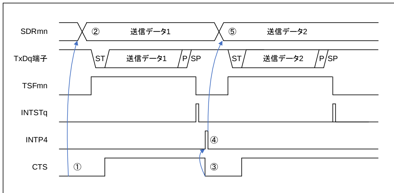
図 1-3 UART 送信のタイミングチャート
