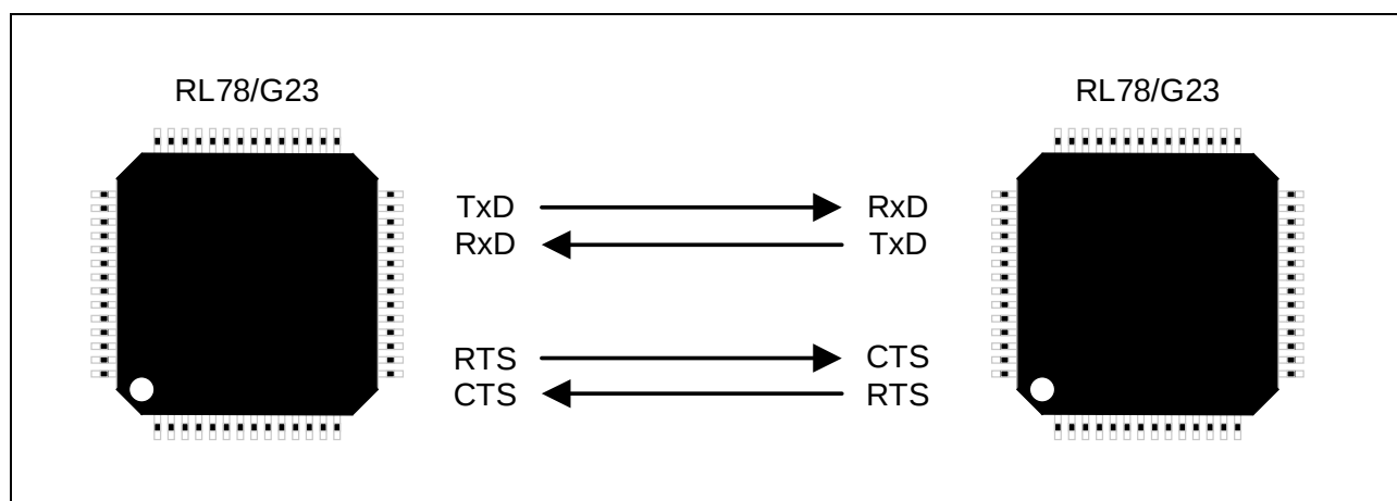
図 1-1 フロー制御の構成図
