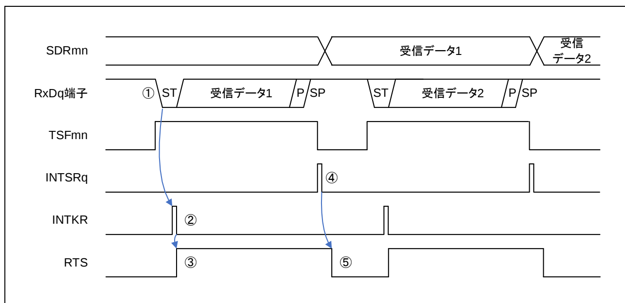
図 1-2 データ受信時のタイミングチャート
