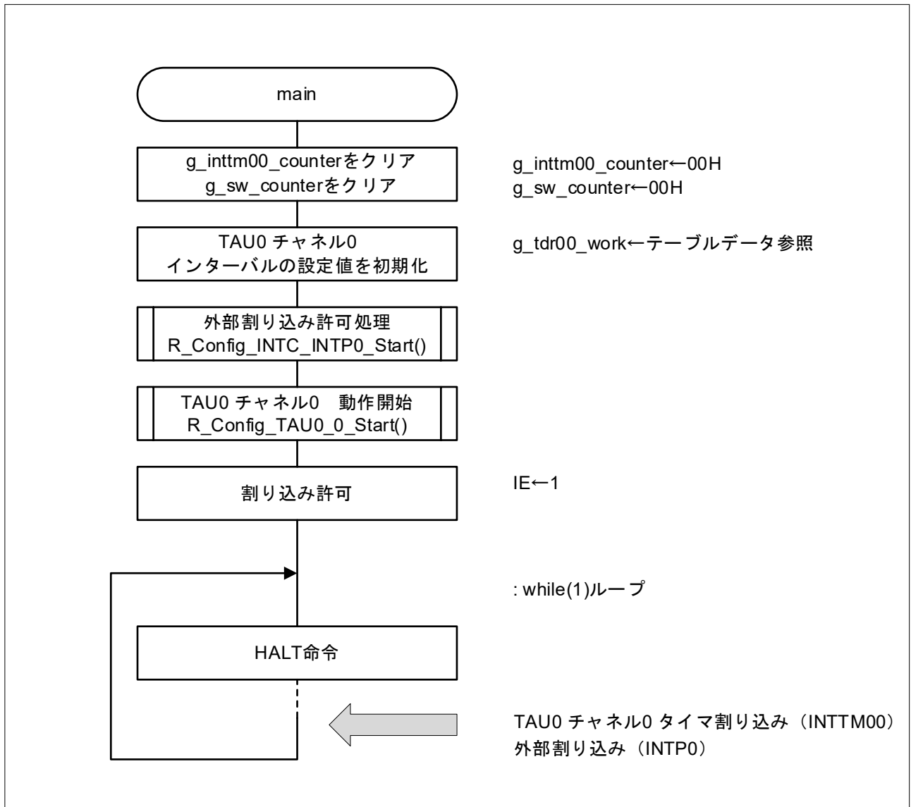
図 4-1 メイン処理
