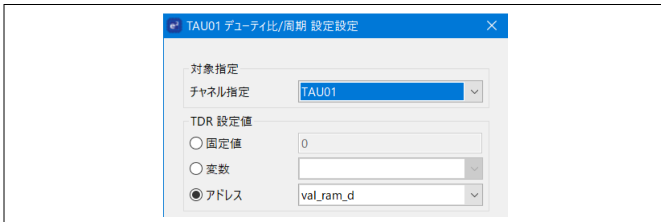
図 6-3 TAU01 デューティ比／周期 設定
