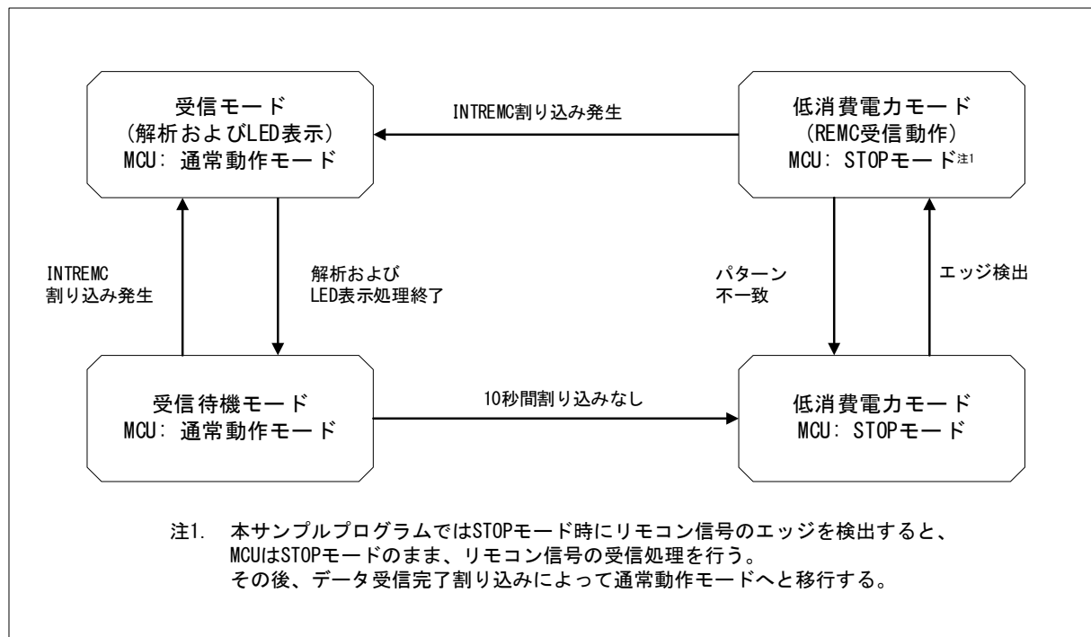
図 1-4 リモコン信号受信の状態遷移図
