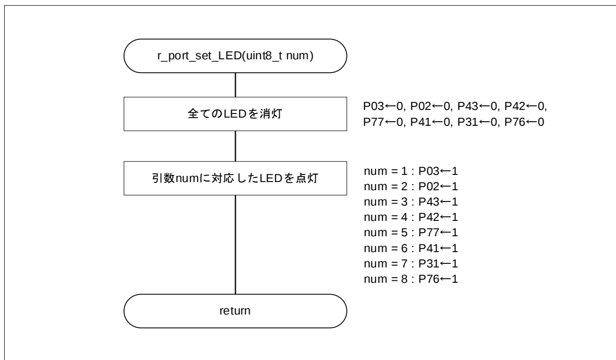
図 4-8 LED 点灯制御
