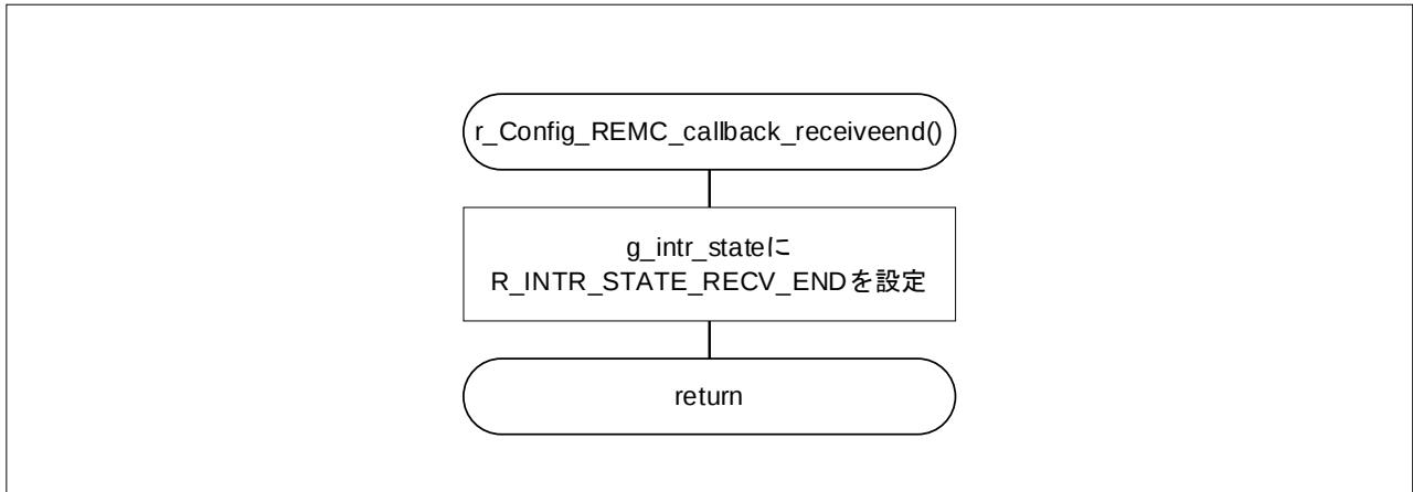
図 4-4 REMC 受信完了割り込み
