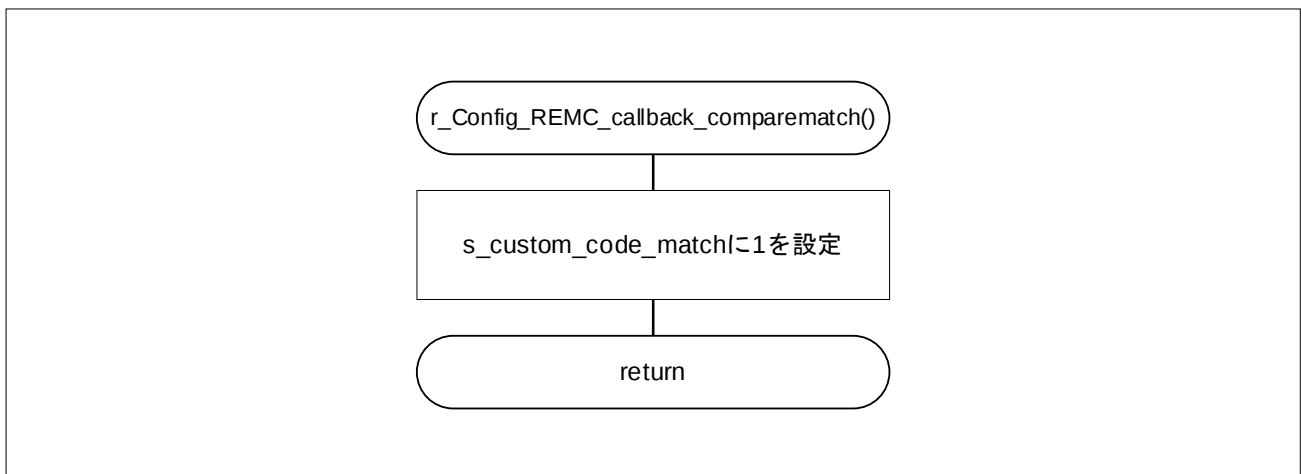
図 4-5 REMC コンペア一致割り込み
