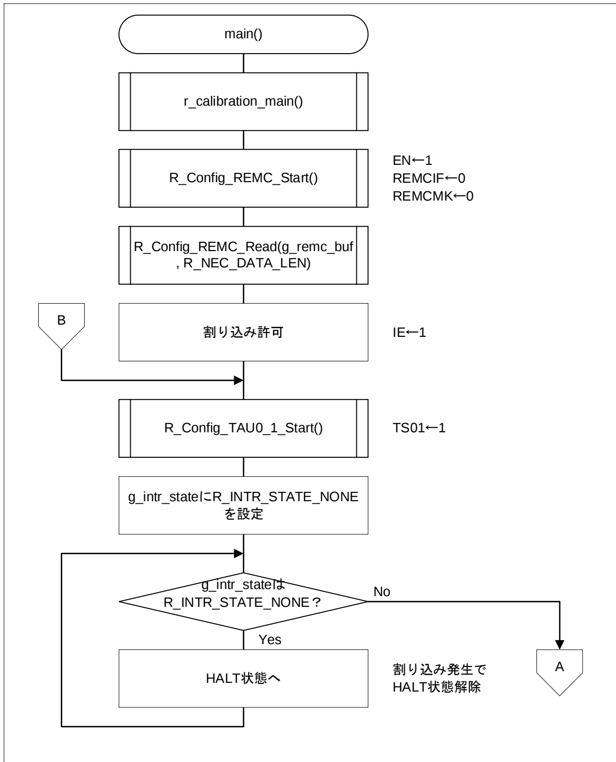
図 4-1 メイン処理 (1/2)
