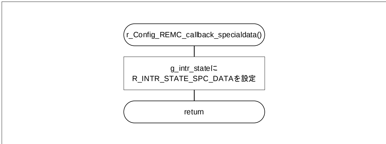
図 4-6 REMC 特殊データ・パターン受信割り込み
