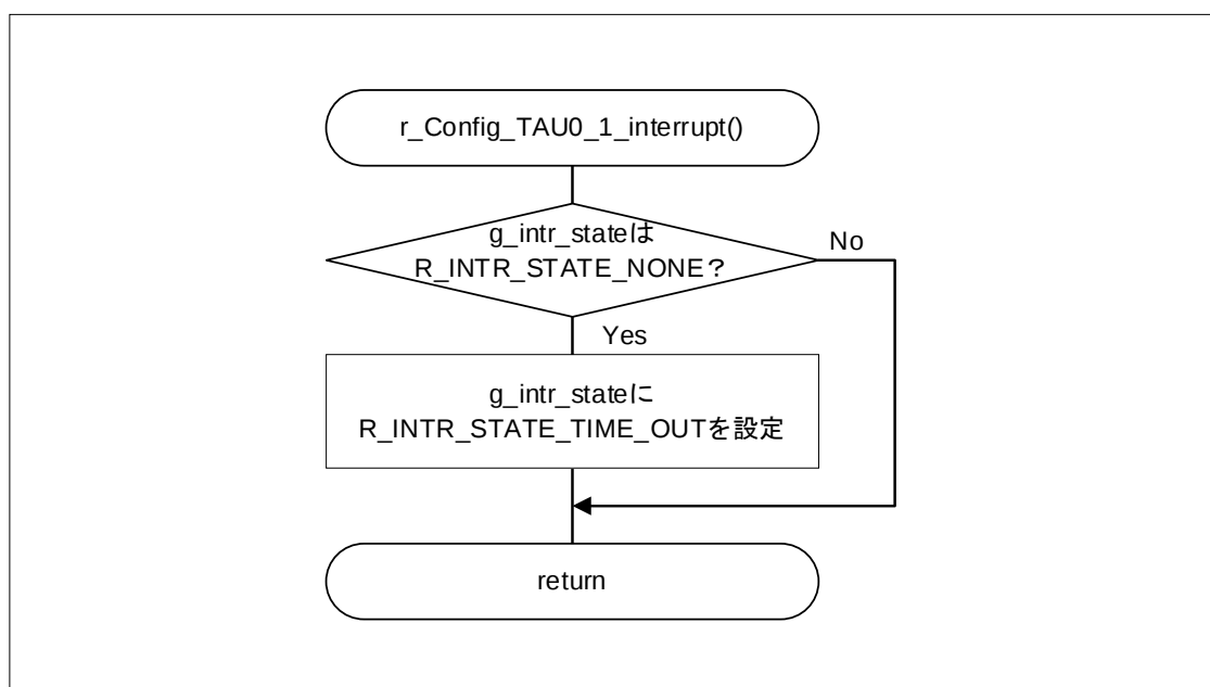
図 4-9 STOP モード移行用タイマ割り込み
