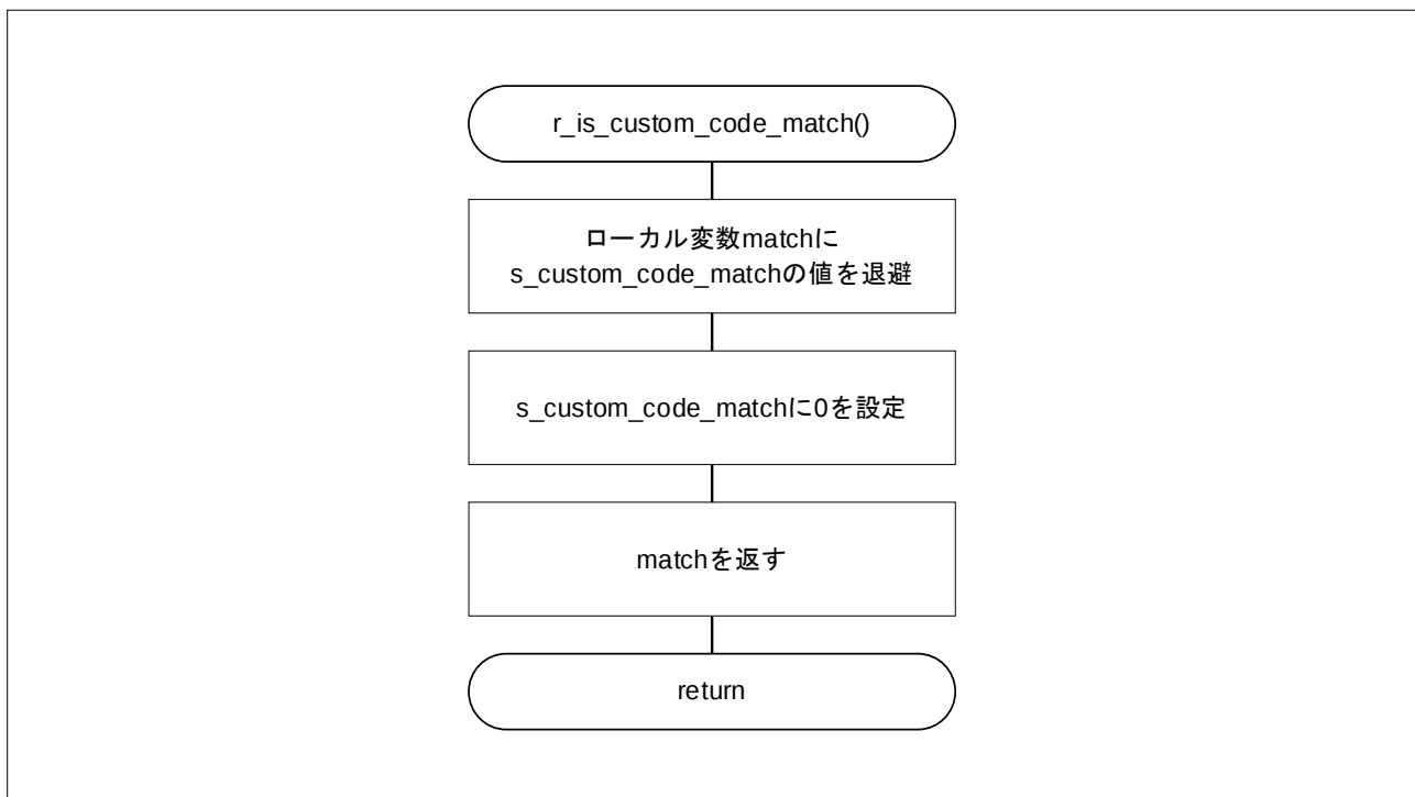
図 4-7 コンペアー一致発生確認
