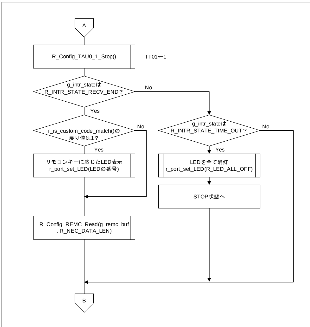
図 4-2 メイン処理 (2/2)
