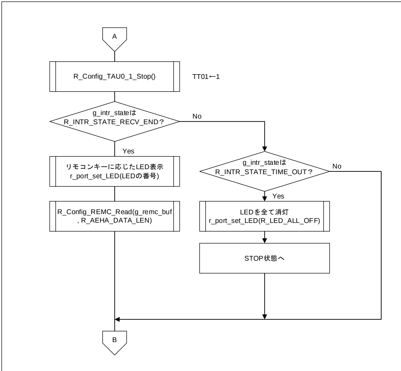
図 4-2 メイン処理 (2/2)
