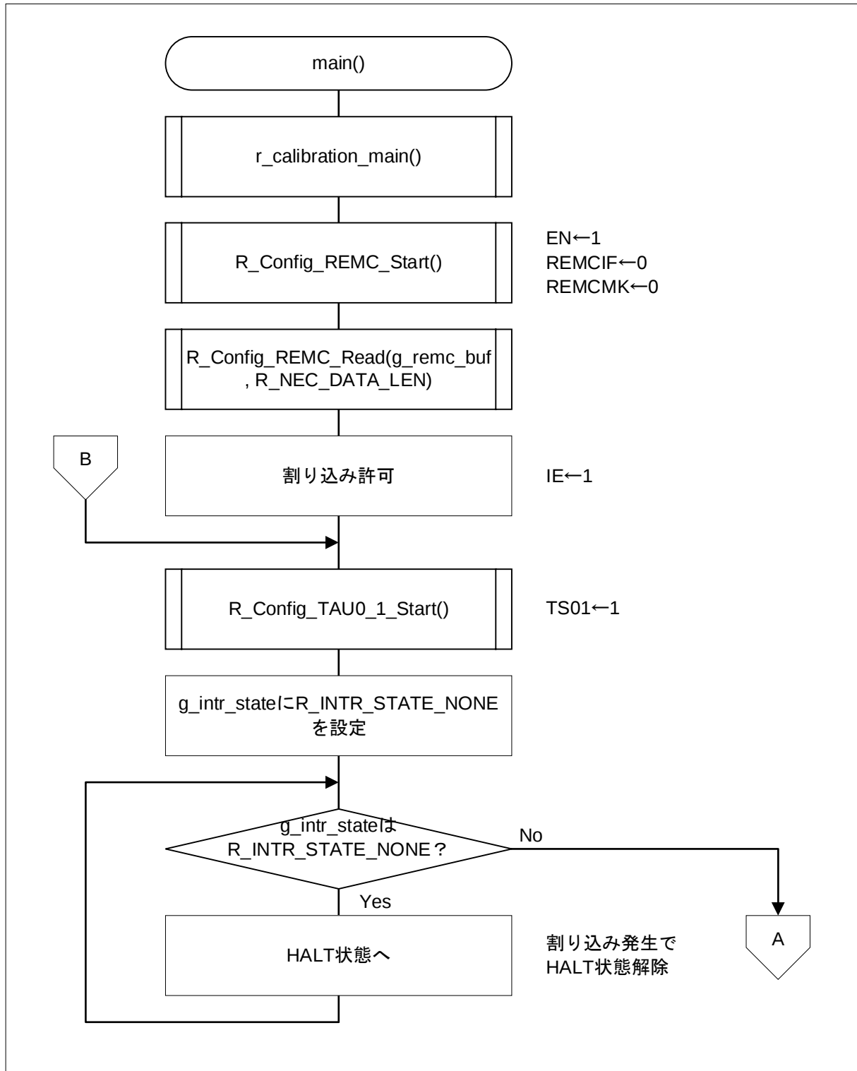
図 4-1 メイン処理 (1/2)
