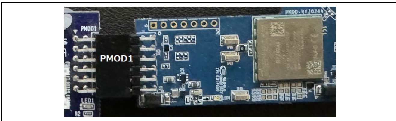
図 4-4 RYZ024A をマイコンボードの PMOD1 に接続
