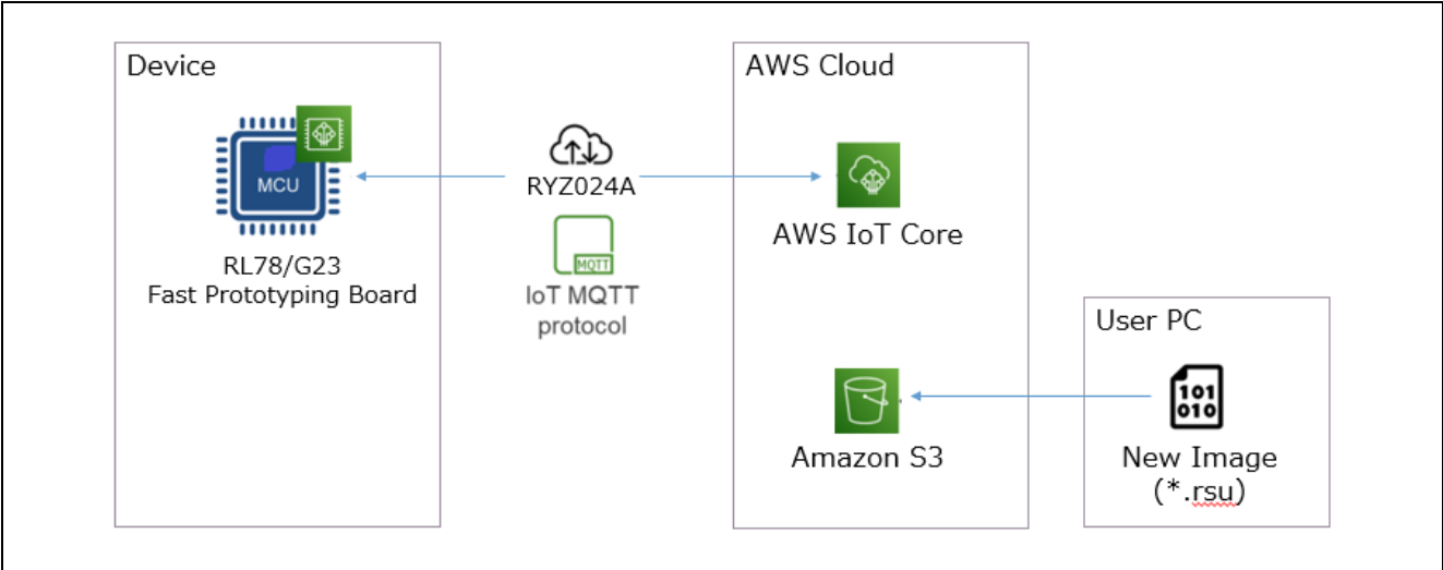
図 2-2 デモプロジェクト(OTA)のシステム構成
