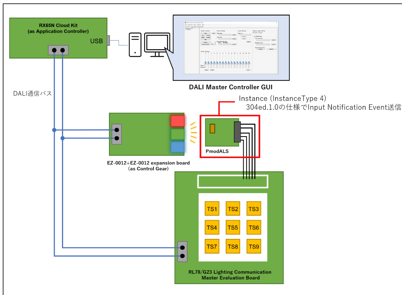
図 4-5 システム構成例(RX65N Cloud kit + DALI-2 オプションボード使用)
