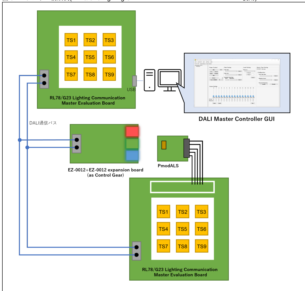
図 3-2 システム構成例(RL78/G23 Lighting Communication Master Evaluation Board 使用)
