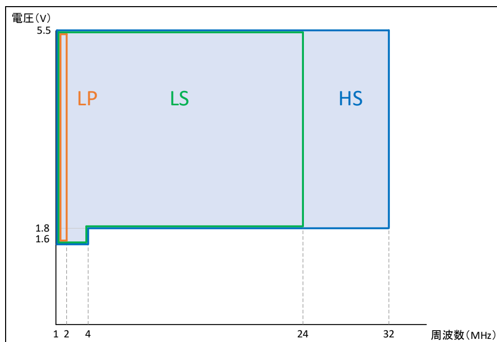
図 1-3 各フラッシュの動作モードの動作範囲
