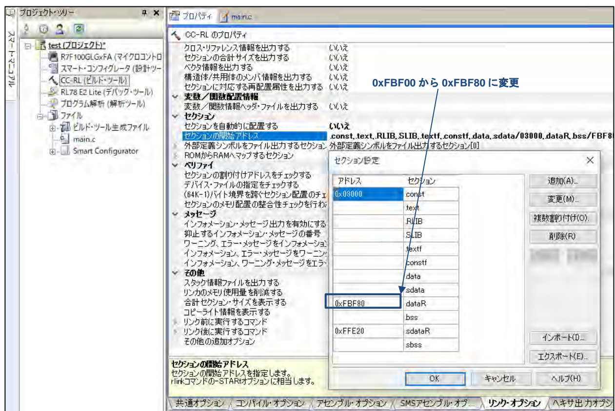
図 2-5 セクション設定（R7F100GLG の場合）
