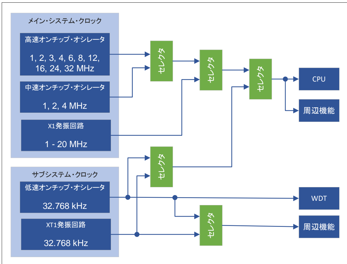
図 5-1 クロック発生回路の構成
