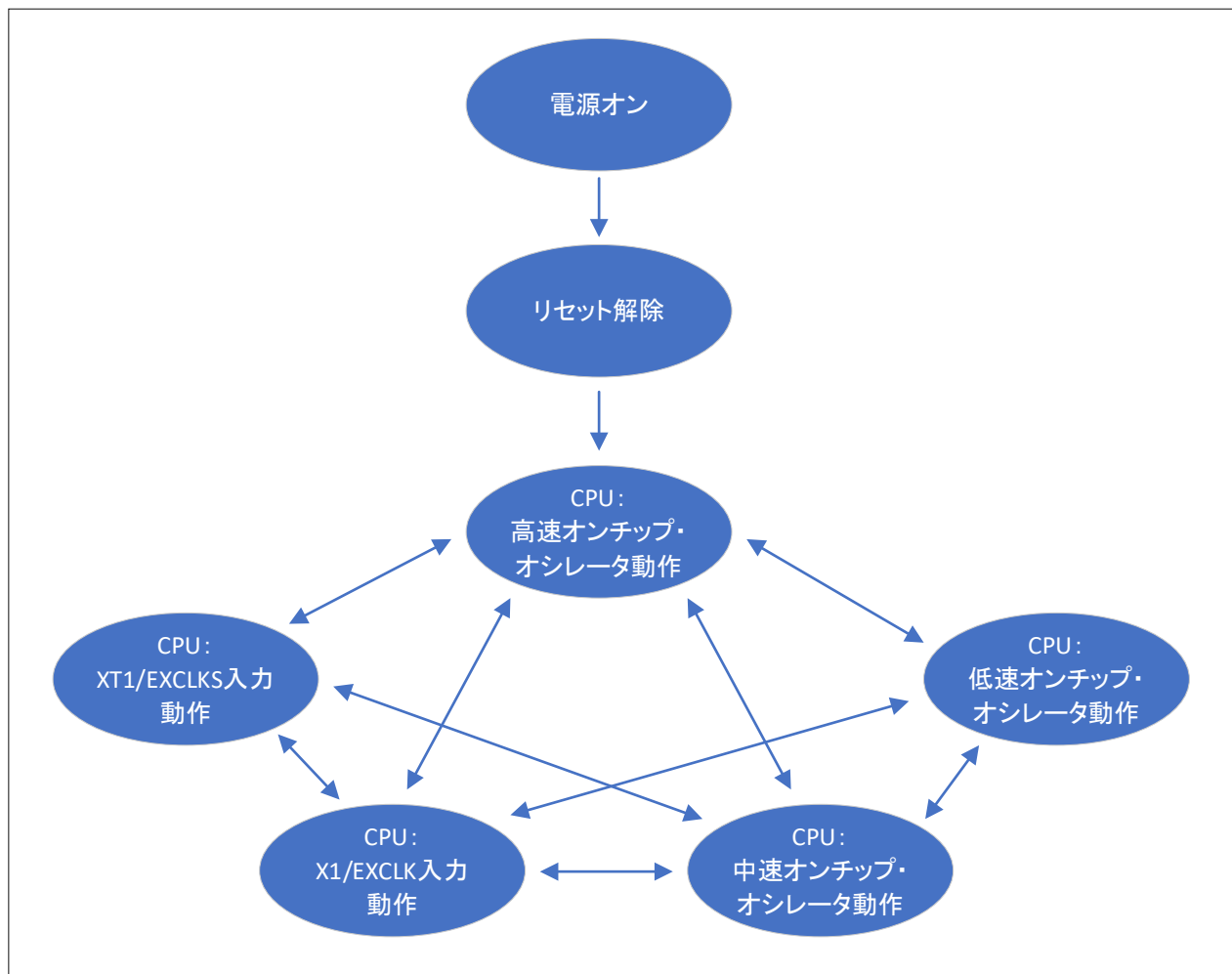
図 5-2 CPUクロック状態移行
