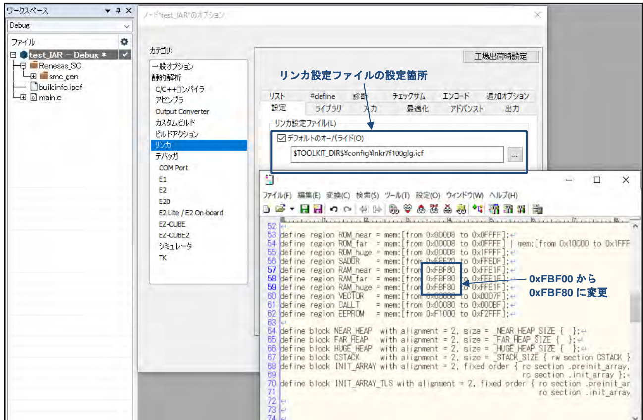
図 2-7 リンカ設定ファイル（R7F100GLG の場合）
