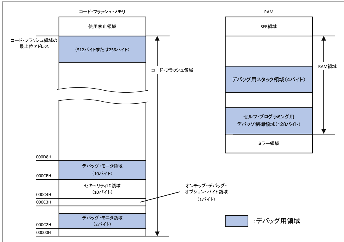
図 4-1 デバッグ用モニタ・プログラムが配置されるメモリ空間
