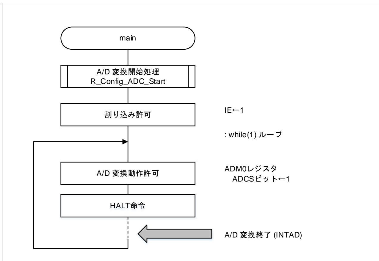
図 4-1 メイン処理
