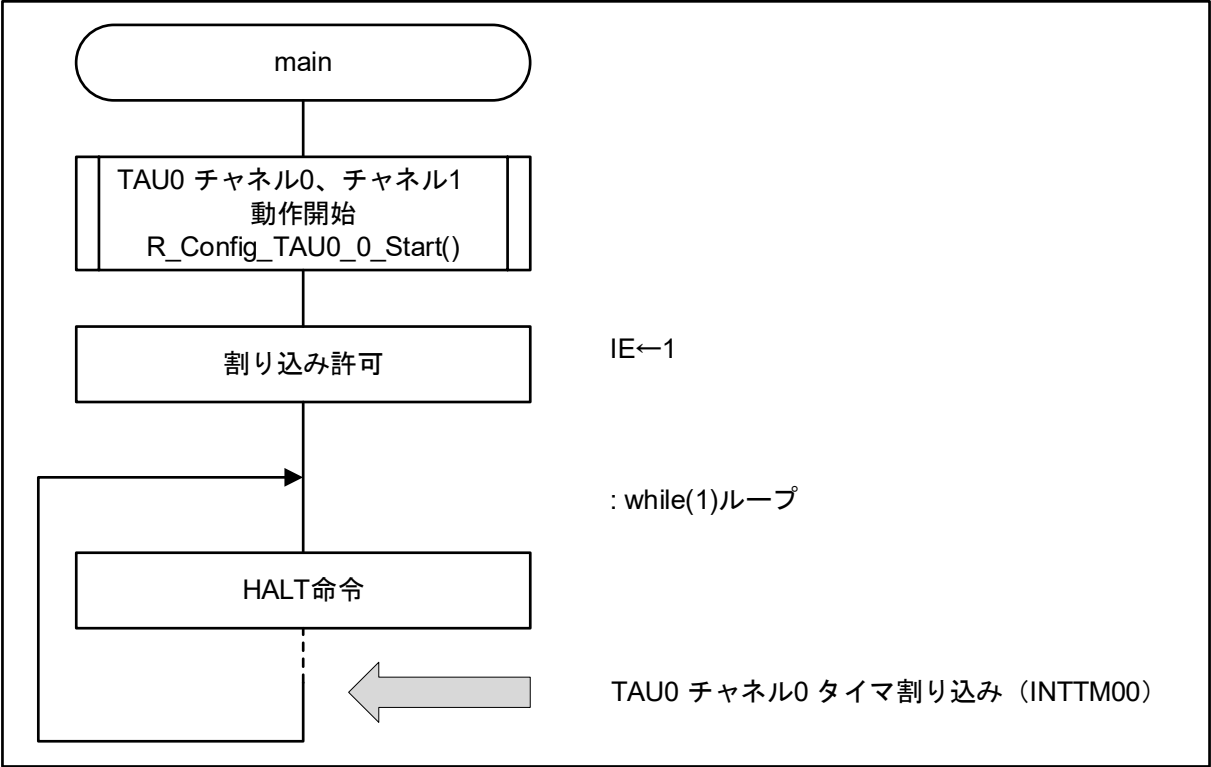
図 4-1 メイン処理
