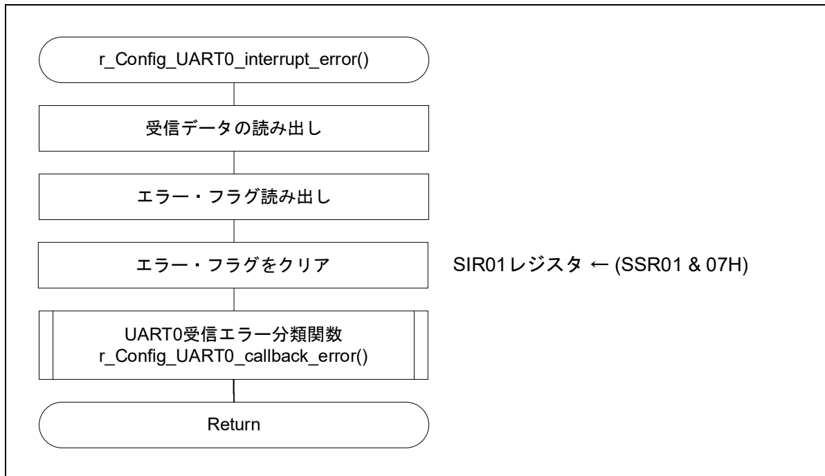
図 4-5 UART0 受信エラー割り込み処理関数
