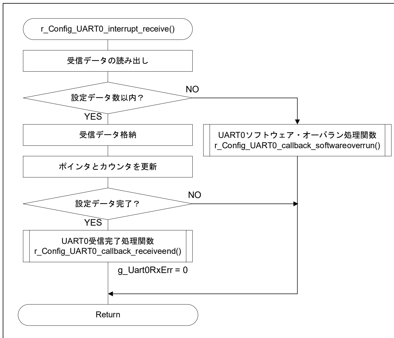
図 4-4 UART0 受信完了割り込み処理関数
