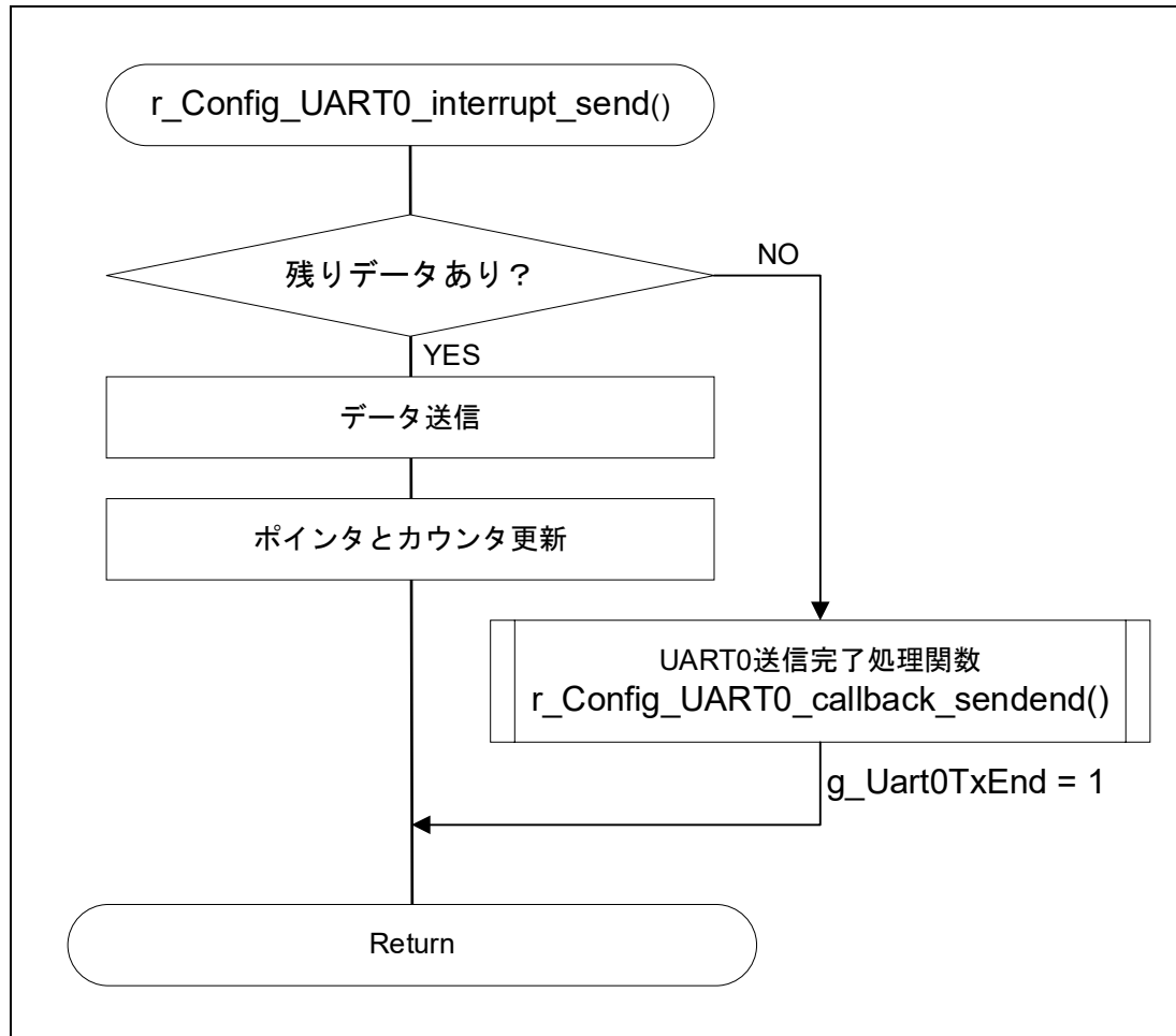
図 4-3 UART0 送信完了割り込み処理関数
