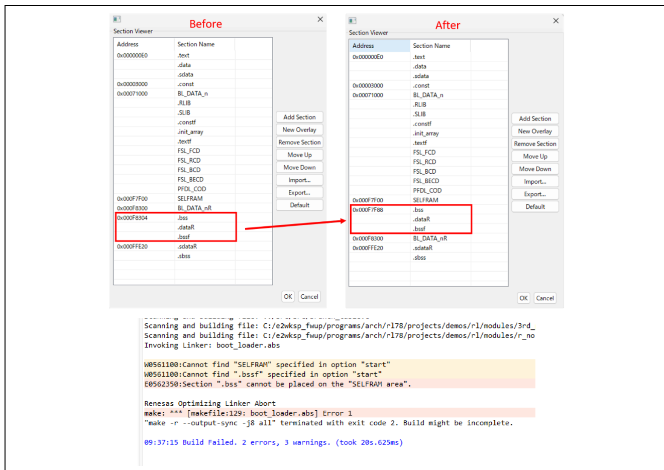
図 4-4 セクション定義とコード生成後のリンクエラー
