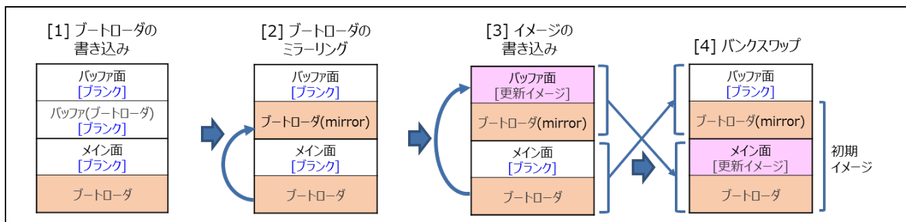
図 1-10 ブートローダを用いた初期状態の構築（デュアルバンク（2 バンク）方式の例）
