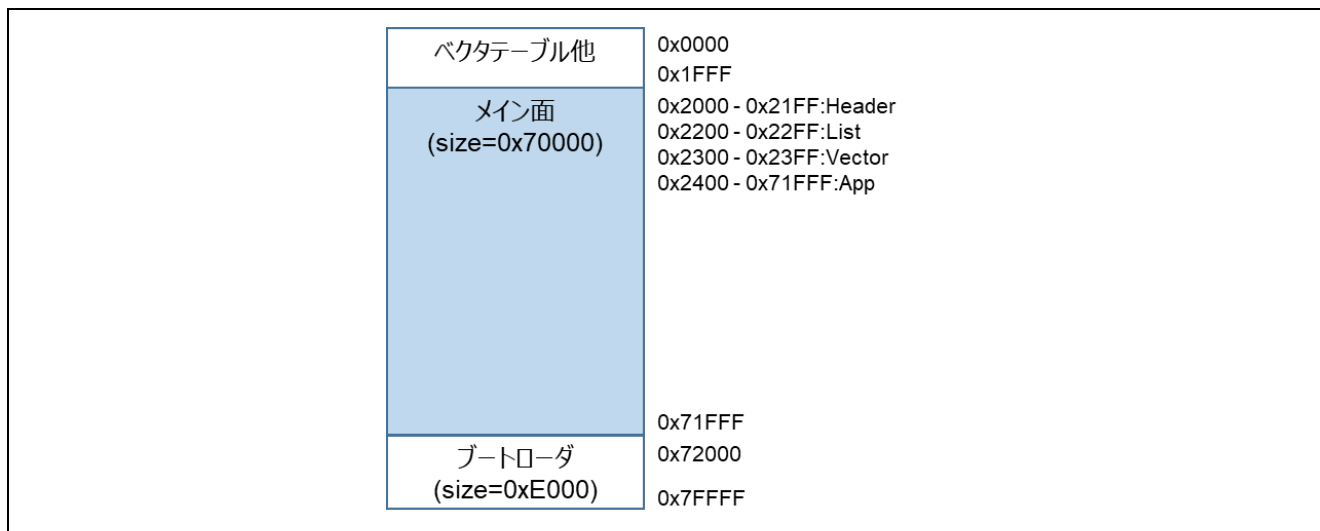
図 6-6 RL78/G13 の全面更新方式のデモプロジェクトのメモリマップ (LLVM の場合)
