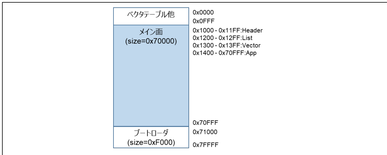
図 6-5 RL78/G13 の全面更新方式のデモプロジェクトのメモリマップ（CC-RL の場合）
