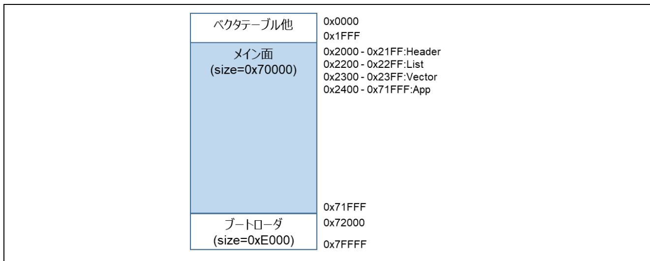
図 6-36 RL78/L23 の全面更新方式のデモプロジェクトのメモリマップ (LLVM の場合)
