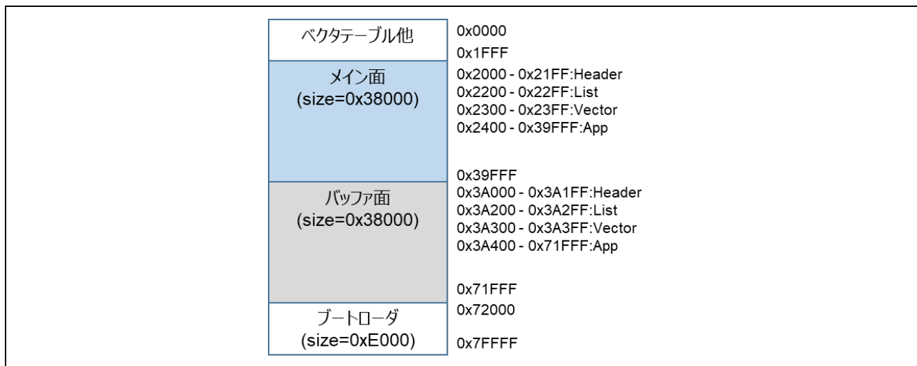
図 6-4 RL78/G13 の半面更新方式のデモプロジェクトのメモリマップ (LLVM の場合)
