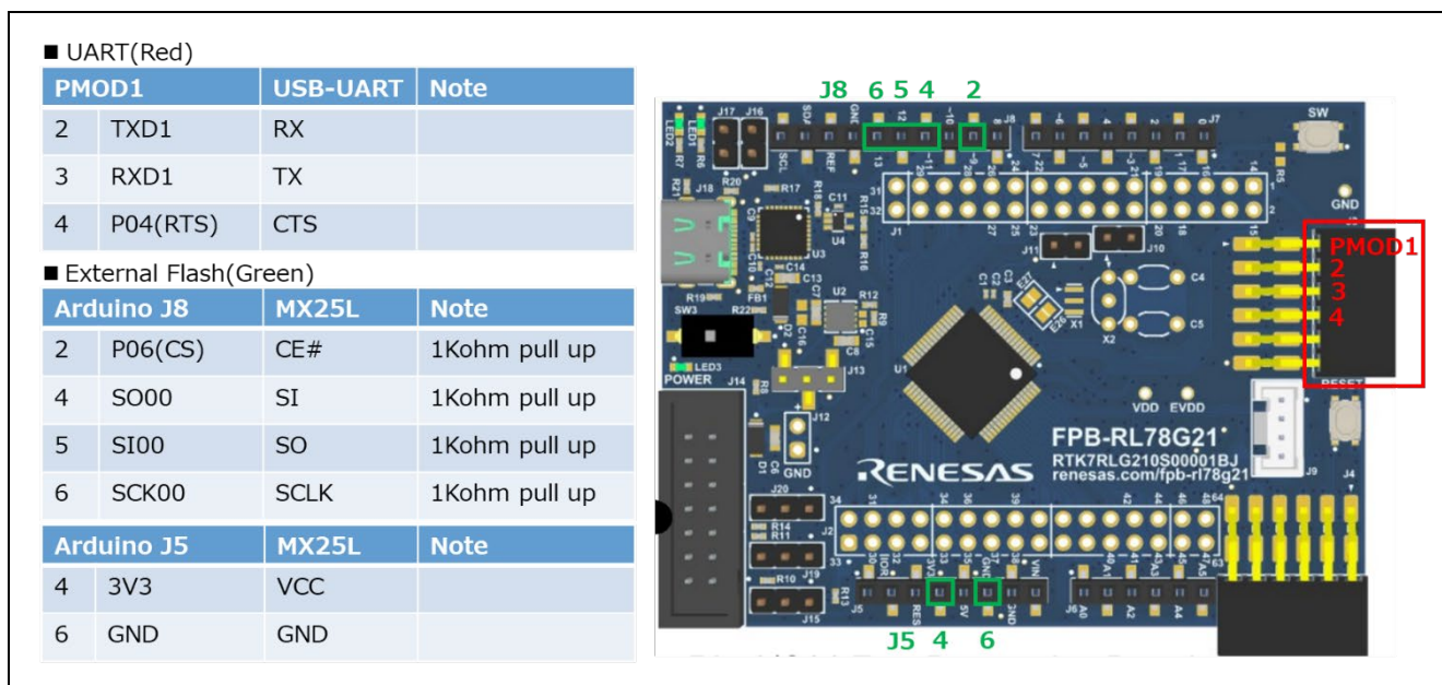
図 6-8 FPB-RL78G21 のピン情報
