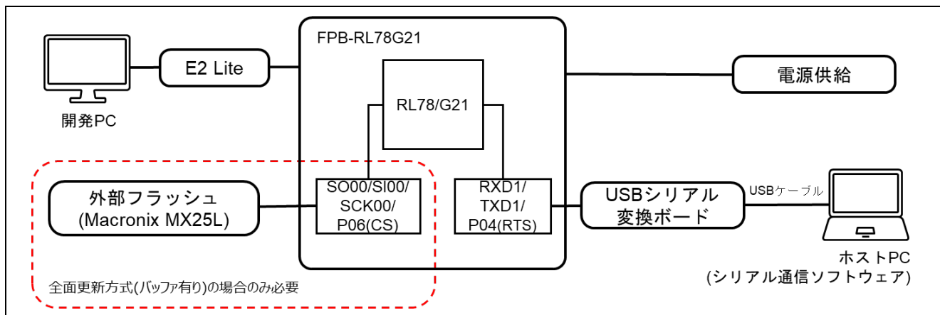
図 6-7 FPB-RL78G21 の機器接続図
