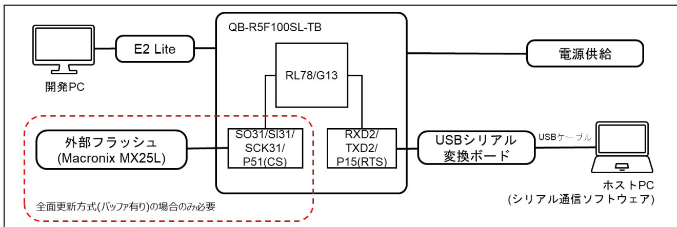
図 6-1 QB-R5F100SL-TB の機器接続図
