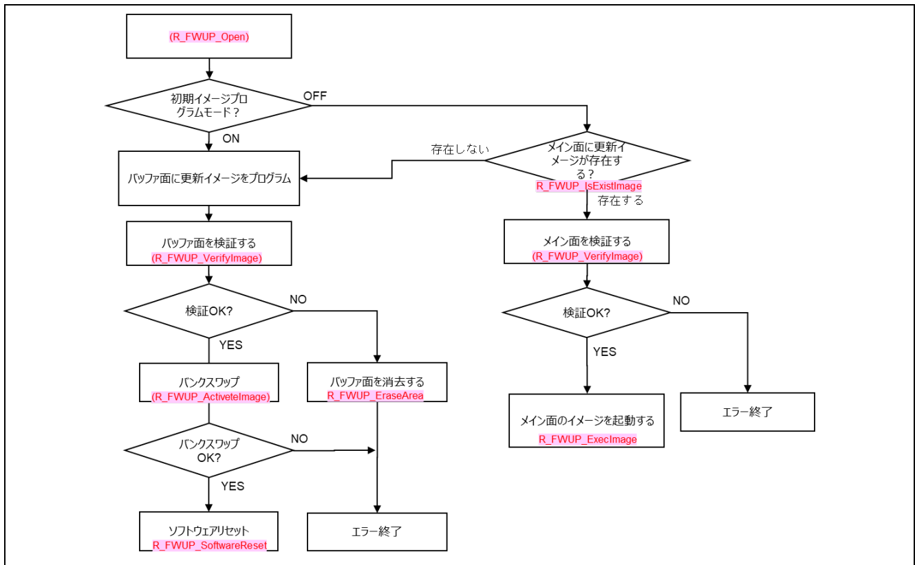
図 2-1 デュアルバンク（2 バンク）方式のブートローダの実装例
