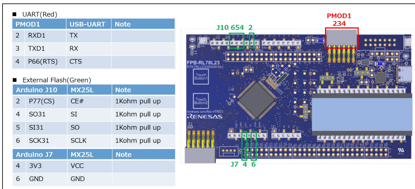
図 6-30 FPB-RL78L23 のピン情報
