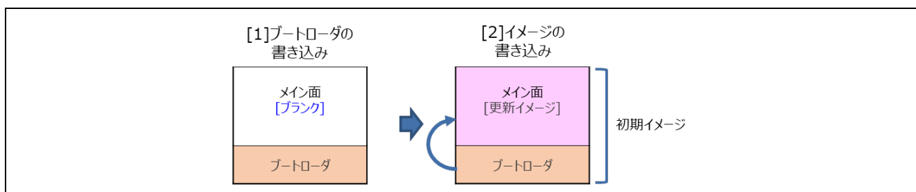
図 1-12 ブートローダを用いた初期状態の構築（全面更新方式）
