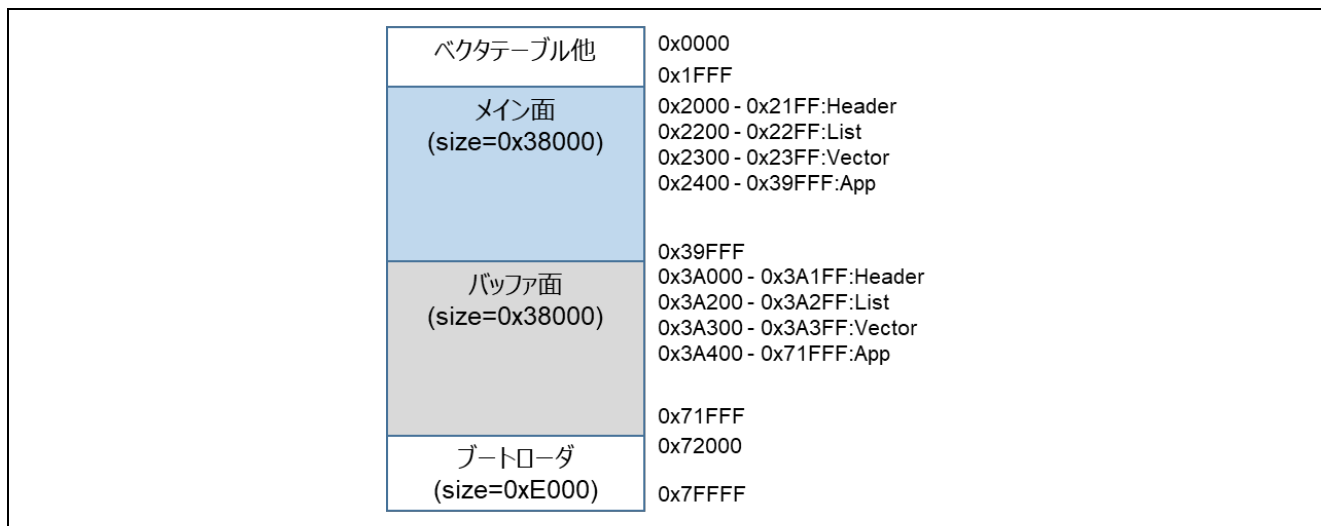
図 6-34 RL78/L23 の半面更新方式のデモプロジェクトのメモリマップ（LLVM の場合）
