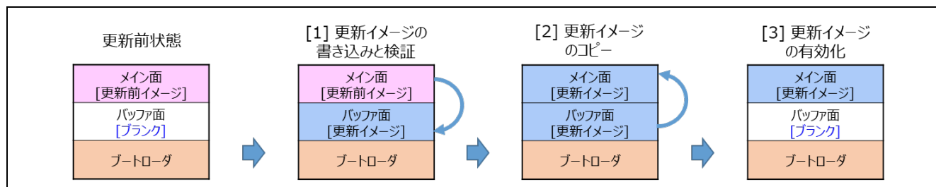
図 1-4 半面更新方式のアップデートの動作
