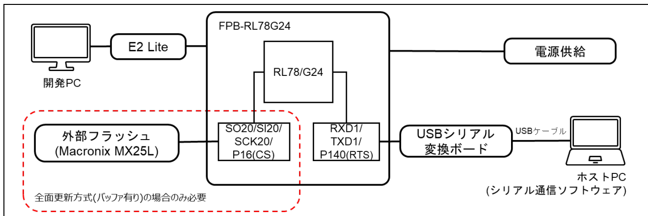
図 6-23 FPB-RL78G24 の機器接続図
