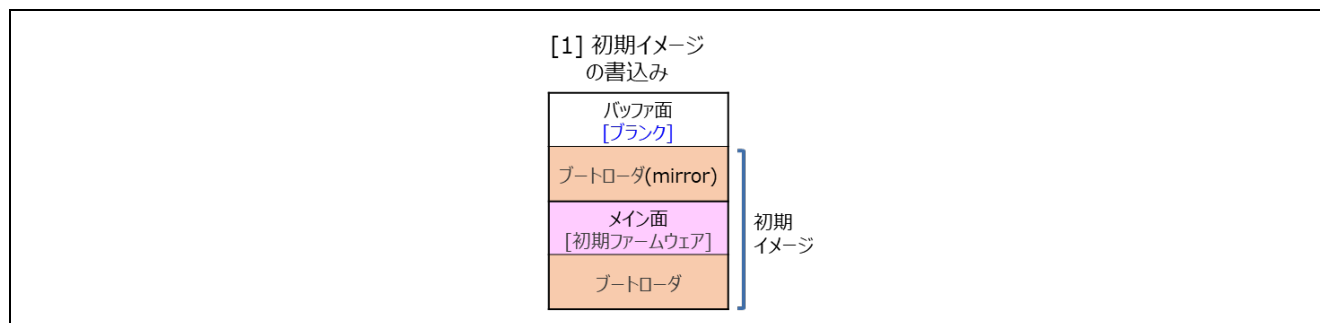
図 1-7 Renesas Image Generator を用いた初期状態の構築（デュアルバンク（2 バンク）方式の例）
