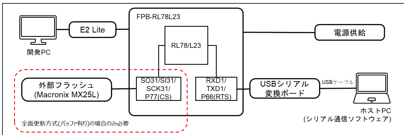
図 6-29 FPB-RL78L23 の機器接続図
