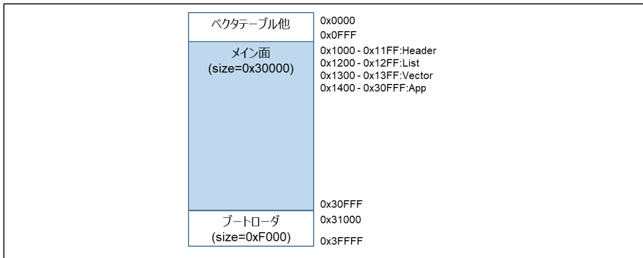
図 6-11 RL78/G21 の全面更新方式のデモプロジェクトのメモリマップ (CC-RL,IAR の場合)
