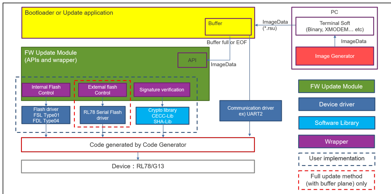
図 1-2 RL78/G13 向けファームウェアアップデートモジュールのモジュール構成
