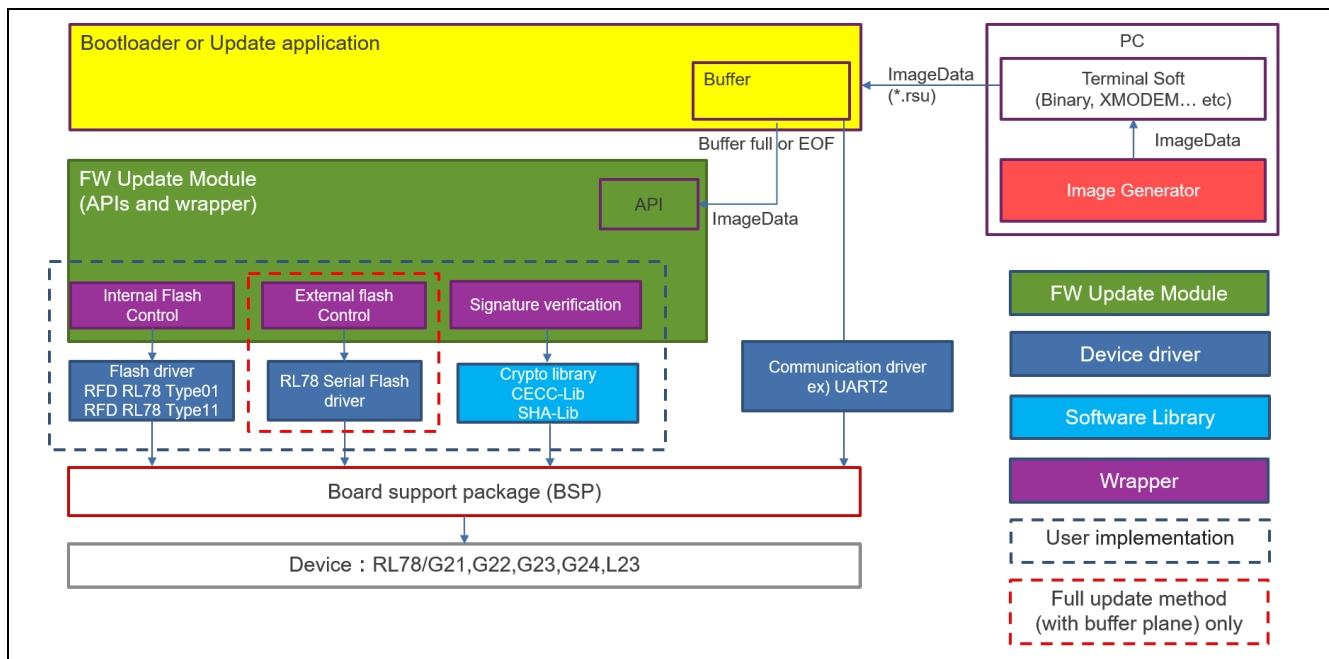
図 1-1 RL78/G21,G22,G23,G24,L23 向けファームウェアアップデートモジュールのモジュール構成
