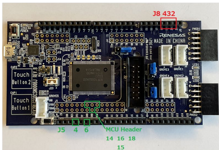
図 6-18 FPB-RL78G23-128p のピン情報
