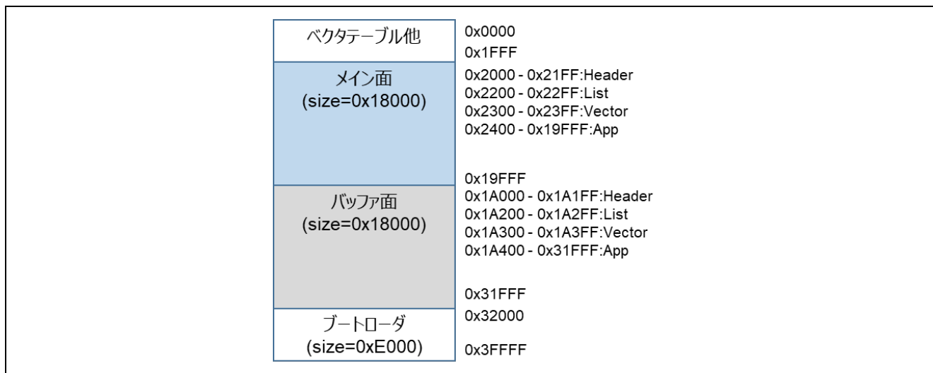
図 6-10 RL78/G21 の半面更新方式のデモプロジェクトのメモリマップ (LLVM の場合)
