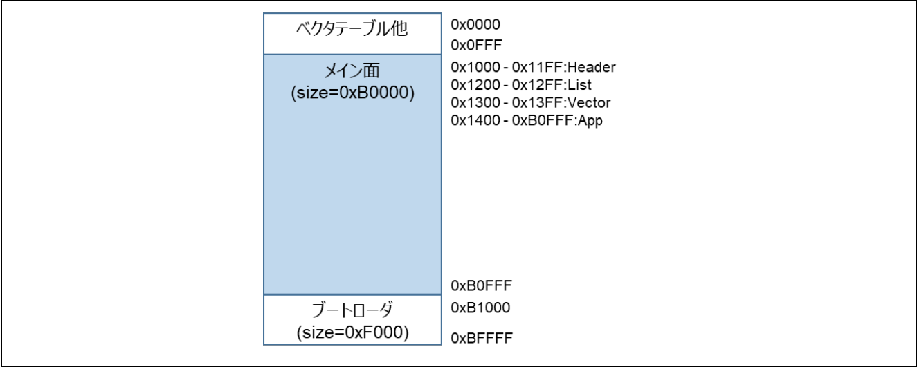
図 6-21 RL78/G23 の全面更新方式のデモプロジェクトのメモリマップ（CC-RL,IAR の場合）
