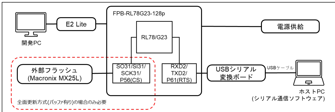
図 6-17 FPB-RL78G23-128p の機器接続図
