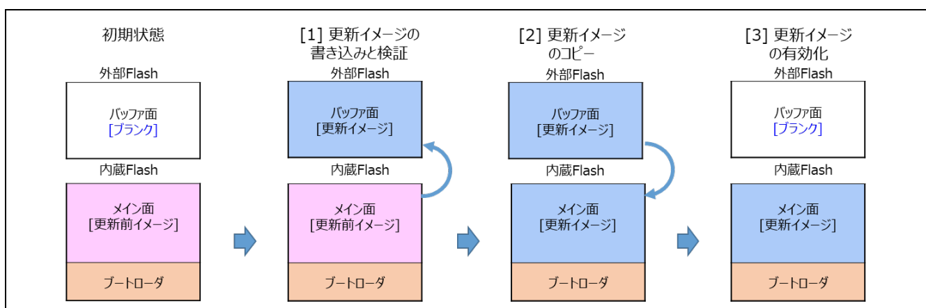
図 1-6 全面更新方式（バッファ有り）のファームウェアアップデートの動作
