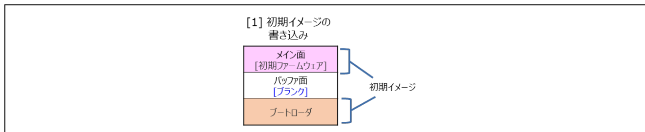
図 1-8 Renesas Image Generator を用いた初期状態の構築（半面更新方式の例）
