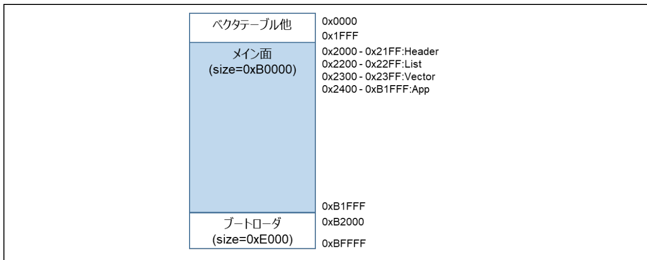
図 6-22 RL78/G23 の全面更新方式のデモプロジェクトのメモリマップ (LLVM の場合)
