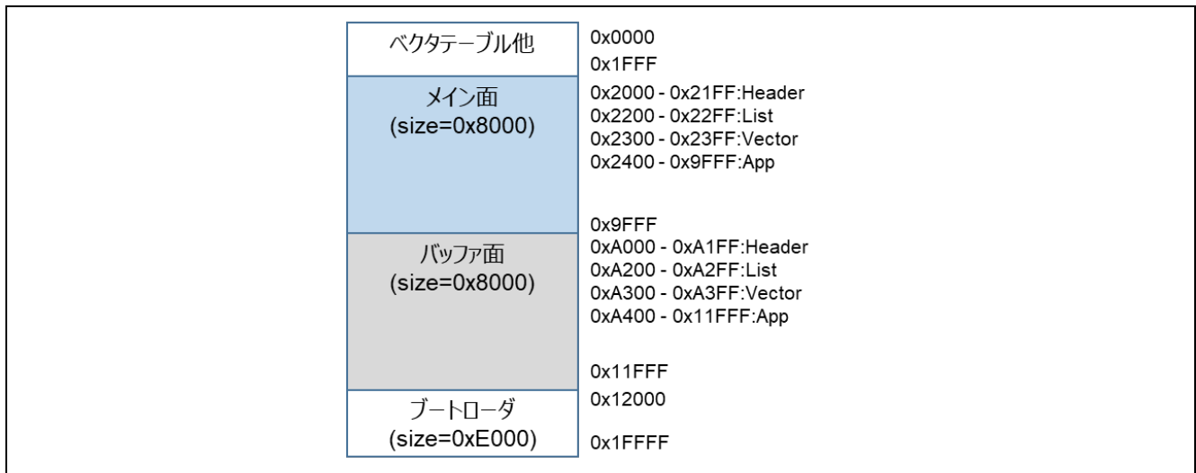
図 6-26 RL78/G24 の半面更新方式のデモプロジェクトのメモリマップ (LLVM の場合)
