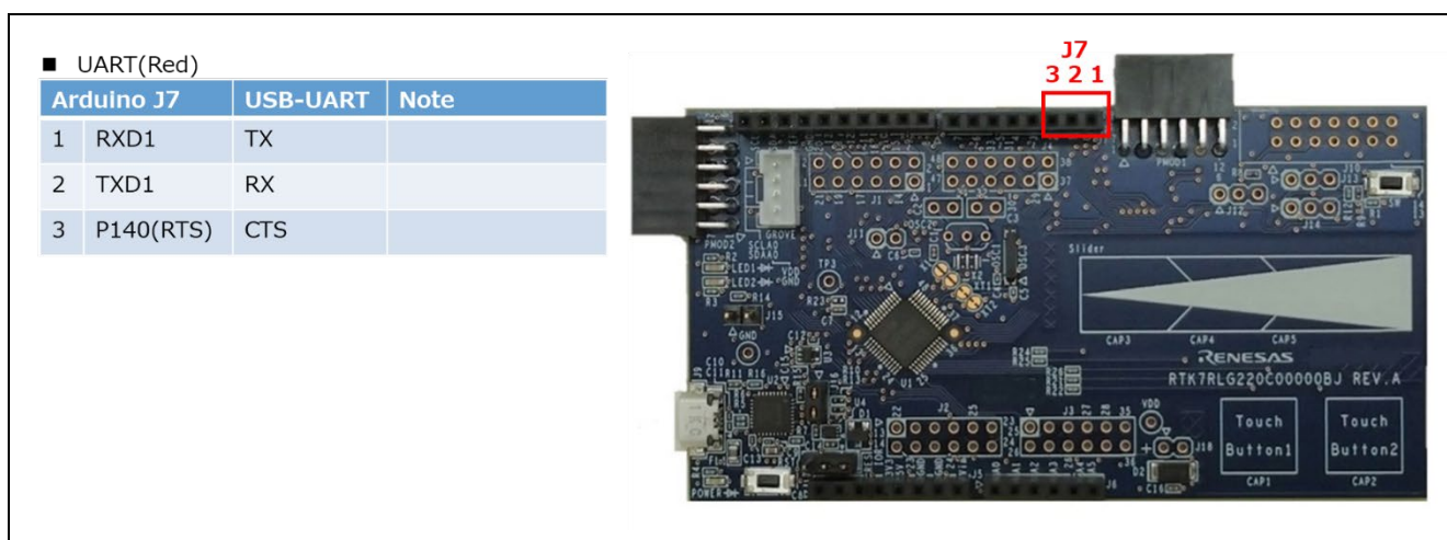
図 6-14 FPB-RL78G22 のピン情報
