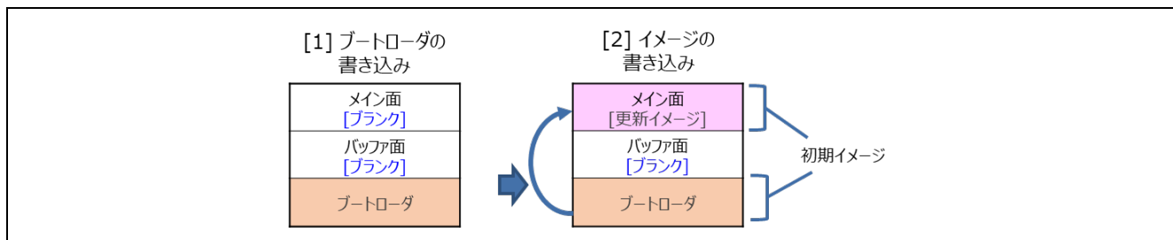
図 1-11 ブートローダを用いた初期状態の構築（半面更新方式）
