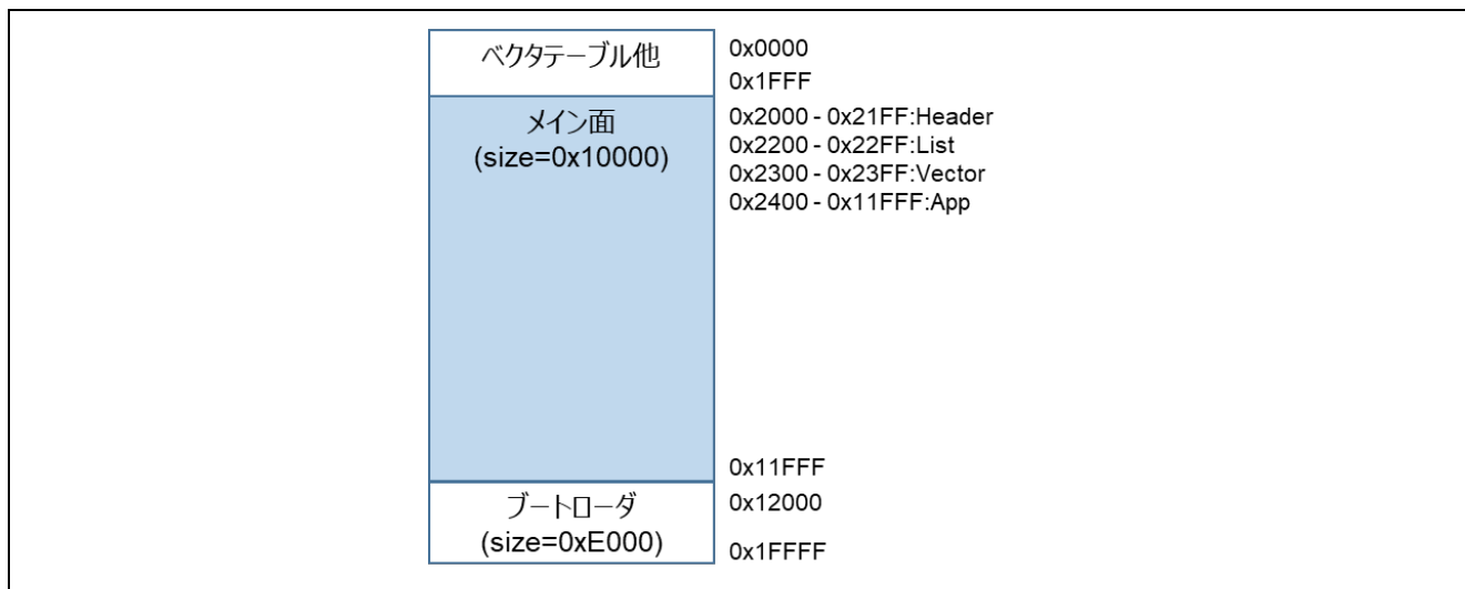
図 6-28 RL78/G24 の全面更新方式のデモプロジェクトのメモリマップ (LLVM の場合)
