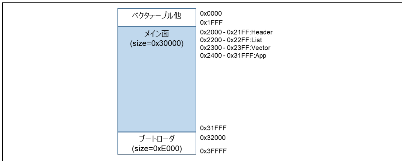
図 6-12 RL78/G21 の全面更新方式のデモプロジェクトのメモリマップ (LLVM の場合)
