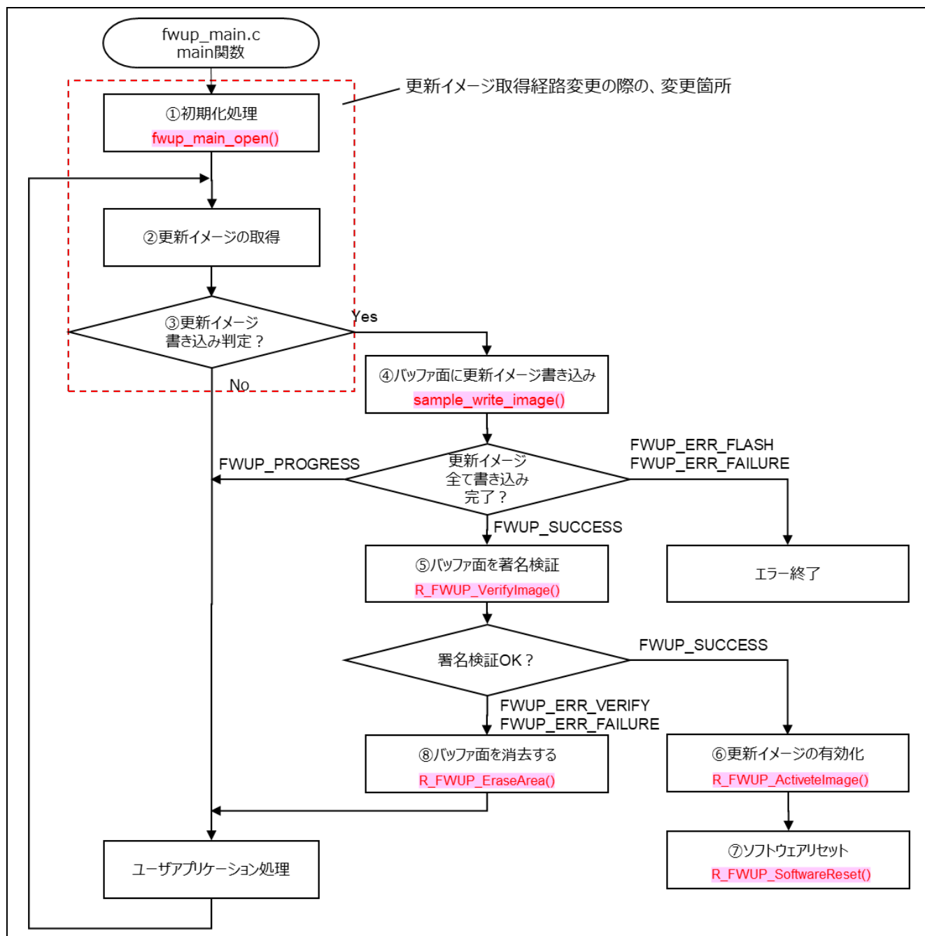
図 4-6 デモプロジェクトの fwup_main の処理フロー
