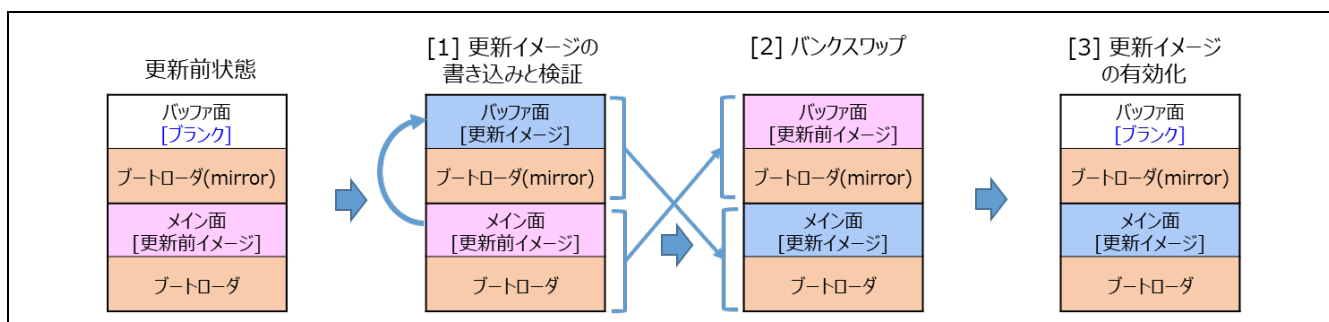
図 1-3 デュアルバンク（2 バンク）方式のアップデートの動作
