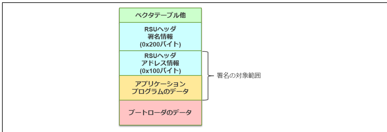
図 5-3 半面／全面更新方式の初期イメージファイルの構成
