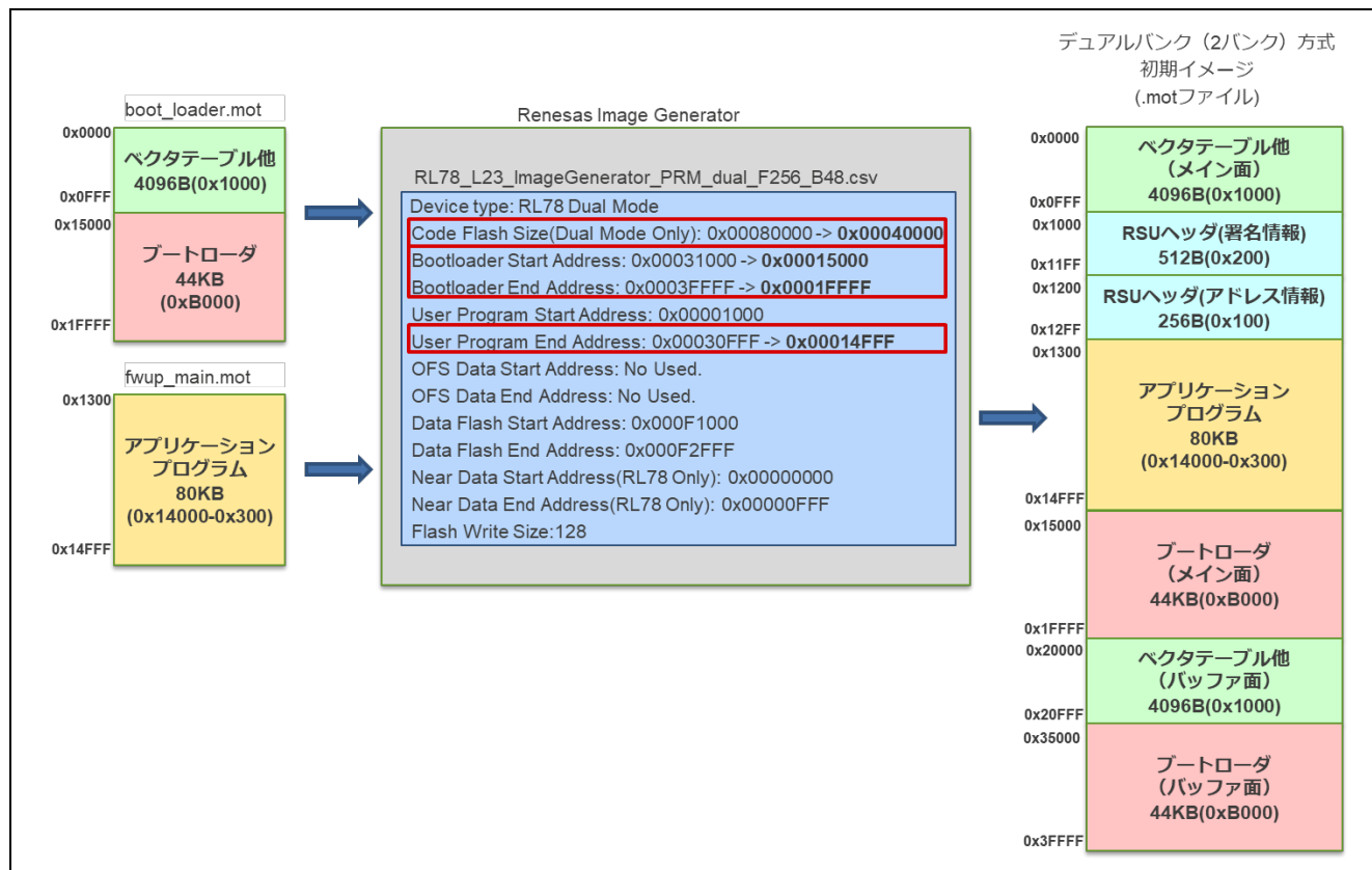
図 4-11 RL78/L23 (コードフラッシュ:256KB,ブートローダ:48KB) のデュアルバンク (2 バンク) 方式のパラメータファイル変更例
