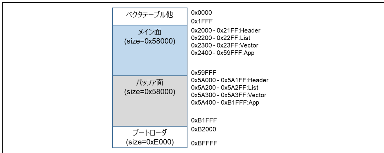
図 6-20 RL78/G23 の半面更新方式のデモプロジェクトのメモリマップ (LLVM の場合)
