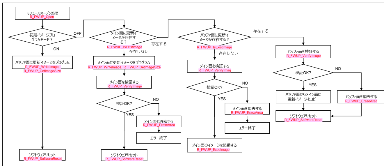
図 2-3 半面/全面更新方式（バッファ有り）のブートローダ実装例
