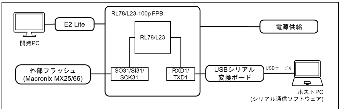
図 6-17 RL78/L23-100p FPB 全面更新方式（バッファ面は外部フラッシュ）の機器接続図
