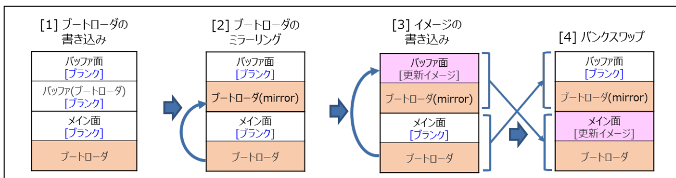
図 1-9 ブートローダを用いた初期状態の構築（デュアルバンク（2 バンク）方式の例）
