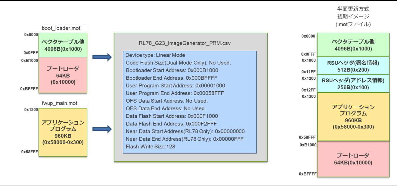
図 5-8 RL78/G23 の半面更新方式の初期イメージ生成を行う際に参照するパラメータ例
