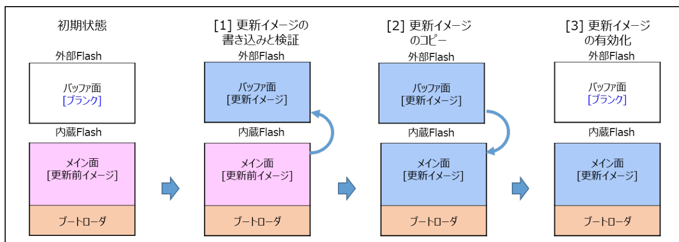
図 1-5 全面更新方式（バッファ面は外部フラッシュ）のファームウェアアップデートの動作
