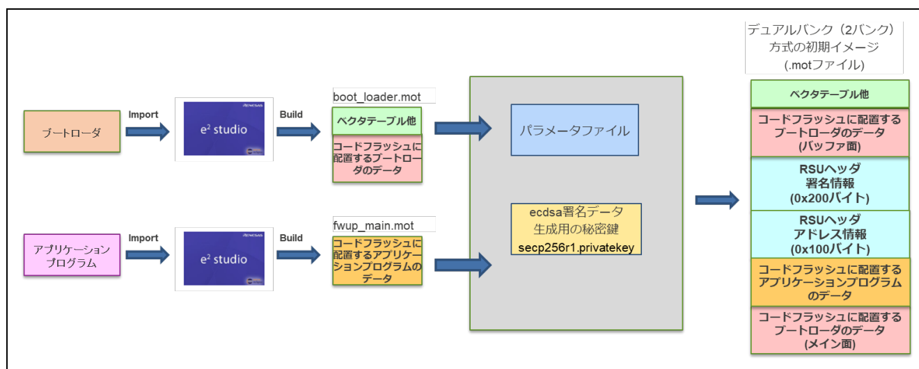
図 5-6 デュアルバンク（2 バンク）方式の初期イメージ
