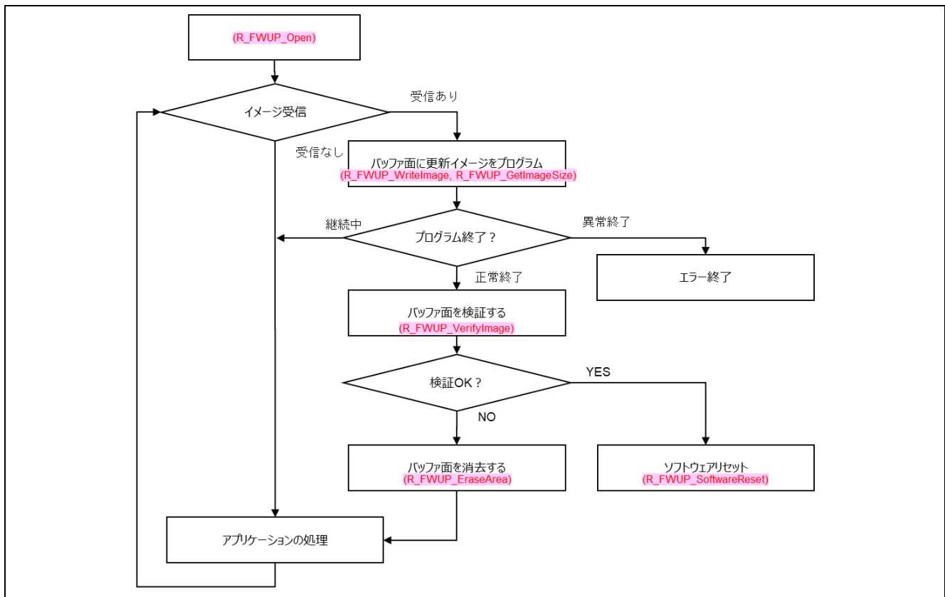
図 2-4 半面/全面更新方式（バッファ有り）のアプリケーションプログラム実装例
