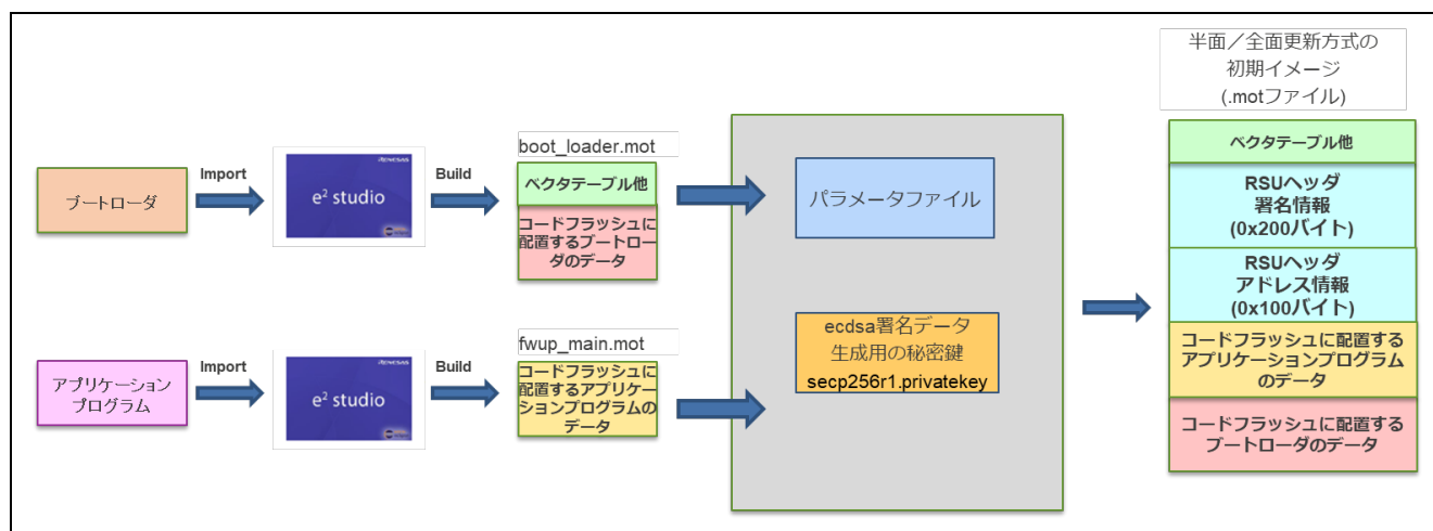
図 5-5 半面更新方式および全面更新方式の初期イメージ
