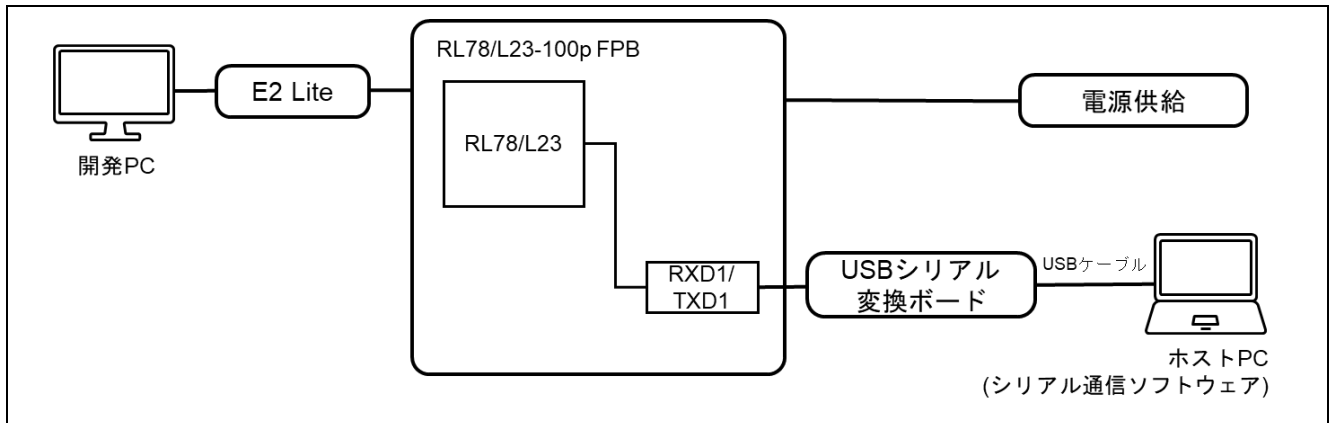
図 6-16 RL78/L23-100p FPB デュアルバンク（2 バンク）方式/半面更新方式の機器接続図
