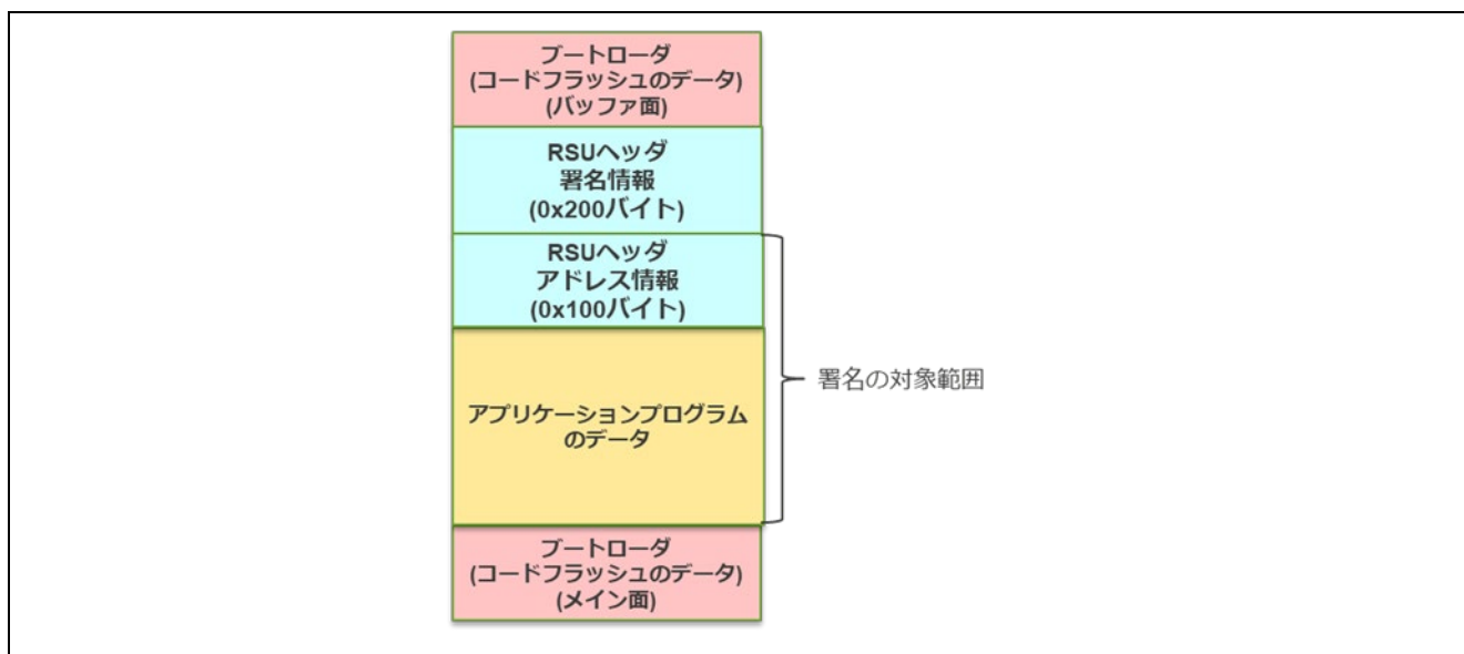
図 5-4 初期イメージファイル（デュアルバンク（2 バンク）方式）の構成
