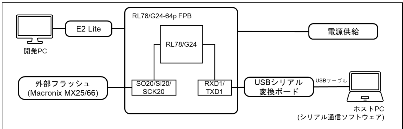
図 6-9 RL78/G24-64p FPB 全面更新方式（バッファ面は外部フラッシュ）の機器接続図
