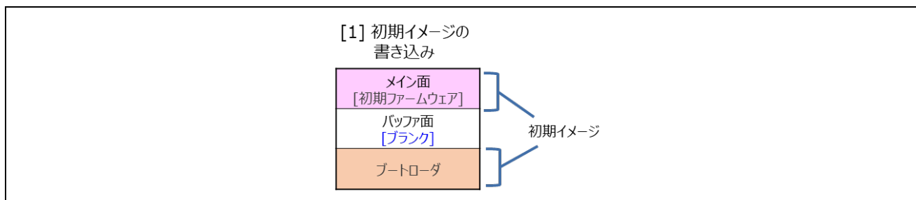
図 1-7 Renesas Image Generator を用いた初期状態の構築（半面更新方式の例）
