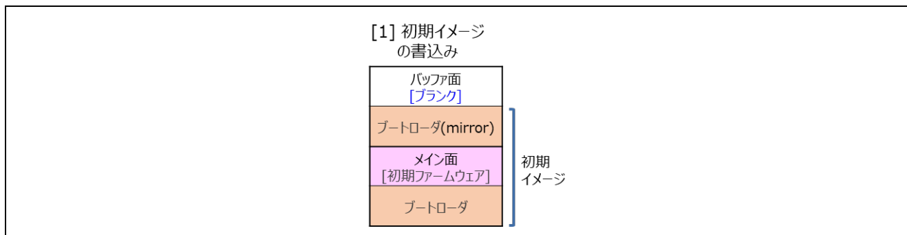
図 1-6 Renesas Image Generator を用いた初期状態の構築（デュアルバンク（2 バンク）方式の例）
