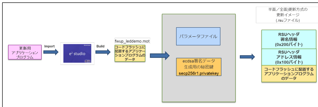
図 5-2 デュアルバンク(2 バンク)方式/半面更新方式/全面更新方式の更新イメージ
