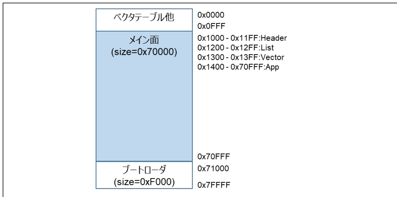
図 6-21 RL78/L23 の全面更新方式（バッファ面は外部フラッシュ）のデモプロジェクトのメモリマップ
