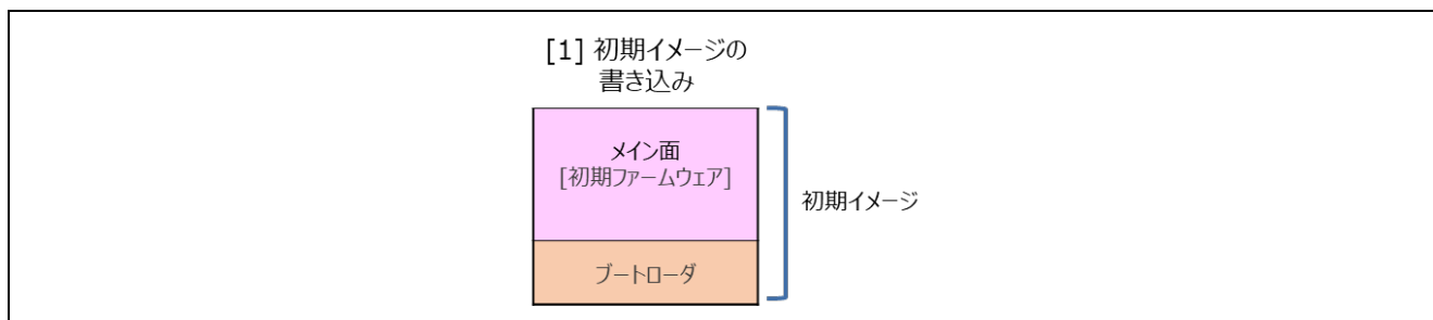
図 1-8 Renesas Image Generator を用いた初期状態の構築（全面更新方式の例）
