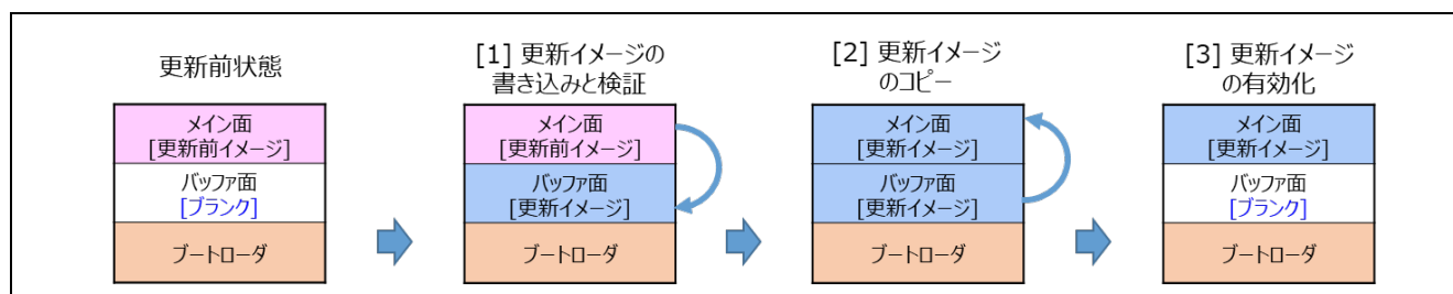
図 1-3 半面更新方式（バッファ面は内部フラッシュ）のアップデートの動作
