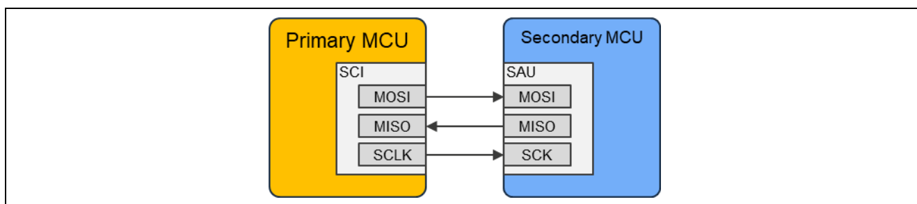
図 1-2 ハードウェア構成(SPI)
