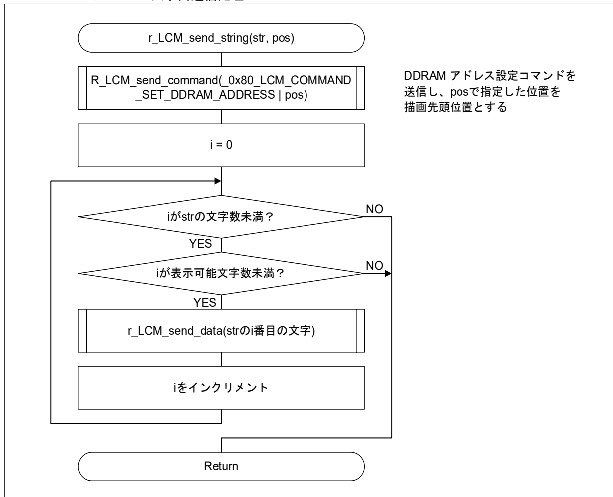
図 4-18 LCD モジュール 文字列送信処理
