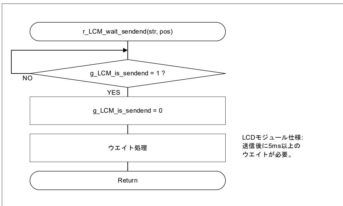
図 4-22 LCD モジュール 通信終了待ち処理
