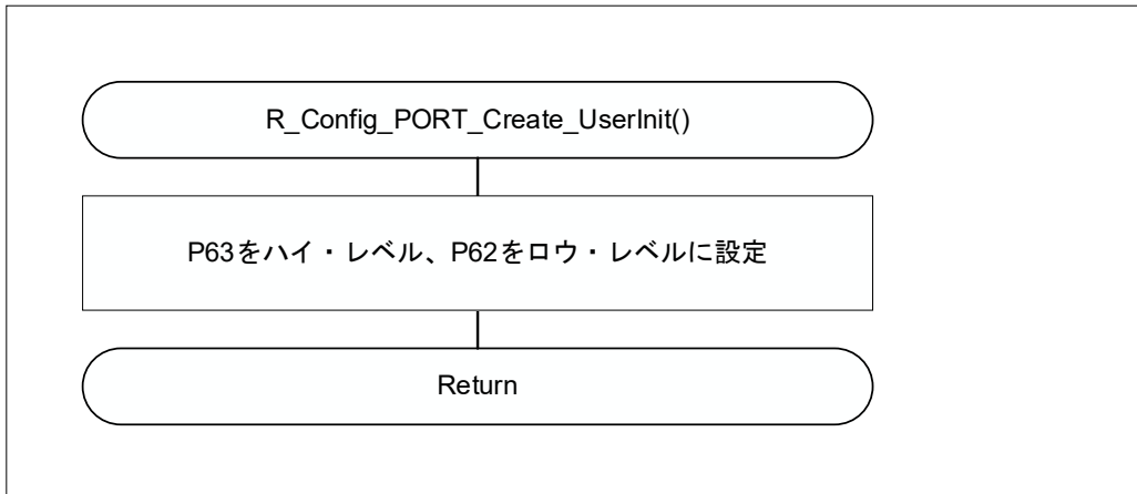
図 4-15 ポート初期化処理 (ユーザ定義箇所)
