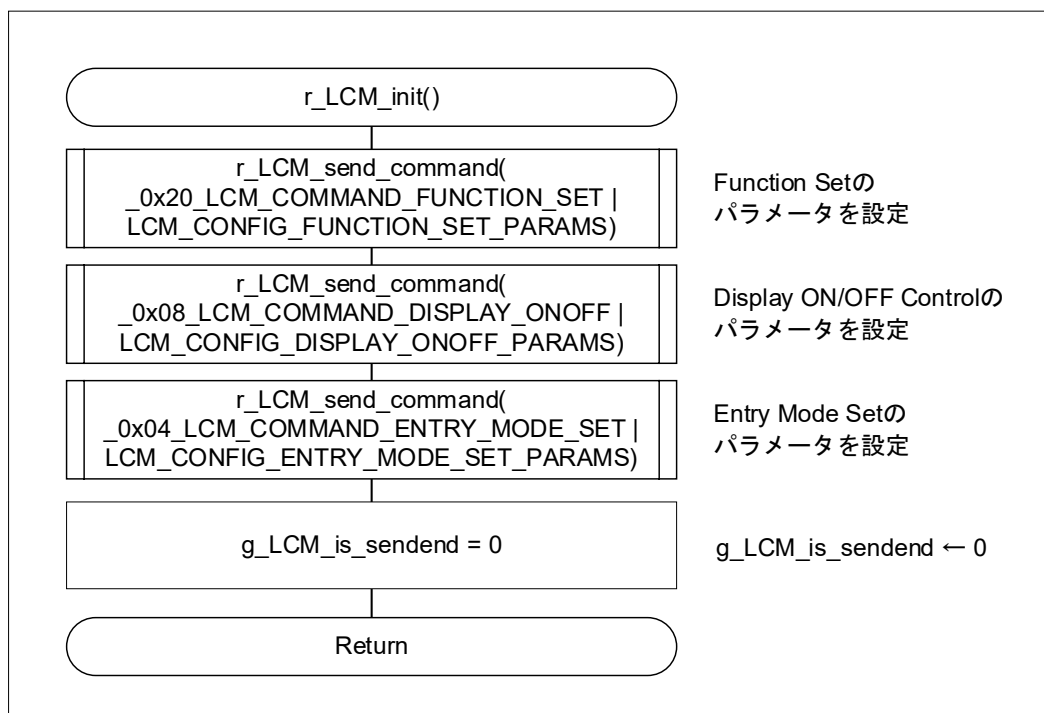
図 4-16 LCD モジュール初期化
