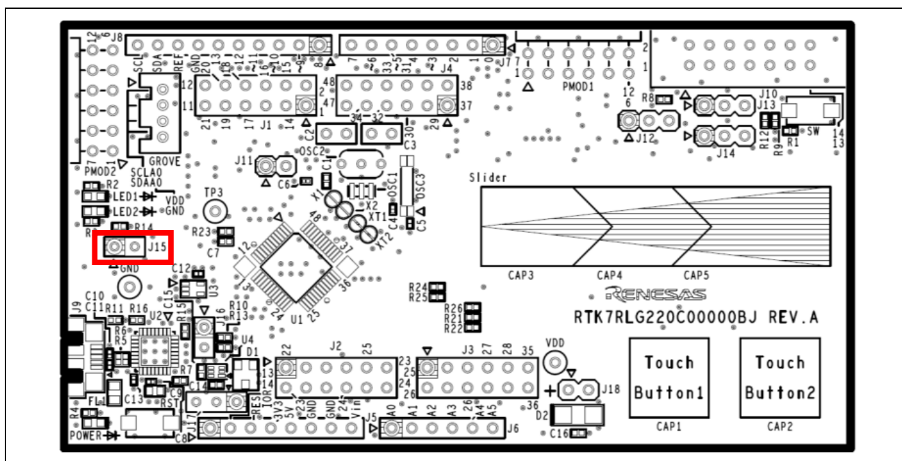
図 6-11 USB-シリアル変換器リセットヘッダ(J15)の位置
