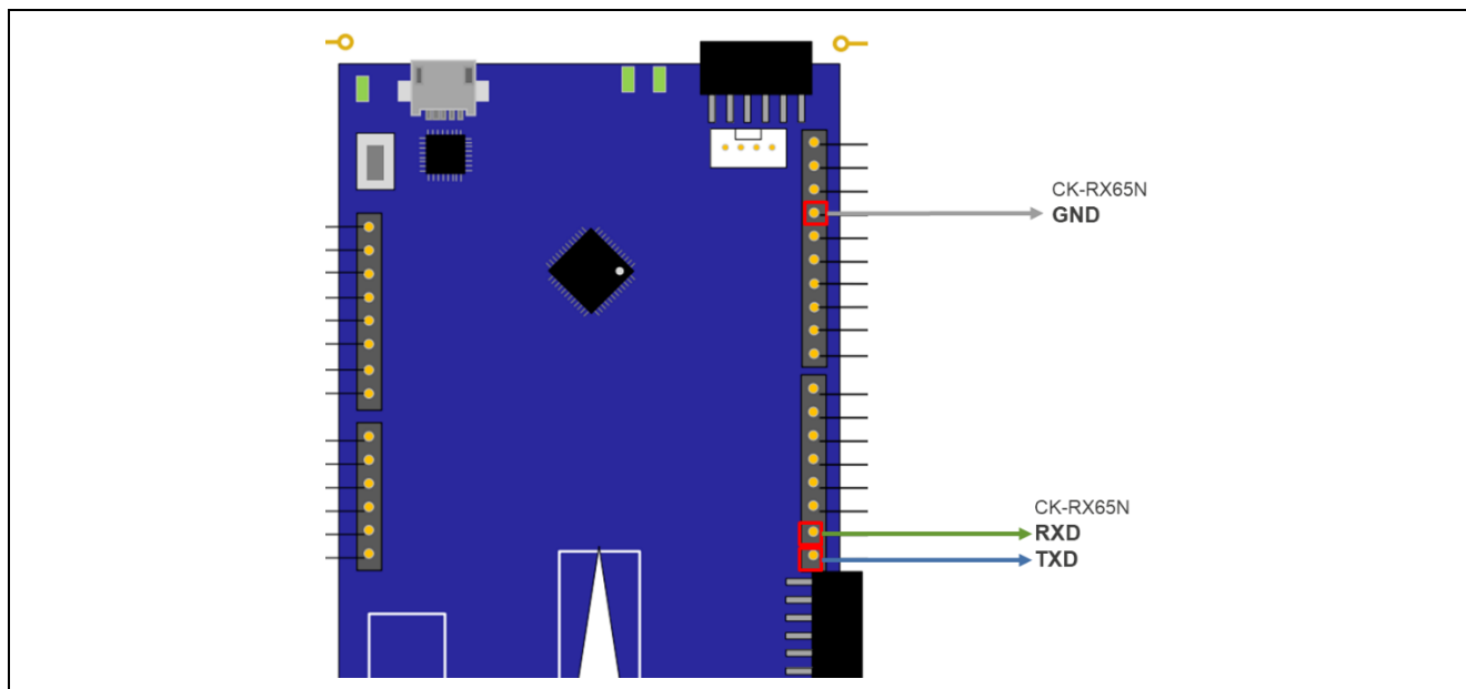
図 6-8 RL78/G22 FPD のマイコン間 UART 通信に使用する端子位置
