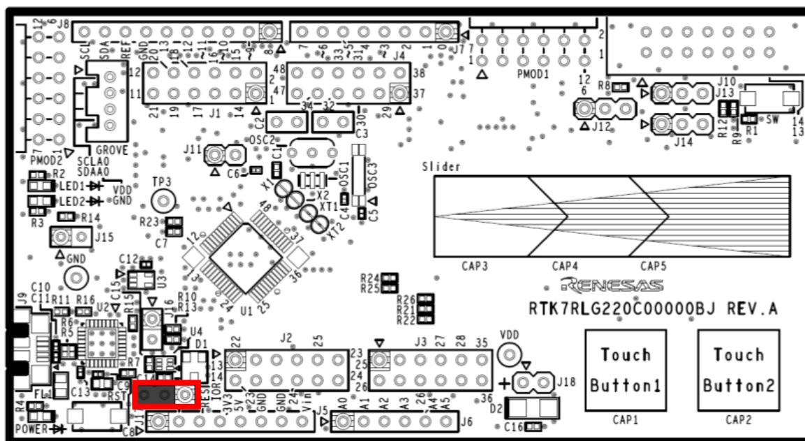
図 6-7 電源選択ヘッダ(J17)の位置
