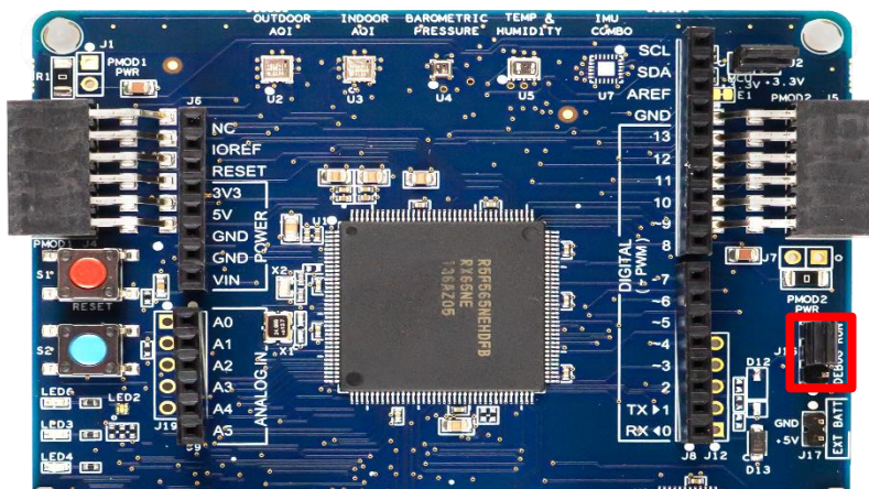
図 6-6 ジャンパ J16 の位置
