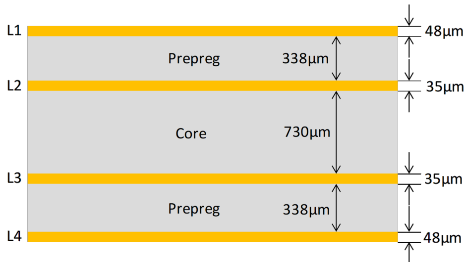
図 2 基板層構成
